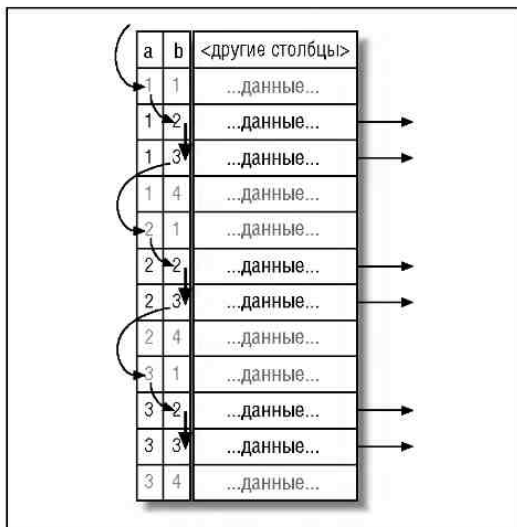
Рис. 4.6. Непоследовательный просмотр индекса, который в MySQL пока не реализован, позволил бы выполнить запрос более эффективно
