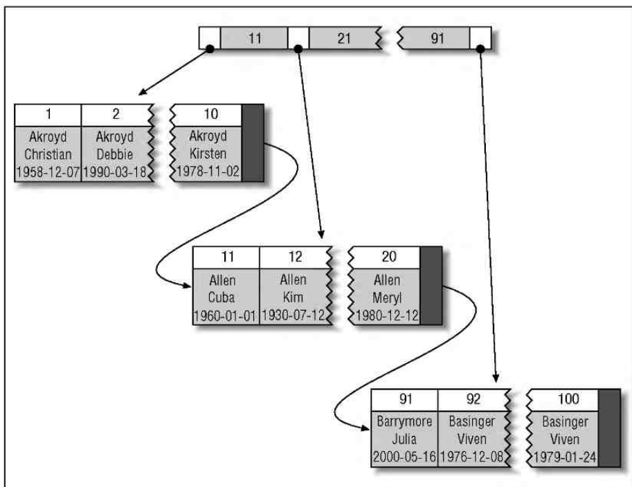
Рис. 3.3. Расположение записей в кластерном индексе
