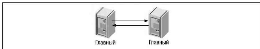
Рис. 8.5. Репликация главный–главный
