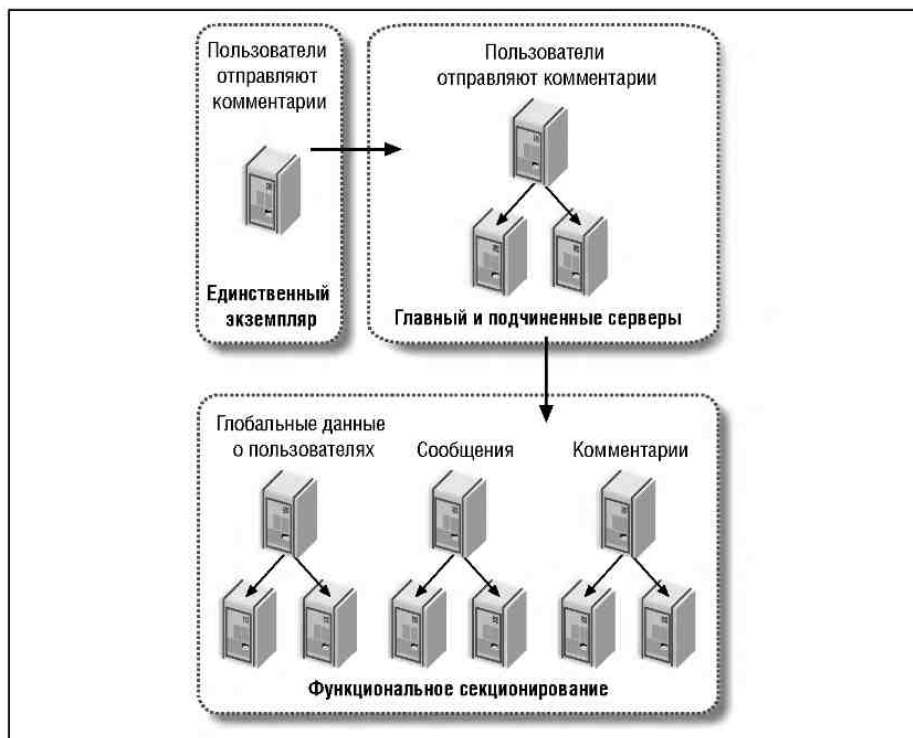
Рис. 9.2. От одного экземпляра к функционально секционированному хранилищу данных
