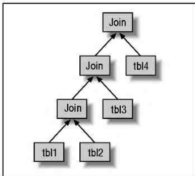
Рис. 4.4. Как соединяются несколько таблиц в MySQL
