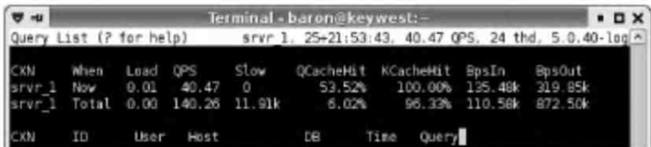
Рис. 14.3. innotop в режиме Q (Query List)
