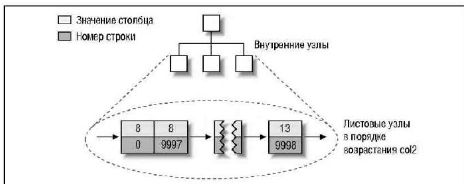
Рис. 3.6. Размещение индекса по столбцу col2 для таблицы layout_test в MyISAM
