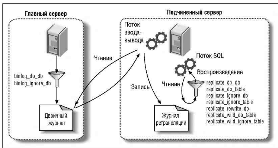
Рис. 8.3. Фильтры репликации
