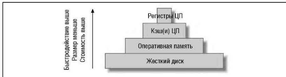
Рис. 7.1. Иерархия кэшей
