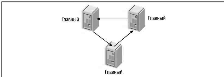
Рис. 8.9. Топология репликации «кольцо»
