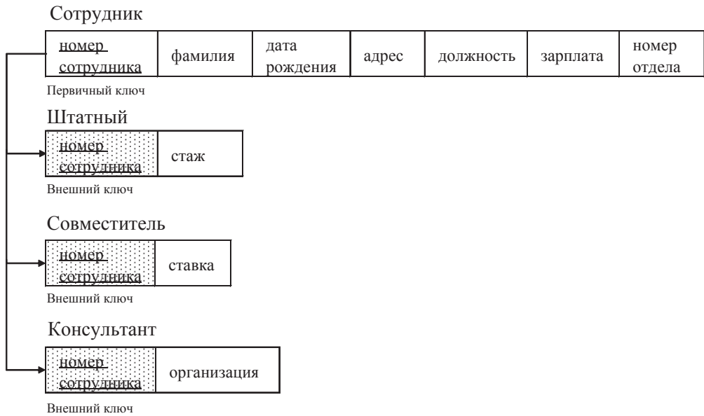
Рис. 3. Категориальная связь
