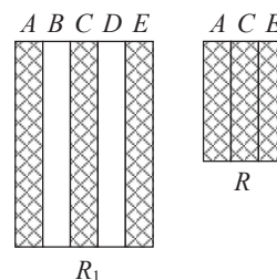
Рис. 8. Операция проекции
