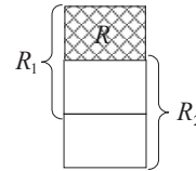
Диаграмма Венна
