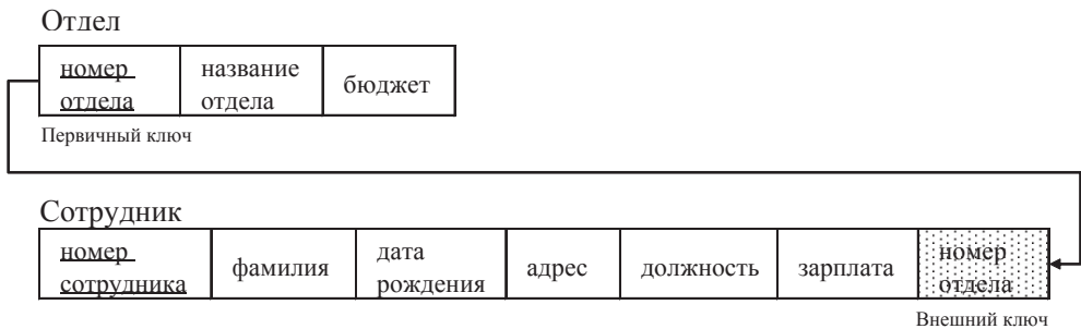
Рис. 1. Неидентифицирующая связь
