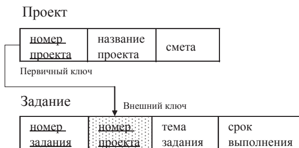
Рис. 2. Идентифицирующая связь
