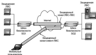
Рис. 10.4. Виртуальные защищенные каналы типа ЛВС–ЛВС и клиент–ЛВС
