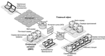
Рис. 13.1. Схема защиты корпоративной сети от воздействия вредоносных программ и вирусов
