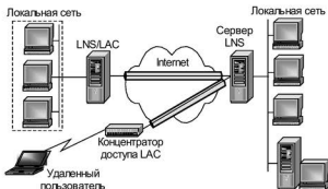
Рис. 8.9. Схемы туннелирования по протоколу L2TP
