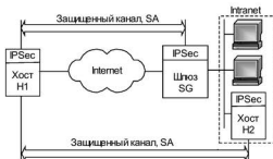
Рис. 8.19. Схема хост-шлюз, дополненная каналом хост-хост
