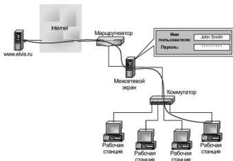
Рис. 9.3. Схема аутентификации пользователя по предъявляемому паролю
