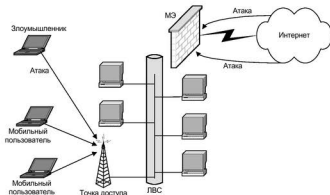
Рис. 1.1. Угрозы при беспроводном доступе к локальной сети
