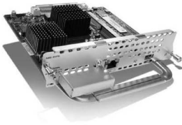
Рис. 10.9. Модуль NME-RVPN
