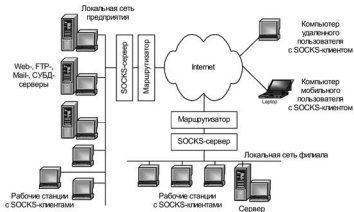
Рис. 8.22. Схема взаимодействия по протоколу SOCKS
