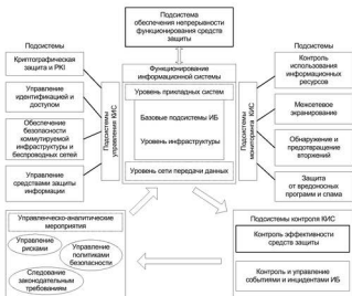
Рис. 6.7. Общая структура многоуровневой комплексной системы защиты информации КИС
