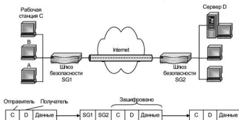
Рис. 10.3. Схема виртуального защищенного туннеля
