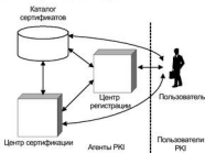
Рис. 4.29. Структура PKI
