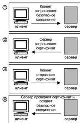
Рис. 8.21. Процесс аутентификации клиента сервером
