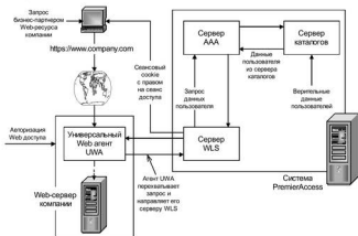
Рис. 11.3. Схема управления веб-доступом
