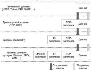
Рис. 8.3. Схема инкапсуляции данных в стеке протоколов TCP/IP
