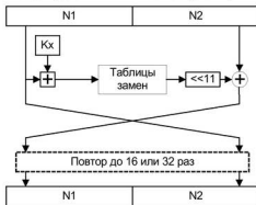
Рис. 4.7. Схема алгоритма ГОСТ 28147-89
