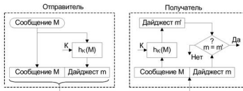
Рис. 5.7. Применение для аутентификации односторонней хэш-функции с параметром-ключом
