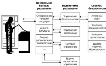
Рис. 14.5. Интеграция сервисов безопасности и системы управления
