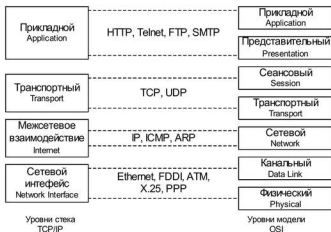
Рис. 8.1. Уровни стека протоколов TCP/IP
