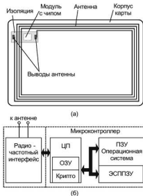
Рис. 5.5. Микропроцессорная смарт-карта с бесконтактным интерфейсом:
