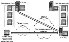
Рис. 8.20. Криптозащищенные туннели, сформированные на основе протокола SSL
