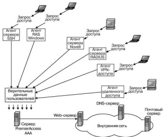
Рис. 11.2. Схема управления доступом к сети
