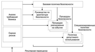
Рис. 2.2. Схема разработки политики безопасности
