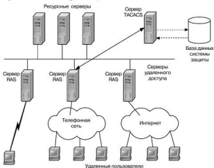
Рис. 11.7. Схема централизованного контроля удаленного доступа
