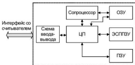
Рис. 5.3. Блок-схема микроконтроллера, встраиваемого в микропроцессорную смарт-карту
