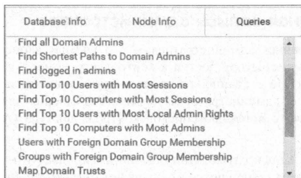
Рис. 1.5. Запросы BloodHound
