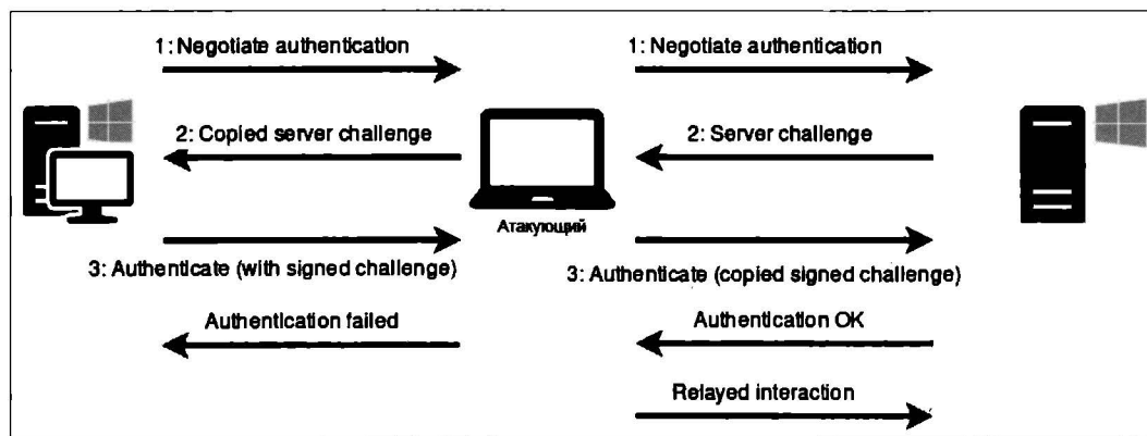
Рис. 2.20. Схема relay-атаки
