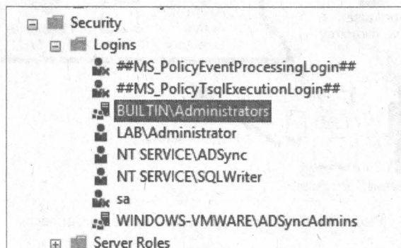
Рис. 1.14. Конфигурации безопасности
