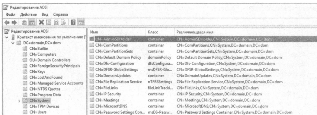
Рис. 7.32. Объект AdminSDHolder
