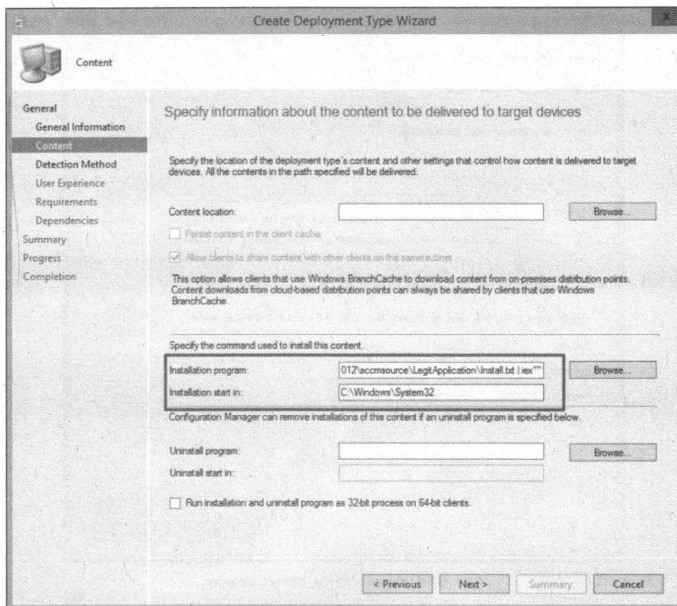
Рис. 3.15. Установка приложения
