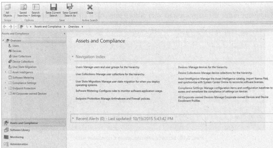
Рис. 3.11. Консоль SCCM
