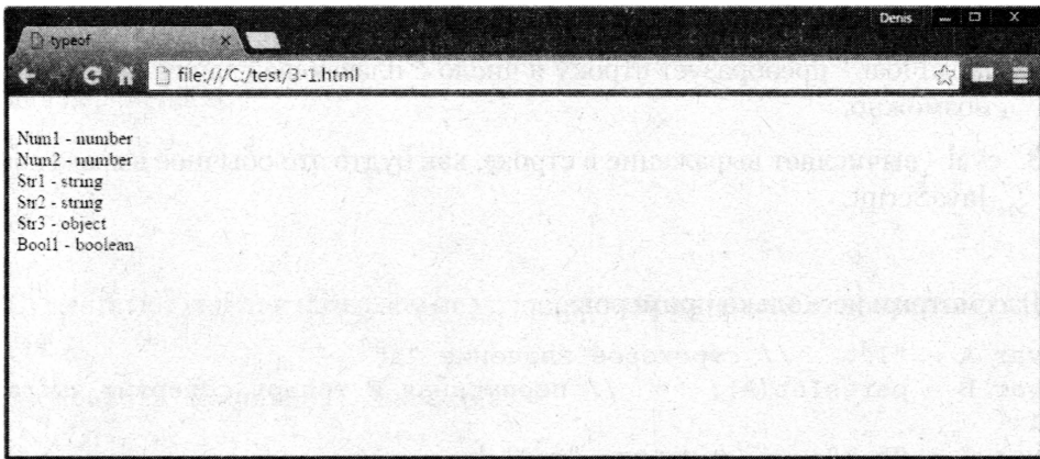
Рис. 3.1. Пример использования оператора typeof
