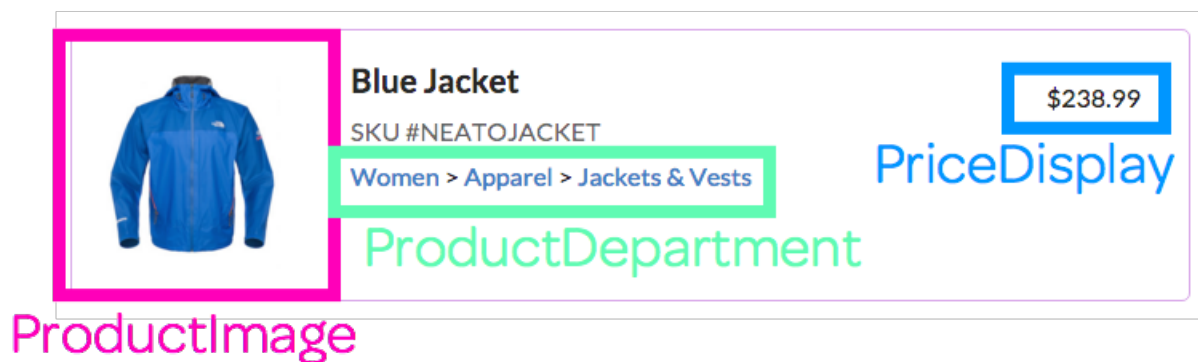
ProductRow’s Sub-components
