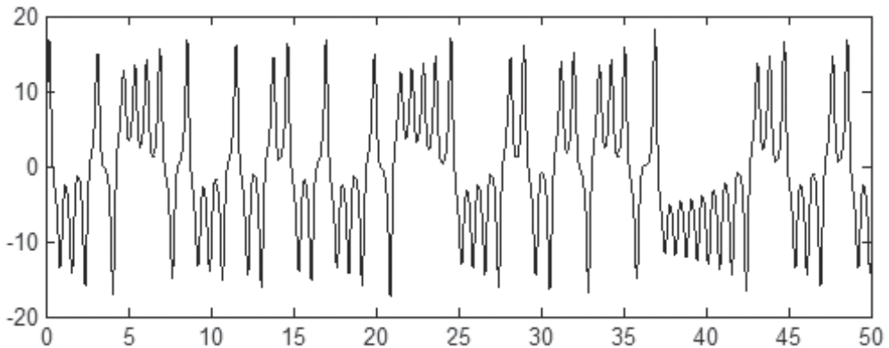
Рис. 1.2.4. График решения x(t)
