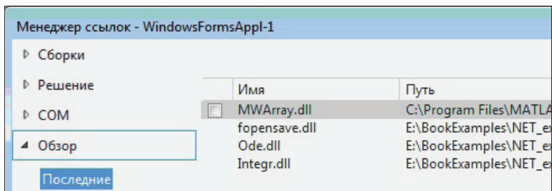
Рис.4.1.7. Менеджер ссылок
