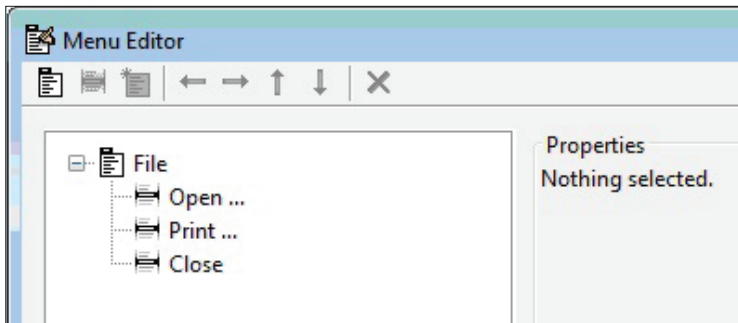
Рис. 1.4.6. Конструктор меню
