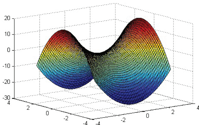
Рис. 1.2.7. График функции двух переменных
