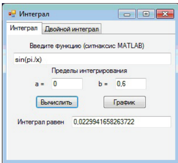
Рис. 4.3.2. Вычисление интеграла
