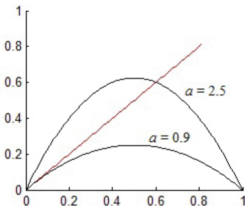
Рис. 1.4.10. Неподвижные точки функции y = ax(1 - x) , при a \in (1, 4]
