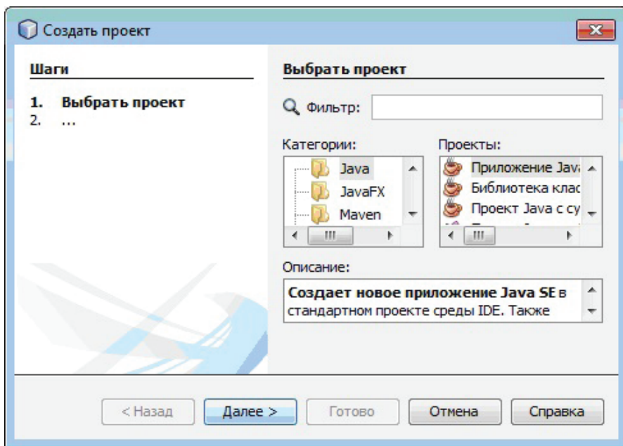
Рис. 3.3.8. Выбор проекта
