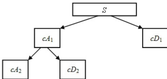
Рис. 4.3.15 Схема вейвлет-разложения
