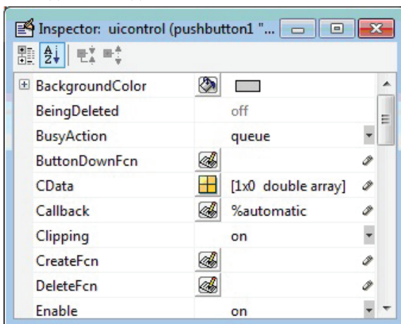
Рис. 1.4.4. Инспектор свойств
