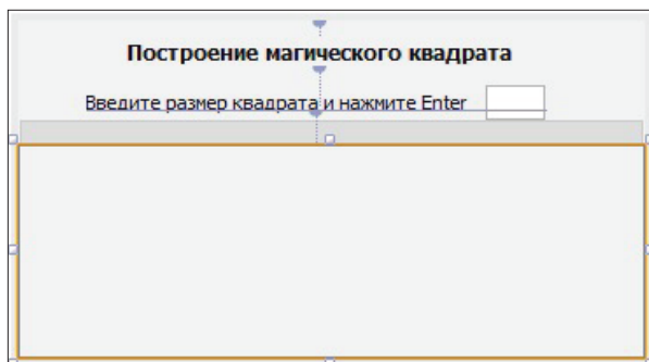
Рис. 3.3.19. Окно приложения
