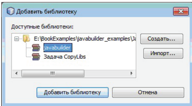
Рис. 3.3.13. Добавление библиотеки
