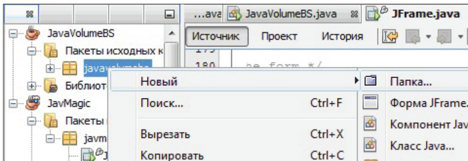
Рис. 3.3.14. Создание формы
