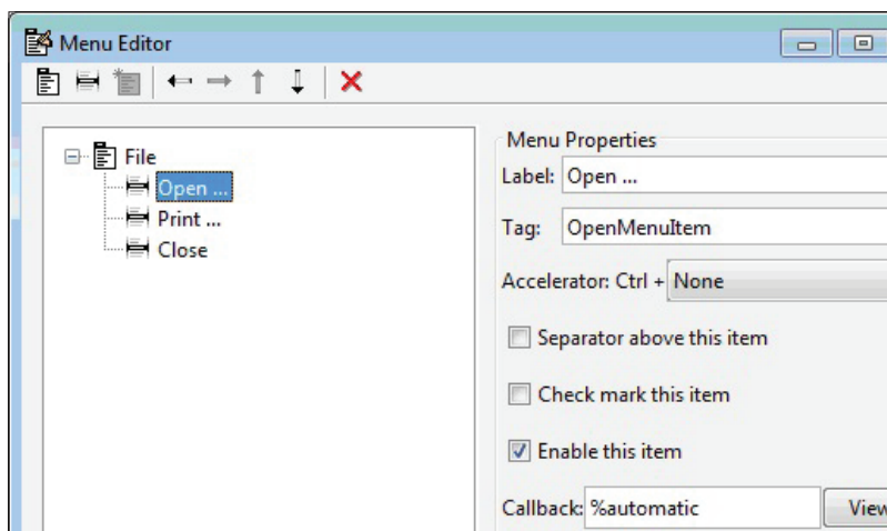
Рис. 1.4.7. Меню File
