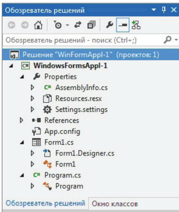
Рис.4.1.5. Обозреватель решений
