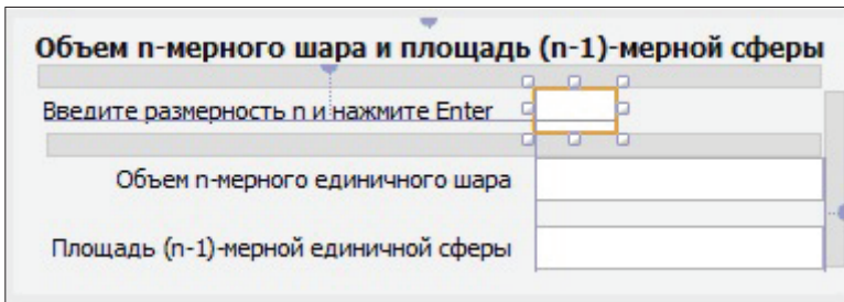
Рис. 3.3.15. Окно приложения
