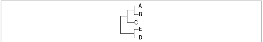
Рис. 12.13. Дендрограмма кластеризованных букв
