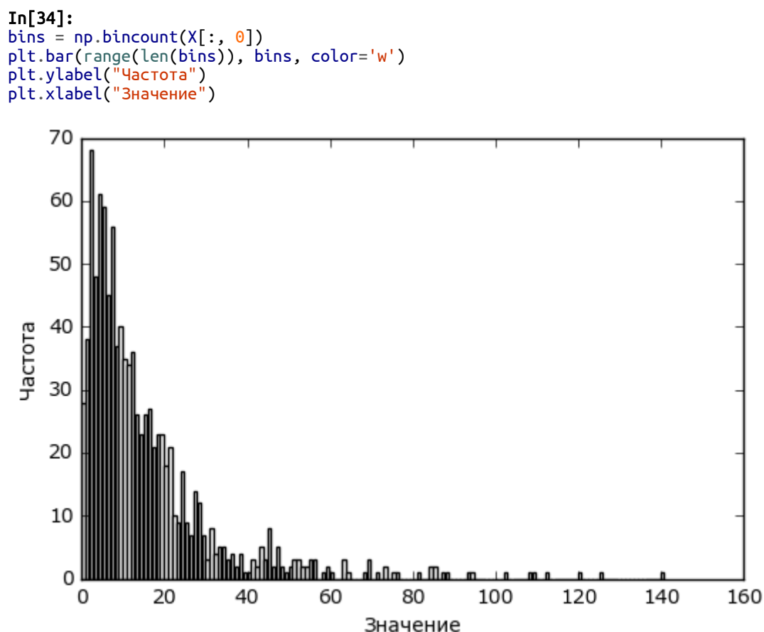
Рис. 4.7 Гистограмма значений X[0]
