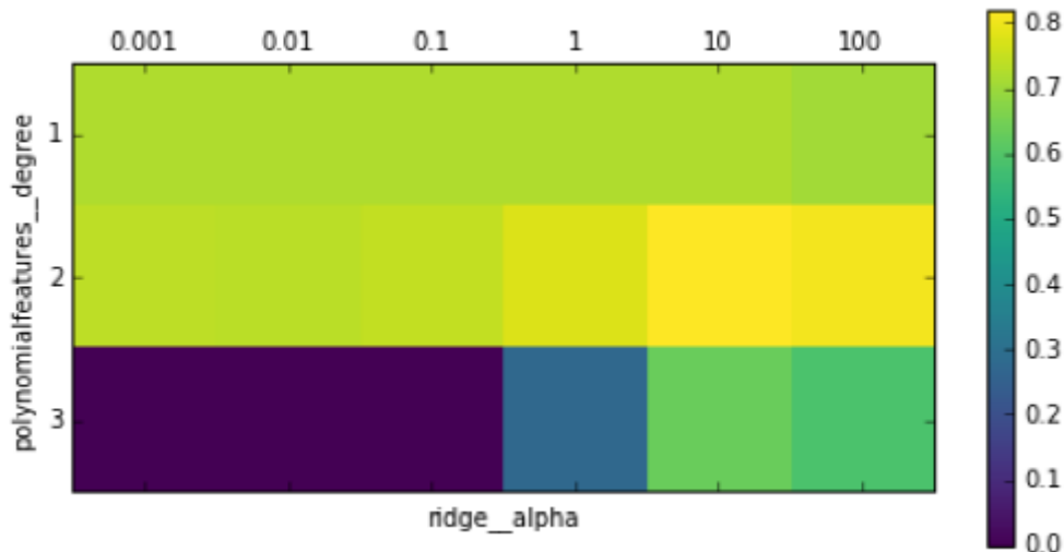
Рис. 6.4 Теплокорта для усредненной правильности перекрестной проверки, выраженной в виде функции двух параметров: параметра degree для полиномиального преобразования и параметра alpha для гребневой регрессии
