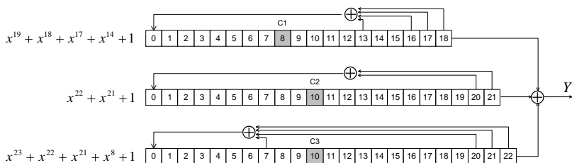
Рис. 6.4 – Регистр сдвига алгоритма шифрования A5/1
