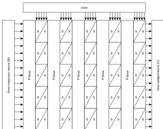
Рис. 5.4 – Общий вид (упрощённая схема) функции шифрования в одном из вариантов проекта «Люцифер». Входной блок (в проекте «Люцифер» его объём – 128 бит) подавался на вход на несколько слоёв (в «Люцифере» слоёв 16) из р-блоков и пар s-блоков. S-блок в каждой паре выбирался в зависимости от значения соответствующего бита ключа
