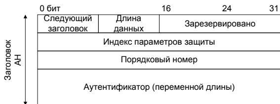
Рис. 13.5 – Заголовок АН пакета
