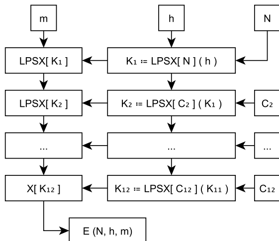
Рис. 8.3 – XSPL-шифр в хэш-функции «Стрибог»
