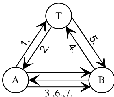
Рис. 11.19 – Взаимодействие участников в протоколе Ву — Лама
