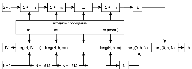
Рис. 8.1 – Использование структуры Меркла — Дамгарда в хэш-функции «Стрибог»
