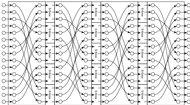
Рис. 5.3 – SP-сеть, состоящая из 4 p-блоков и 3 слоёв s-блоков, по 5 блоков в каждом слое
