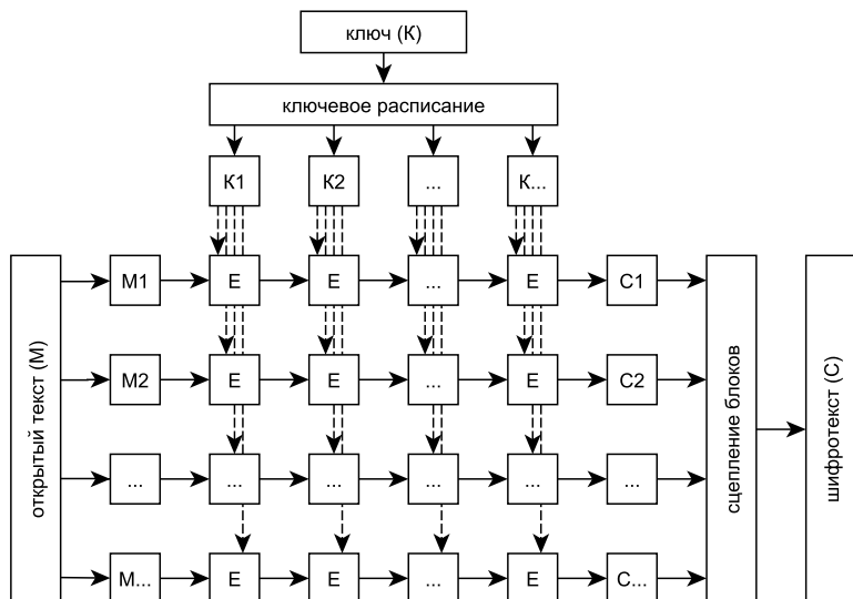
Рис. 5.1 – Общая структура раундового блочного шифра. С помощью функции ключевого расписания из ключа K получается набор раундовых ключей K1, K2, \dots . Открытый текст M разбивается на блоки M1, M2, \dots , каждый из которых проходит несколько раундов шифрования, используя соответствующие раундовые ключи. Результаты последних раундов шифрования каждого из блоков объединяются в шифротекст C с помощью одного из режимов сцепления блоков
