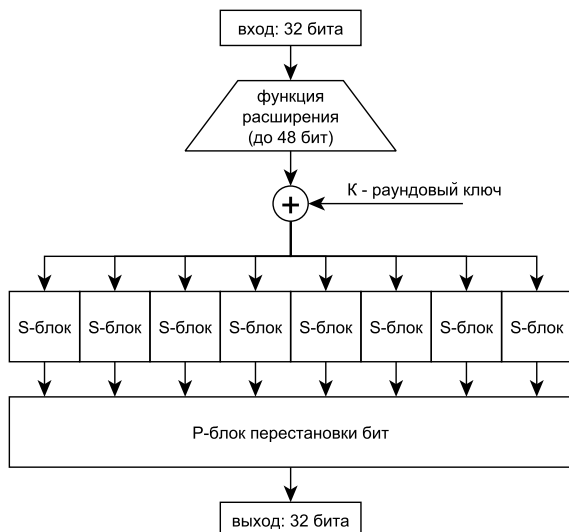
Рис. 5.6 – Функция Фейстеля шифра DES
