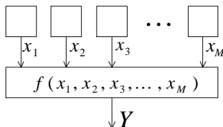
Рис. 6.3 – Криптографический генератор с нелинейной булевой функцией
