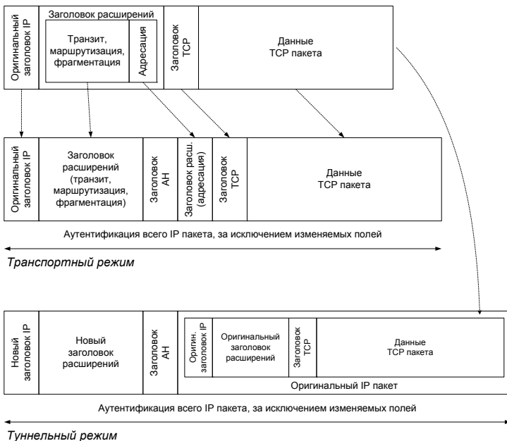
Рис. 13.6 – Применение протокола АН к пакету IPv6
