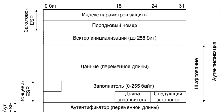
Рис. 13.3 – Формат ESP-пакета
