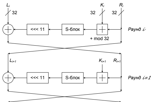
Рис. 5.7 – Схема ГОСТ 28147-89
