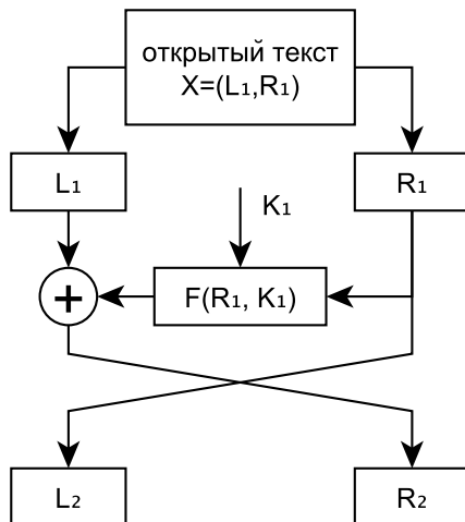
Рис. 5.5 – Ячейка Фейстеля
