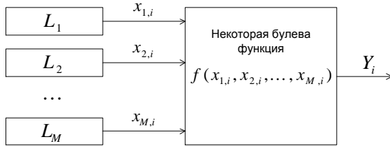
Рис. 6.2 – Генератор с несколькими регистрами сдвига
