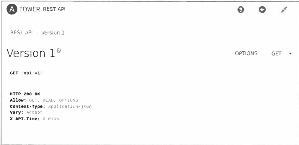
Рис. 19.9 ❖ Ansible Tower API версии 1
