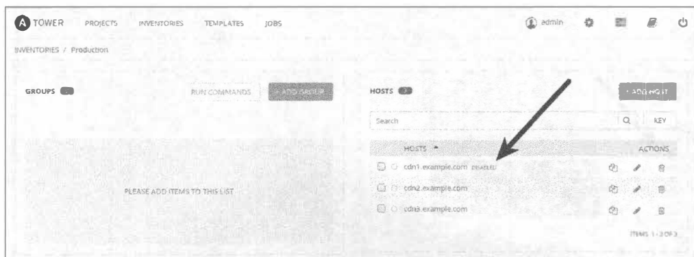
Рис. 19.5. Исключение хостов из обработки в Ansible Tower
