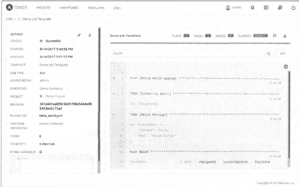
Рис. 19.8 ❖ Подробный обзор результатов задания в Ansible Tower
