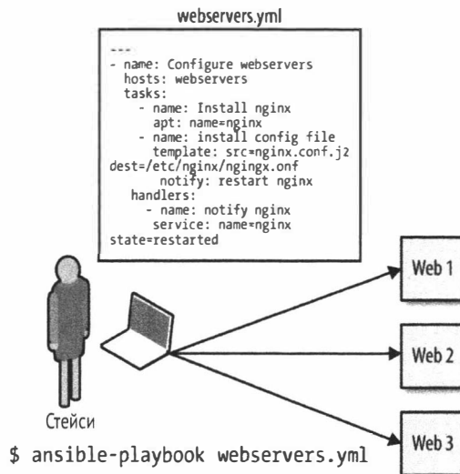
Рис. 1.1 ❖ Ansible выполняет сценарий настройки трех веб-серверов
