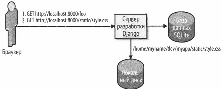
Рис. 5.2 ❖ Приложение Django в режиме разработки
