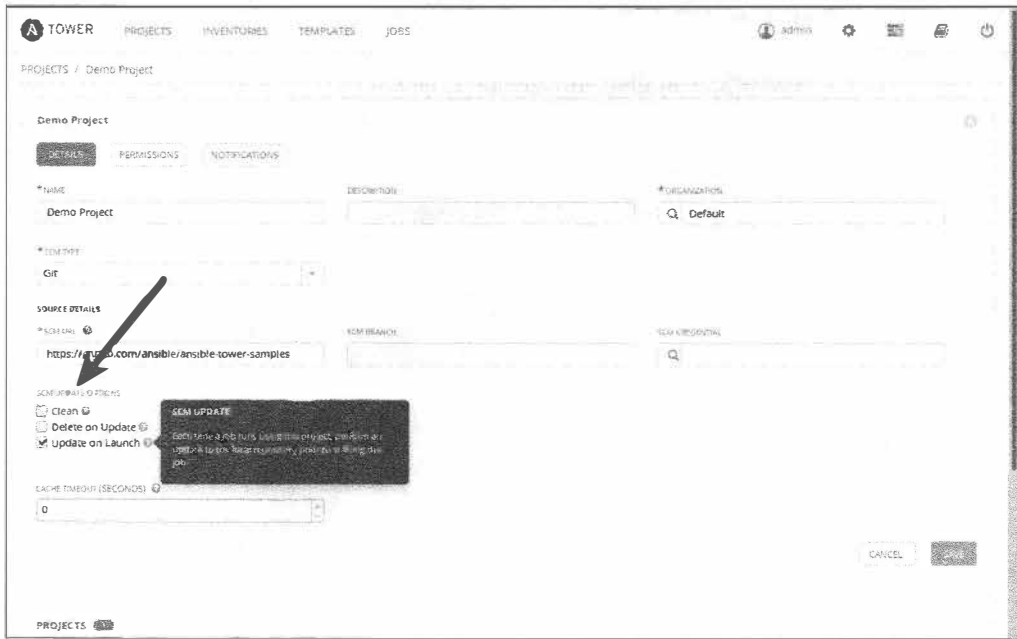
Рис. 19.3 ❖ Параметры настройки обновления проекта из системы управления версиями в Ansible Tower
