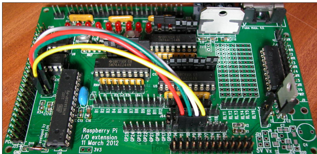
Рис. 6.33. Перемычки для соединения ATmega ISP
