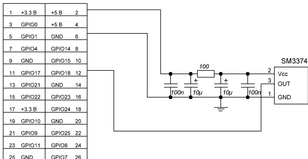
Рис. 6.9. Схема подключения ИК-ресивера SM3374 к Raspberry Pi
