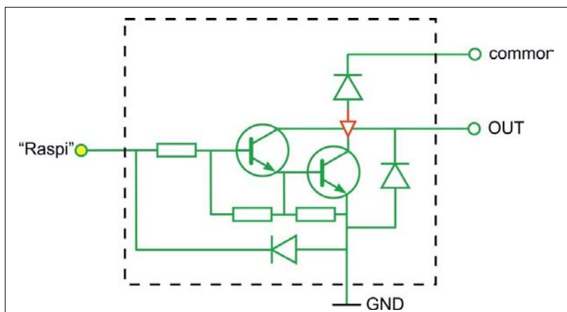
Рис. 6.30. Схема подключения блока драйвера с открытым коллектором
