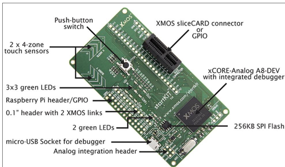
Рис. 6.47. Плата XMOS StartKIT
