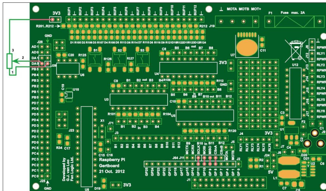
Рис. 6.32. Схема соединений для теста atod.py
