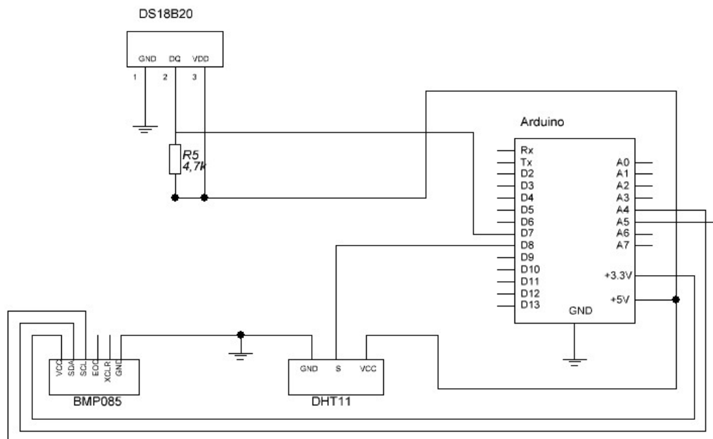
Рис. 4.47. Схема подключения датчиков к Arduino
