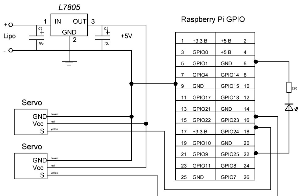
Рис. 6.18. Электрическая схема проекта
