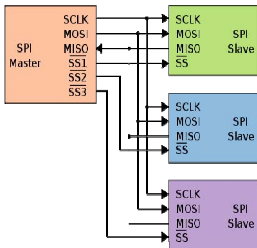
Рис. 6.54. Один из способов подключения SPI
