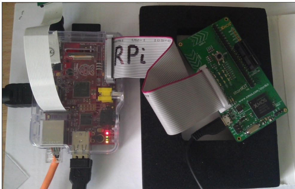
Рис. 6.53. Соединение xMOS StartKIT и Raspberry Pi
