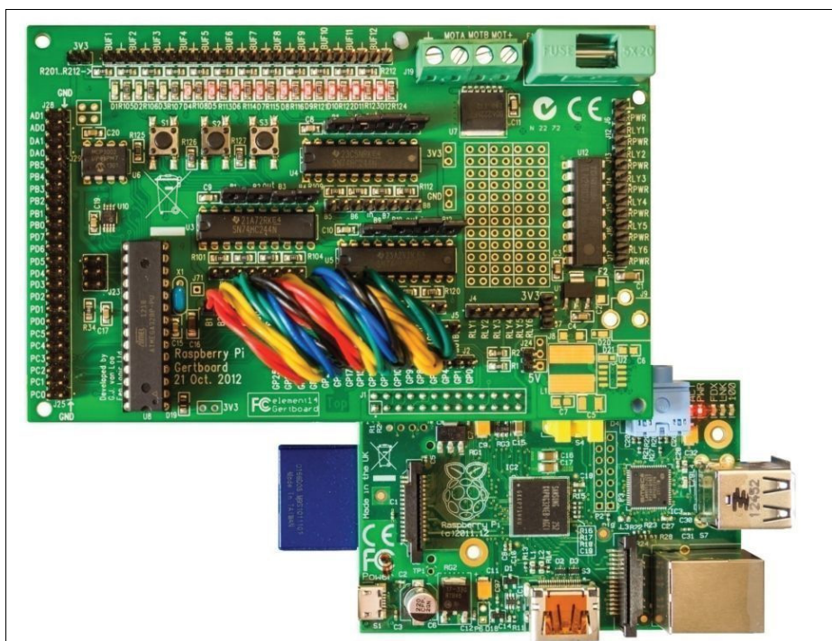
Рис. 6.22. Плата Gertboard, подключенная к Raspberry Pi
