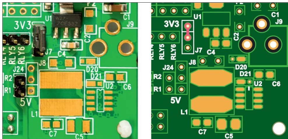
Рис. 6.25. Перемычка для переключения на питание 3,3 В
