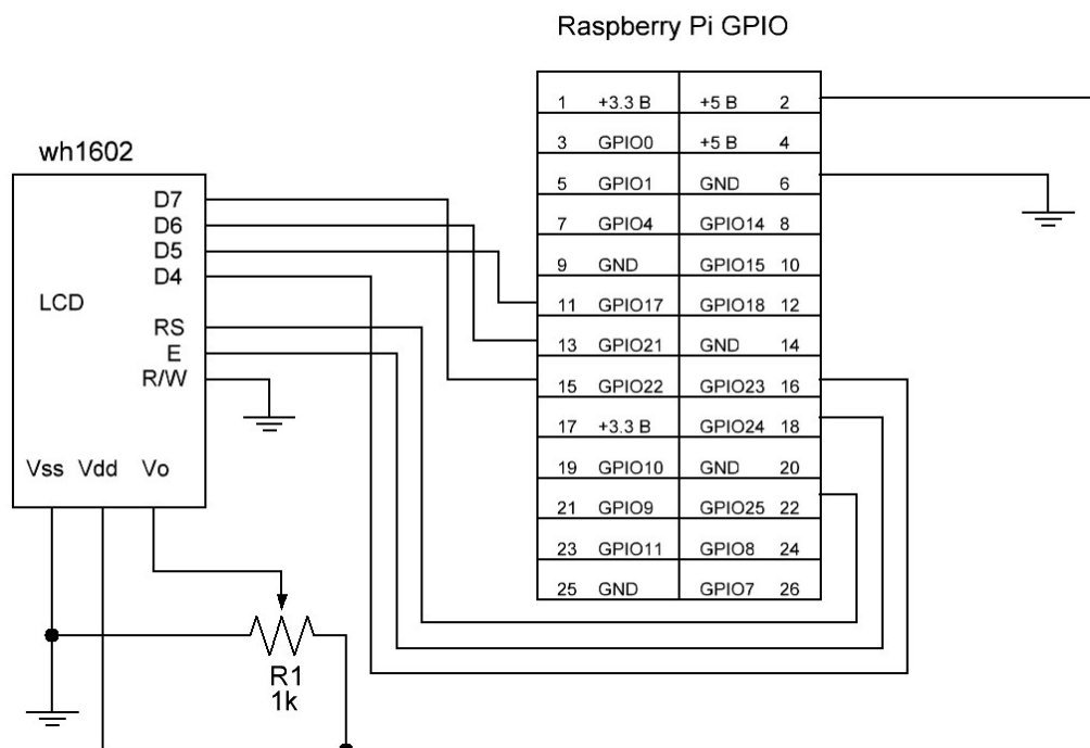
Рис. 6.5. Схема подключения дисплея к выводам GPIO
