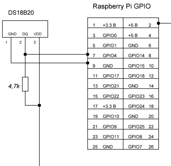
Рис. 6.20. Схема подключения датчика DS18B20
