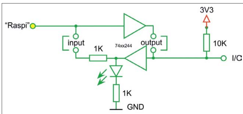
Рис. 6.26. Схема установки переключки портов I/O с 4 по 12
