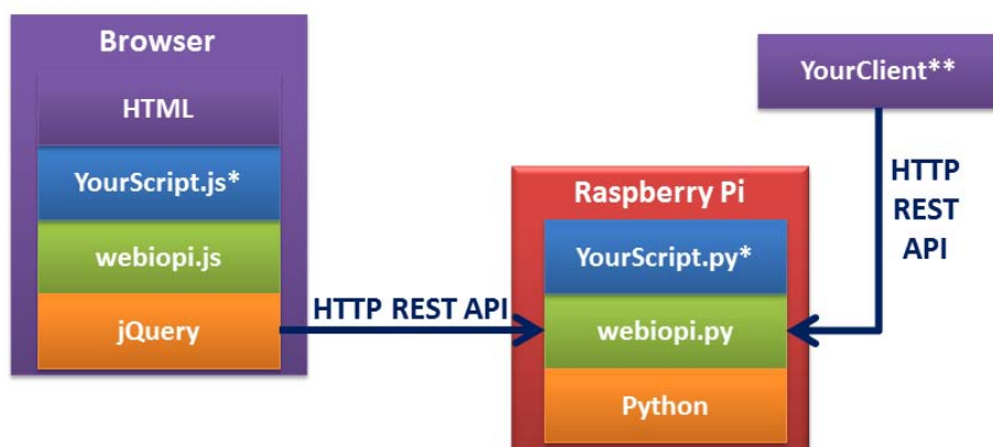
Рис. 6.14. Схема WebIOPI
