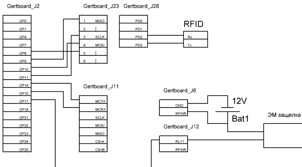
Рис. 6.43. Схема подключения RFID-считывателя
