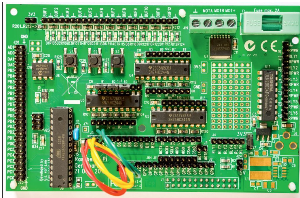
Рис. 6.28. Соединения проводников для теста кнопок
