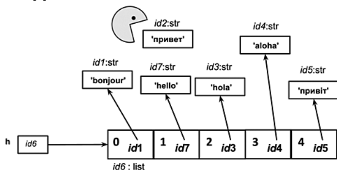
Рис. 4.30. Схема памяти Python в момент изменения списка
