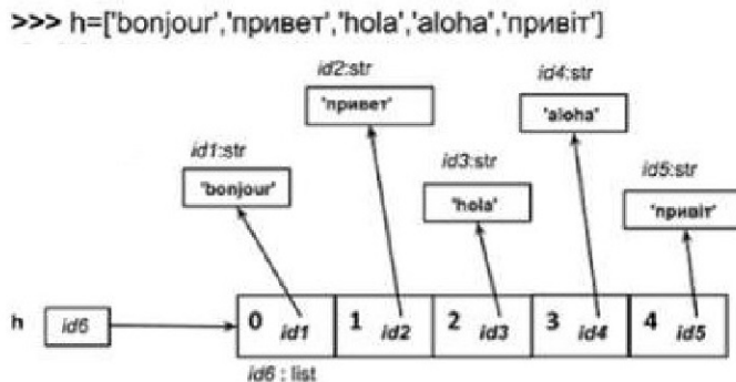
Рис. 4.29. Схема памяти Python при работе со списком
