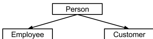
Рис. 4.43. Иерархия классов
