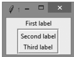
Рис. 4.49. Изменение параметров фрейма при создании объекта
