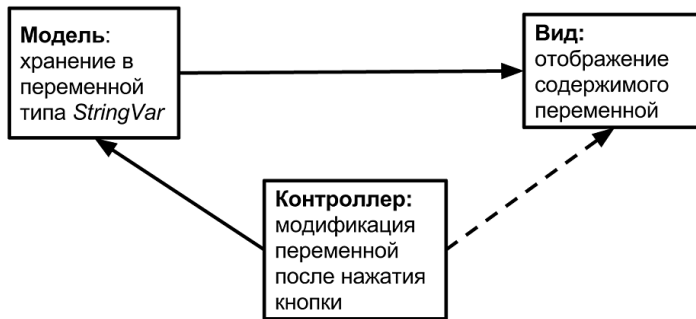
Рис. 4.52. Схема шаблона MVC
