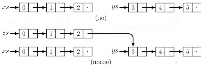
Рис. 2.5: выполнение zs = xs ++ ys в функциональном окружении (заметим, что списки-аргументы xs и ys не затронуты операций).
