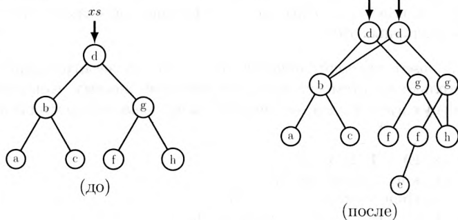
Рис. 2.8: выполнение ys = \text{insert} ("e", xs) (как и прежде, обратите внимание на совместное использование структуры деревьями xs и ys ).
