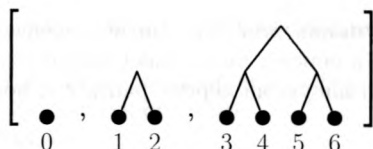
Рис. 9.5: двоичный список с произвольным доступом, содержащий элементы 0 \dots 6 .
