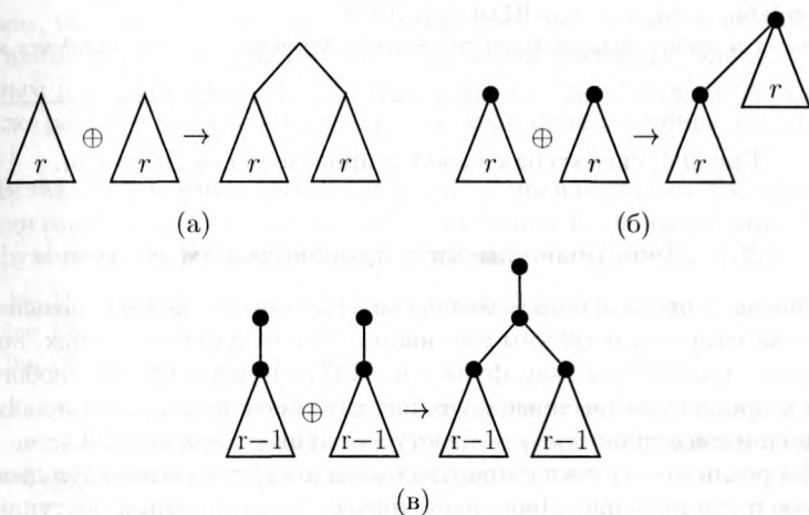
Рис. 9.3: связывание двух деревьев ранга r в дерево ранга r + 1 для (а) полных двоичных листовых деревьев, (б) биномиальных деревьев и (в) подвешенных деревьев.
