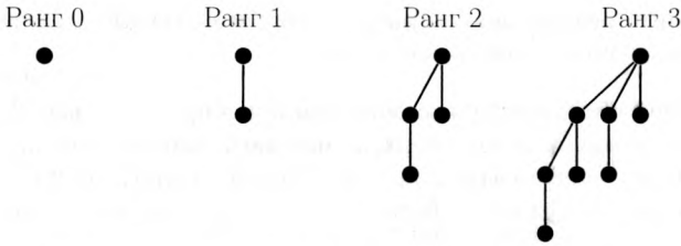
Рис. 3.3: биномиальные деревья рангов 0–3.
