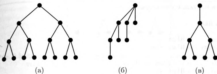
Рис. 9.2: три дерева ранга 3: (а) полное двоичное листовое дерево, (б) биномиальное дерево и (в) подвешенное дерево.
