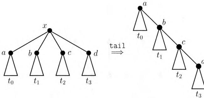
Рис. 10.5: операция tail.
