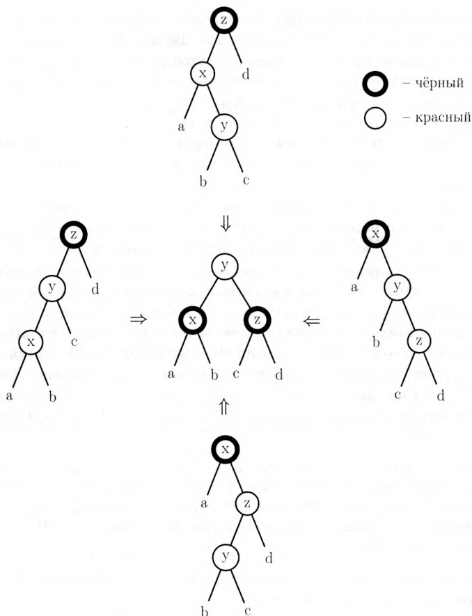
Рис. 3.5: избавление от красных узлов с красными родителями.
