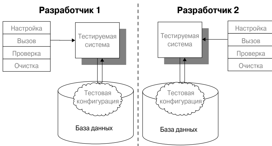
Рис. 13.1. “Песочница” с базой данных (Database Sandbox) для каждого разработчика. Совместное использование “песочницы” несколькими разработчиками — не что иное, как “экономия на свечках” (это все равно что электрик и сантехник, работающие над одной стеной одновременно)
