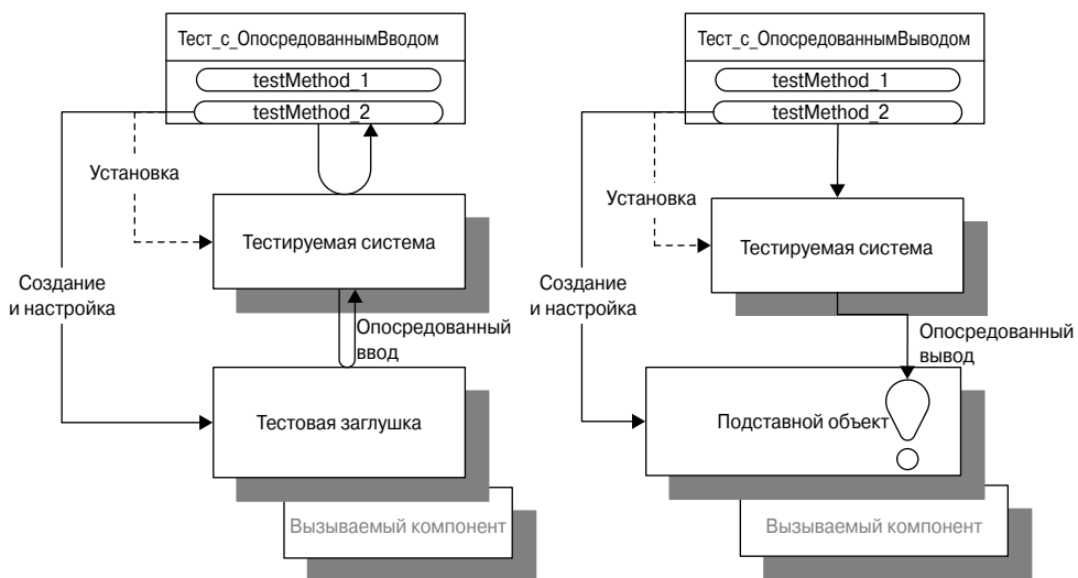
Рис. 6.8. Тест с пересечением уровней (Layer-Crossing Test) может взаимодействовать с тестируемой системой через “черный ход”. Тест слева управляет опосредованным входом тестируемой системы с помощью тестовой заглушки (Test Stub). Тест справа проверяет опосредованный вывод с помощью подставного объекта (Mock Object)
