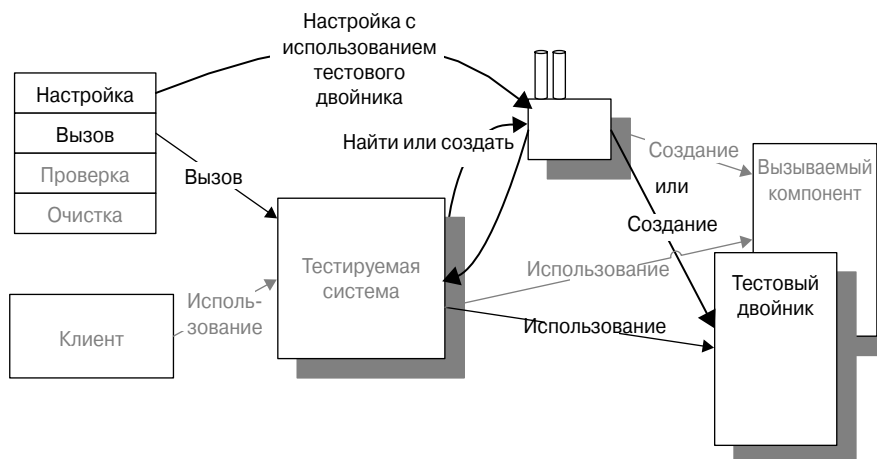
Рис. 11.11. Локатор служб (Service Locator) “настроен” тестом на предоставление тестового двойника (Test Double) тестируемой системе. Использование тестовых двойников (Test Double) предполагает наличие механизма подмены вызываемого компонента. При использовании поиска зависимости (Dependency Lookup) тестируемая система должна запрашивать у широкоизвестного объекта ссылку на вызываемый компонент. Тест может предоставить локатор служб (Service Locator), который будет возвращать ссылку на тестовый двойник (Test Double)
