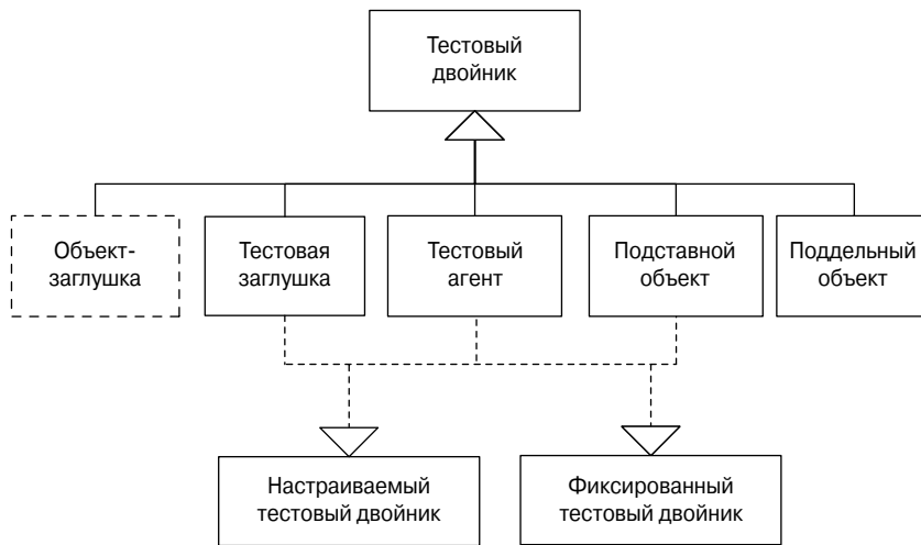
Рис. 11.8. Существует несколько типов тестовых двойников (Test Double). Объект-заглушка (Dummy Object) представляет собой альтернативу шаблонам значений. Тестовая заглушка (Test Stub) используется для проверки опосредованного ввода. Тестовый агент (Test Spy) и подставной объект (Mock Object) проверяют опосредованный вывод. Поддельный объект (Fake Object) эмулирует поведение настоящих вызываемых компонентов, но обладает дружественными к тесту характеристиками
