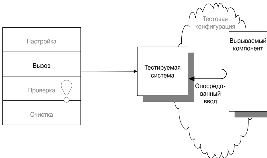
Рис. 11.1. Опосредованный ввод был получен тестируемой системой от вызываемого компонента. Не каждый ввод тестируемой системы предоставляется тестом. Иногда опосредованный ввод предоставляется другими вызываемыми компонентами в виде возвращаемых значений, модифицированных параметров или исключений
