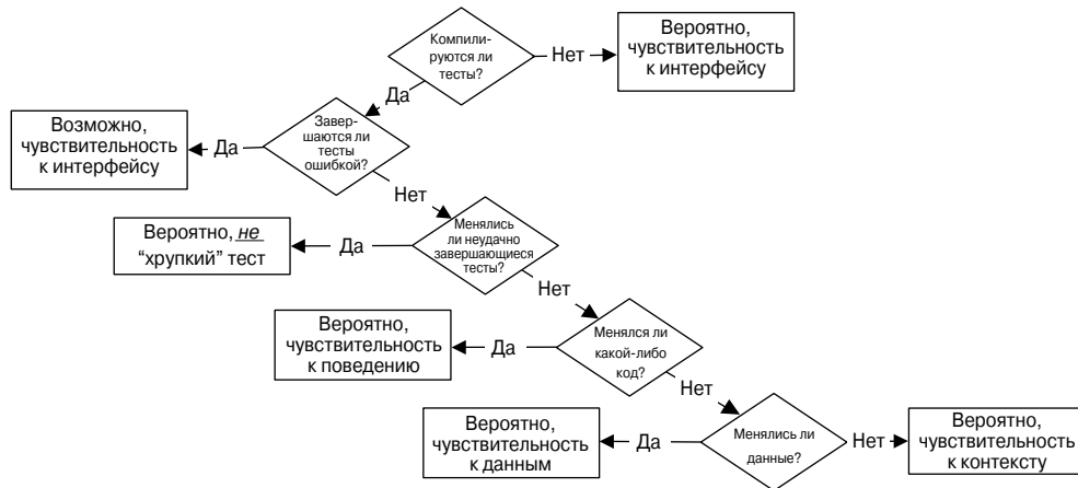
Рис. 16.2. Диагностика “хрупкого” теста
