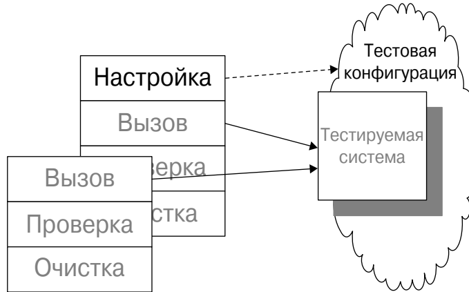
Рис. 9.2. Общая тестовая конфигурация (Shared Fixture) и два использующих ее тестовых метода (Test Method). Общая тестовая конфигурация (Shared Fixture) создается один раз и используется несколькими тестами, которые в результате намеренно или ненамеренно взаимодействуют друг с другом. Обратите внимание на отсутствие фазы настройки тестовой конфигурации во втором тесте
