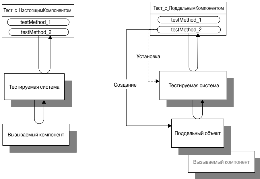
Рис. 6.7. Обычный тест взаимодействует с тестируемой системой только через “главный вход”. Тест справа замещает вызываемый компонент поддельным объектом (Fake Object) для обеспечения повторяемости и повышения быстродействия
