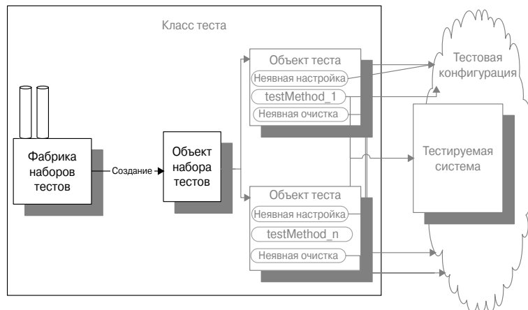
Рис. 12.6. Класс теста (Testcase Class) выступает в роли фабрики наборов тестов (Test Suite Factory). По умолчанию класс теста (Testcase Class) выступает в роли фабрики наборов тестов (Test Suite Factory) и создает объект набора тестов (Test Suite Object), необходимый программе запуска тестов (Test Runner). Кроме того, можно перечислить конкретное подмножество запускаемых тестов, создав фабрику наборов тестов (Test Suite Factory), возвращающую объект набора тестов (Test Suite Object) с интересующими разработчика тестами
