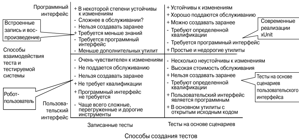
Рис. 6.3. Варианты на передней грани. Это более подробное представление передней грани, показанной на рис. 6.2. Здесь также показаны преимущества (+) и недостатки (–) каждого подхода
