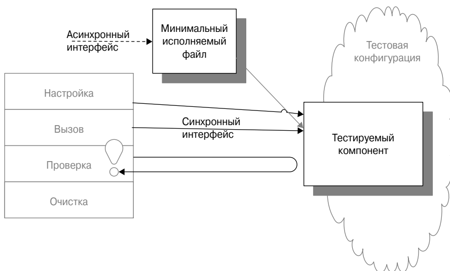
Рис. 6.11. Используя минимальный выполняемый файл (Humble Executable), можно упростить тесты. Данный шаблон улучшает повторяемость и скорость проверки логики, которую в противном случае пришлось бы проверять асинхронными тестами
