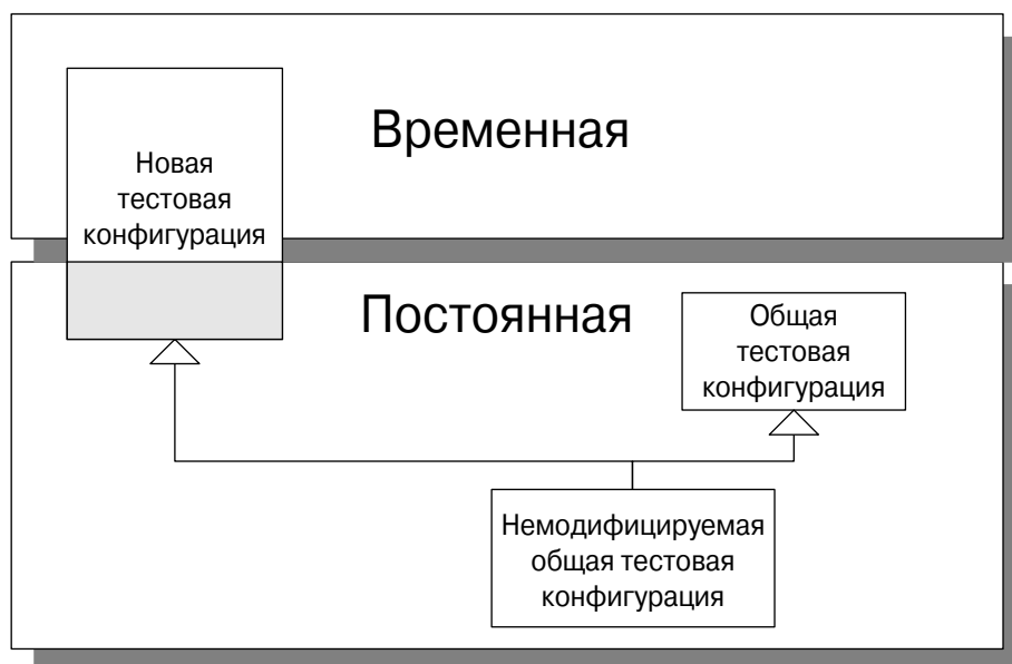
Рис. 8.1. Временная новая тестовая конфигурация (Transient Fresh Fixture). Новая тестовая конфигурация (Fresh Fixture) может быть двух видов — временной (transient) и постоянной (persistent). Оба типа требуют создания тестовой конфигурации. Последний тип также требует очистки тестовой конфигурации
