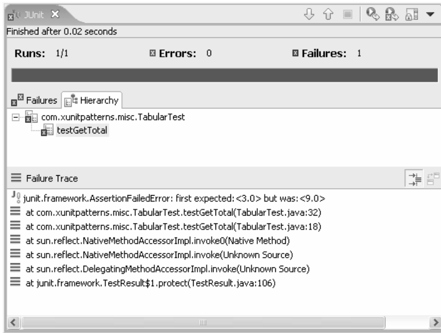
Рис. 20.3. Результаты выполнения табличного теста (Tabular Test). На нижней панели приведена информация о неудачном завершении метода табличного теста, представленного на верхней панели. Из-за неудачного завершения оставшаяся часть метода не выполняется
