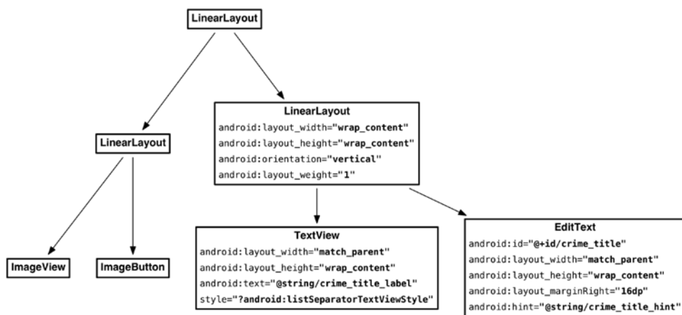
Рис. 16.4. Макет текстовой части (res/layout/view_camera_and_title.xml)
