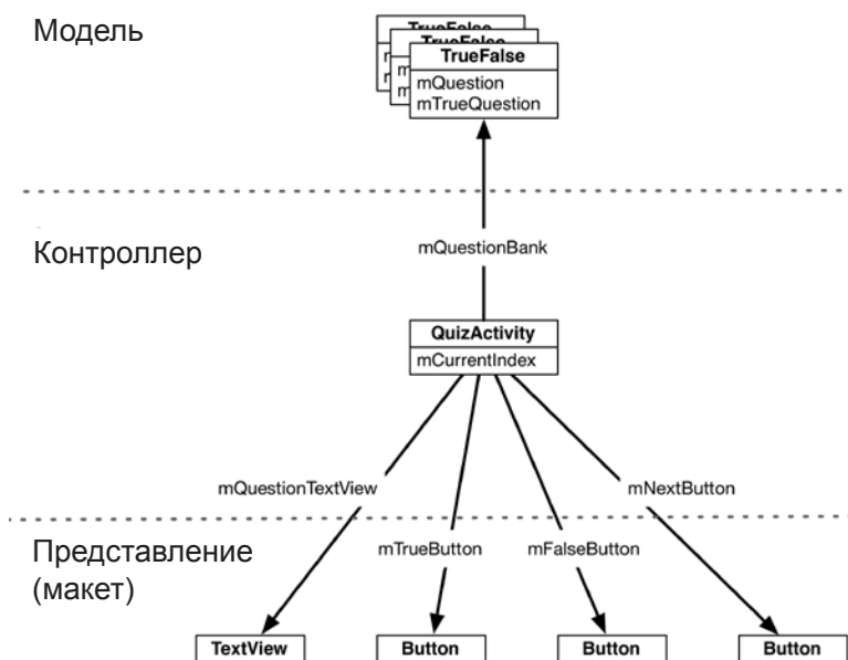
Рис. 2.4. Диаграмма объектов GeoQuiz
