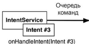
Рис. 26.1. Как IntentService обслуживает команды
