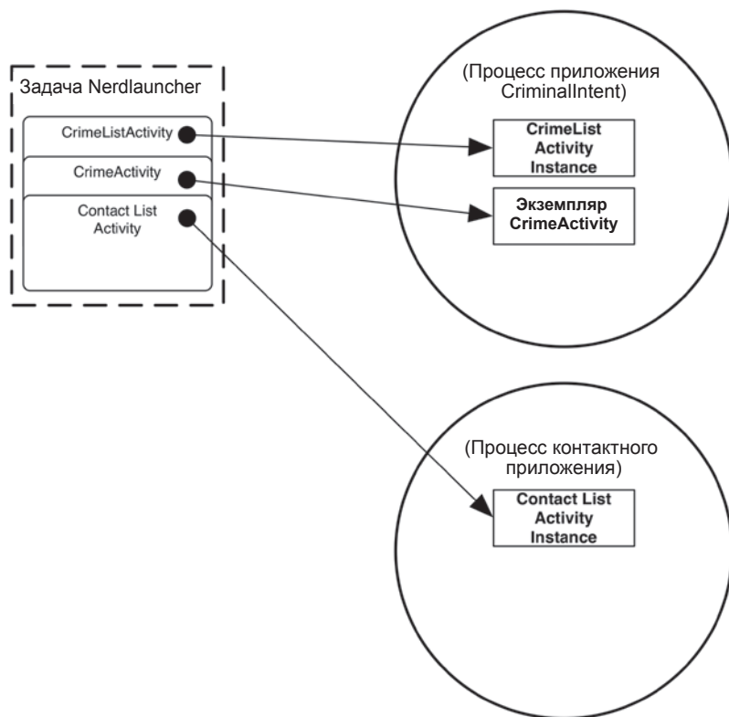
Рис. 22.13. Задачи и процессы
