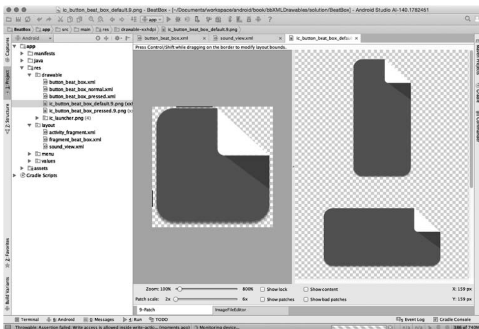
Рис. 21.9. Создание 9-зонного изображения
