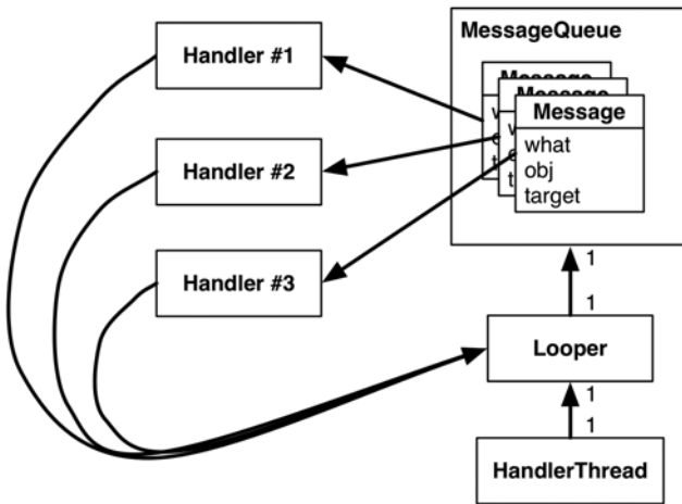
Рис. 24.5. Несколько объектов Handler, один объект Loop
