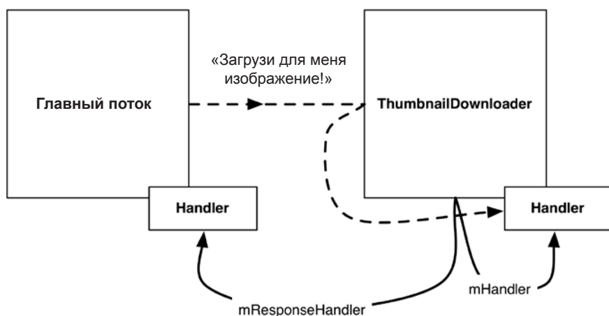
Рис. 24.7. Планирование операций в ThumbnailDownloader из главного потока
