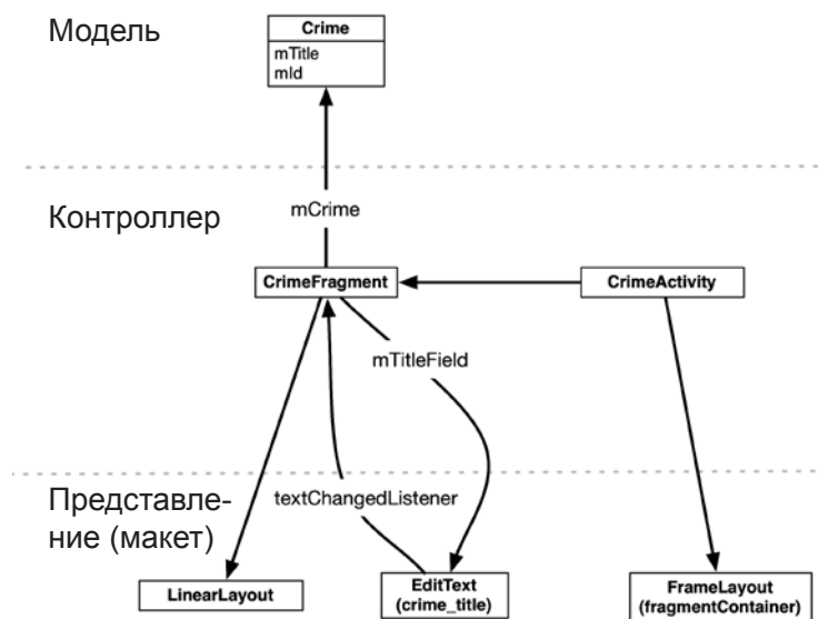
Рис. 7.6. Диаграмма объектов CriminalIntent (для этой главы)
