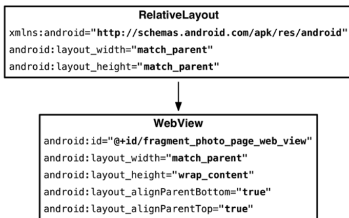
Рис. 28.2. Исходный макет (res/layout/fragment_photo_page.xml)
