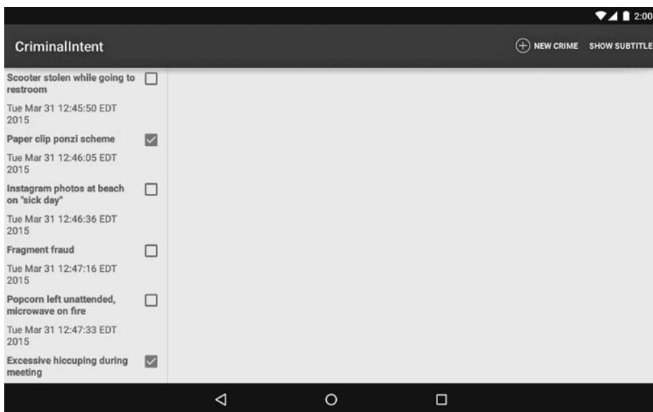
Рис. 17.5. Двухпанельный макет на планшете
