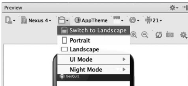
Рис. 5.6. Просмотр макета activity_cheat.xml в альбомной ориентации
