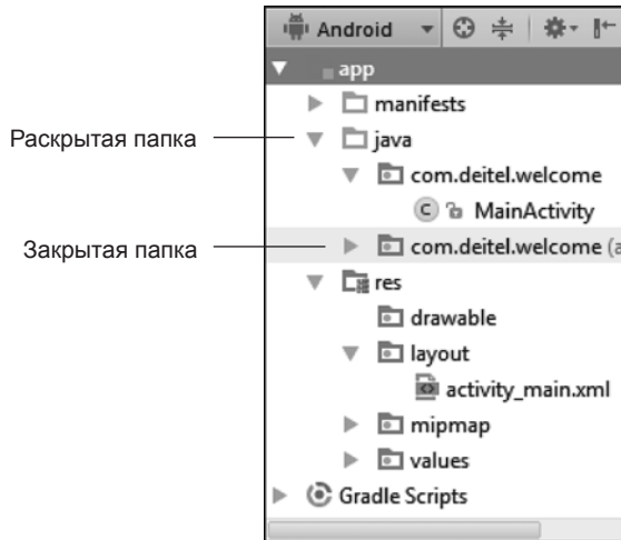
Рис. 2.7. Окно Project
