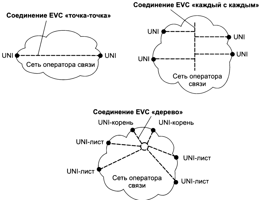
Рис. 20.19. Три типа услуг Ethernet
