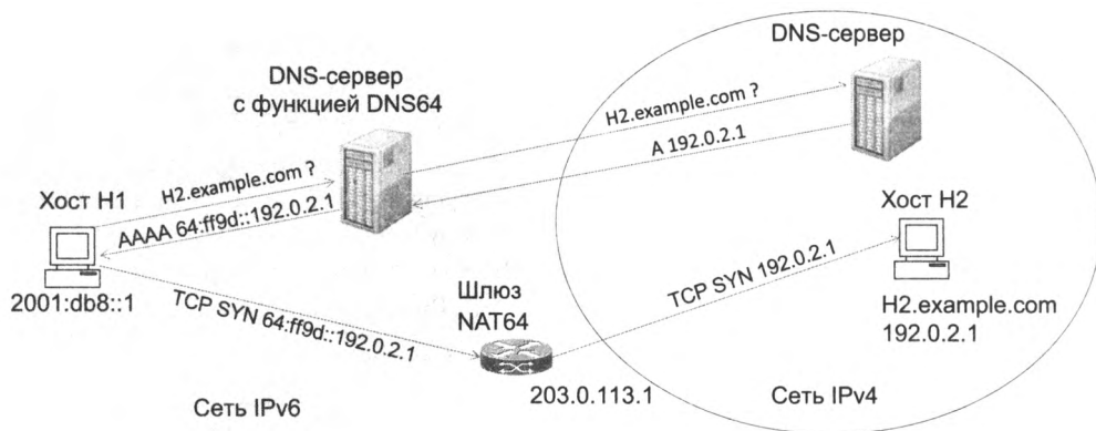
Рис. 17.19. Трансляция протоколов IPv6 ↔ IPv4 с использованием технологии NAT64
