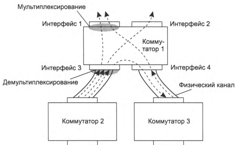
Рис. 2.16. Операции мультимплексирования и демultipлексирования потоков при коммутации
