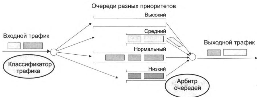
Рис. 5.14. Приоритетные очереди
