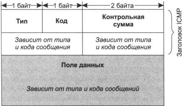
Рис. 14.14. Формат ICMP-сообщения
