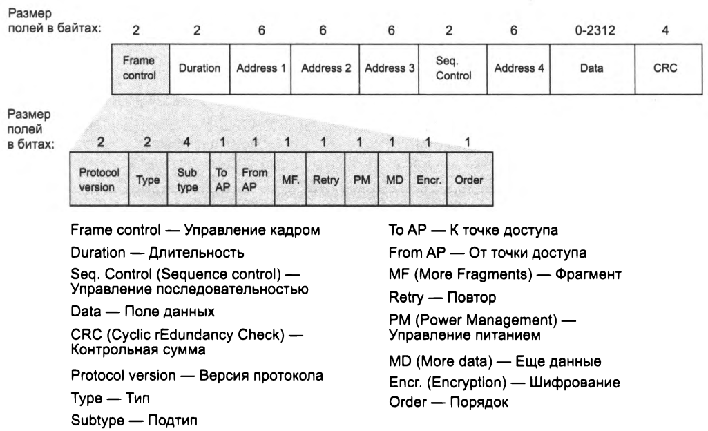
Рис. 22.6. Формат кадра Wi-Fi
