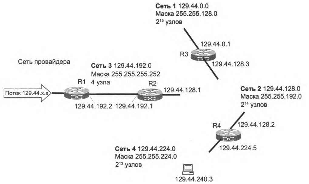
Рис. 14.12. Структуризация сети масками переменной длины
