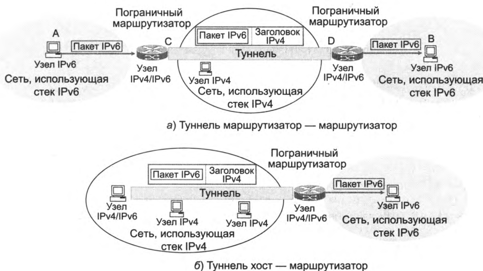
Рис. 17.18. Согласование технологий IPv4 и IPv6 путем туннелирования
