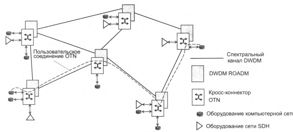
Рис. 9.19. Коммутируемая сеть OTN/DWDM
