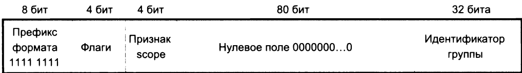
Рис. 17. 4. Формат группового адреса IPv6
