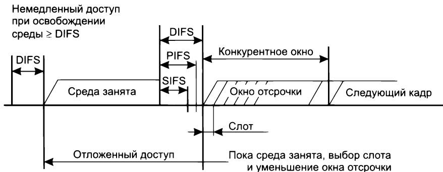
Рис. 22.8. Сосуществование режимов PCF и DCF
