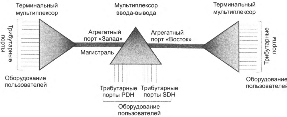
Рис. 8.3. Простейшая первичная сеть
