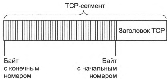
Рис. 15.15. Нумерация байтов в TCP-сегменте
