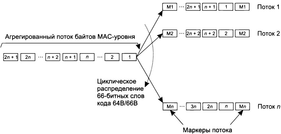
Рис. 10.18. Распределение данных подуровнем PCS по потокам
