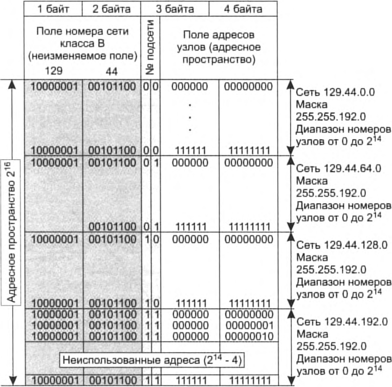
Рис. 14.9. Разделение адресного пространства 129.44.0.0 сети класса В на четыре равные части
