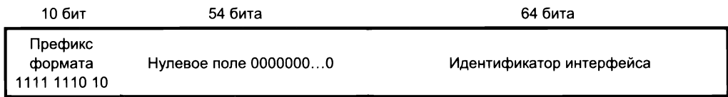
Рис. 17.3. Формат адреса уровня линии связи
