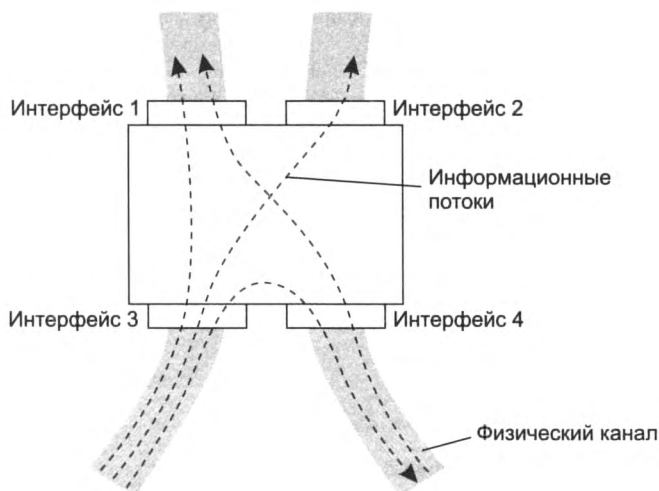
Рис. 2.14. Коммутатор
