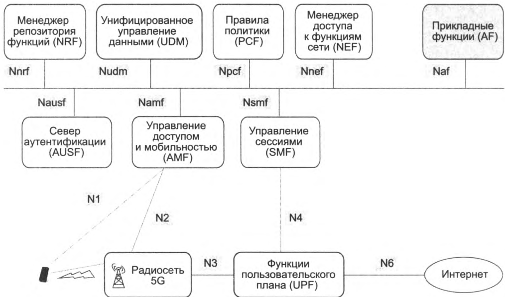
Рис. 23.12. Представление архитектуры 5G, основанное на услугах
