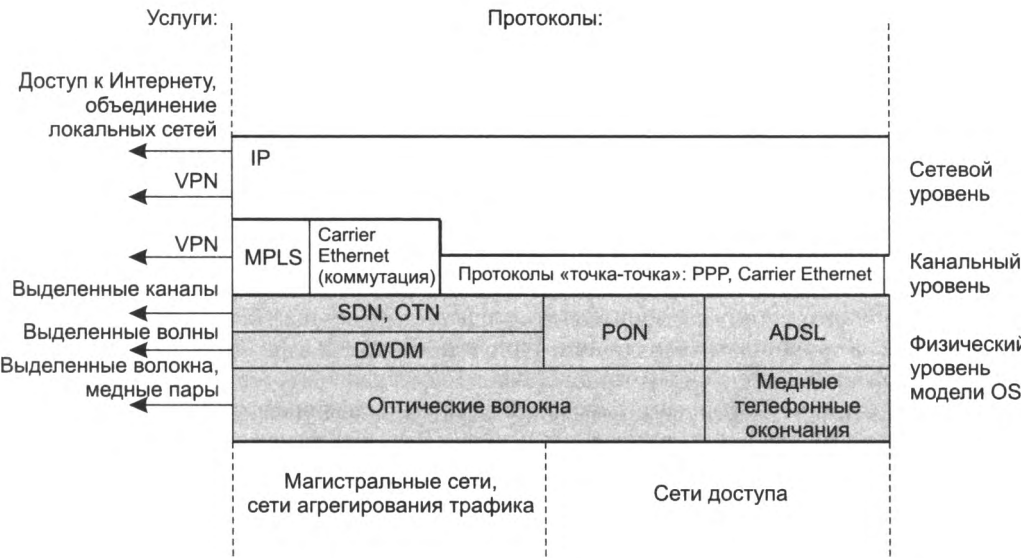
Рис. 18.5. Многослойная структура сети оператора связи/поставщика услуг Интернета
