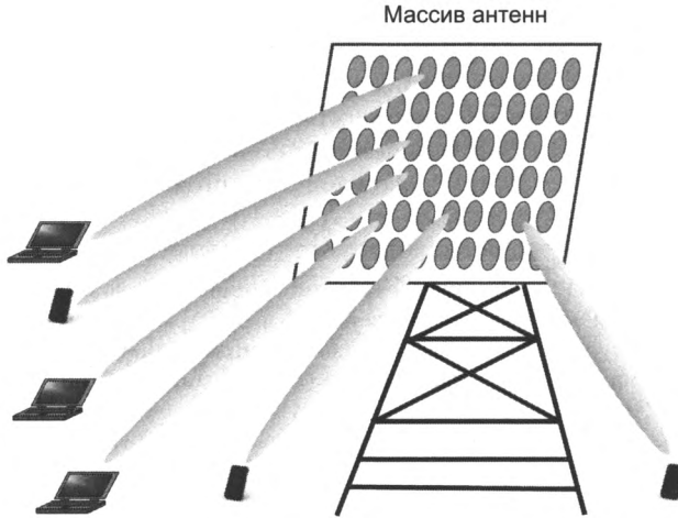
Рис. 21.11. Формирование диаграммы направленности системой Massive MIMO
