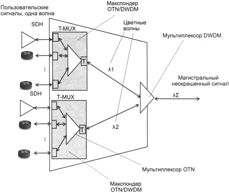
Рис. 9.18. Сеть OTN/DWDM с макспондерами
