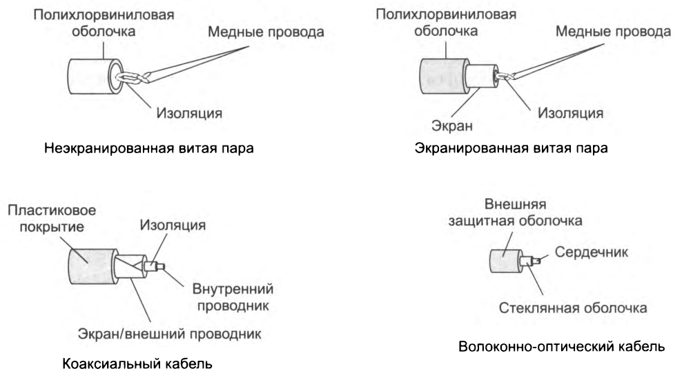
Рис. 6.19. Устройство кабелей
