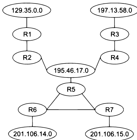
Рис. 16.2. Граф сети, построенный протоколом OSPF
