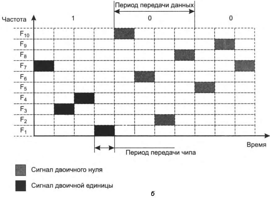
Рис. 21.14. Соотношение между скоростью передачи данных и частотой смены подканалов
