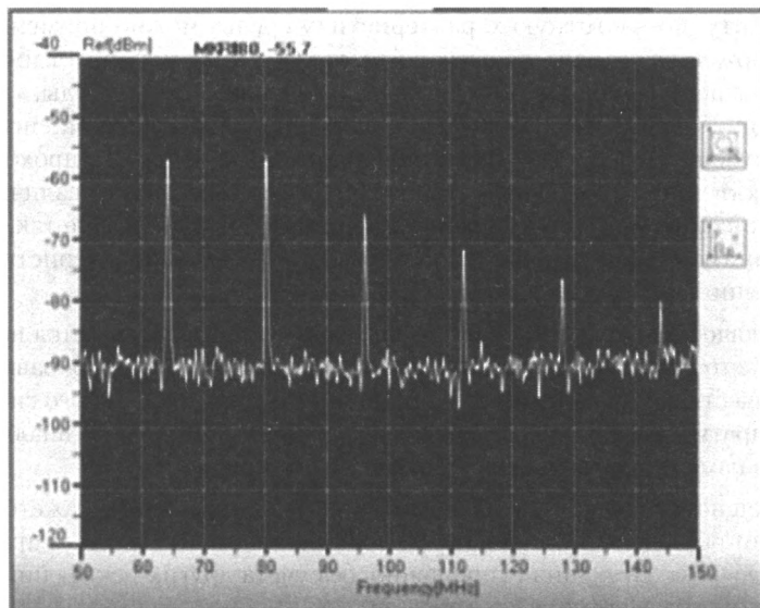
Рис. 6.8. Спектр сигнала, найденного спектральным анализатором
