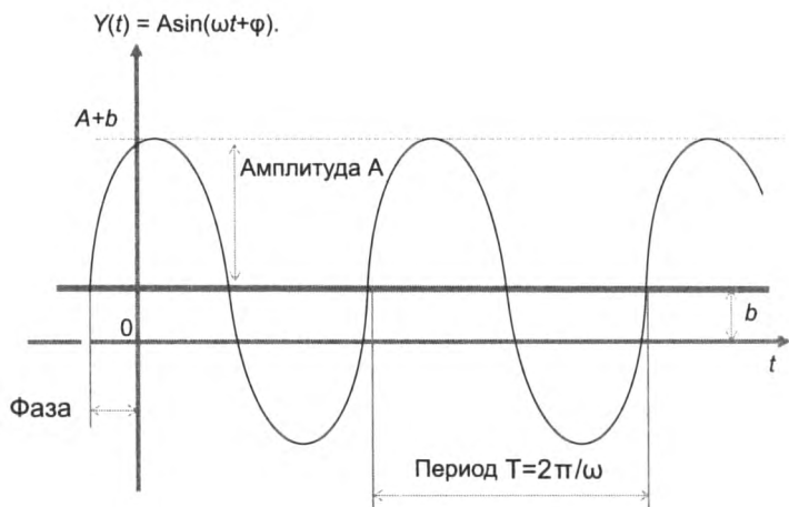
Рис. 6.4. Синусоида
