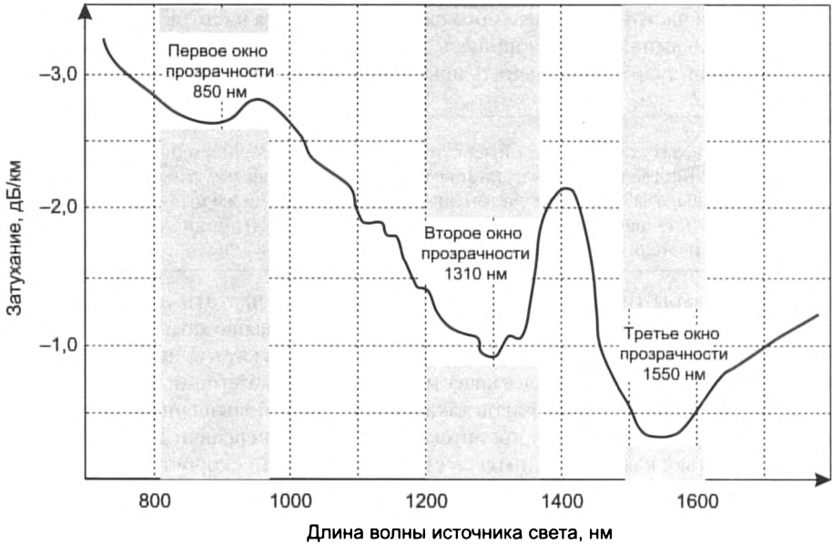
Рис. 6.11. Окна прозрачности оптического волокна
