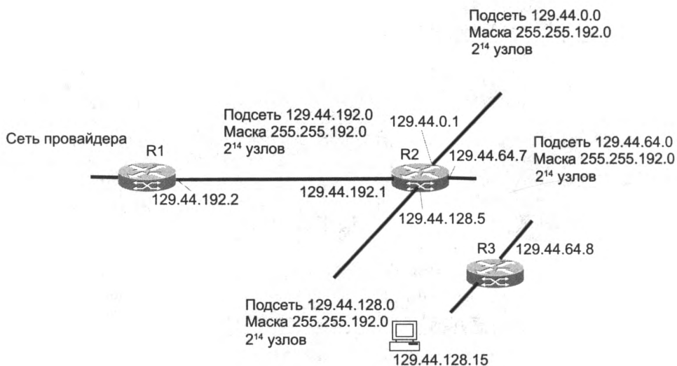
Рис. 14.10. Маршрутизация с использованием масок одинаковой длины
