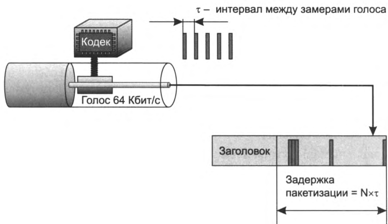
Рис. 19.5. Задержка пакетизации
