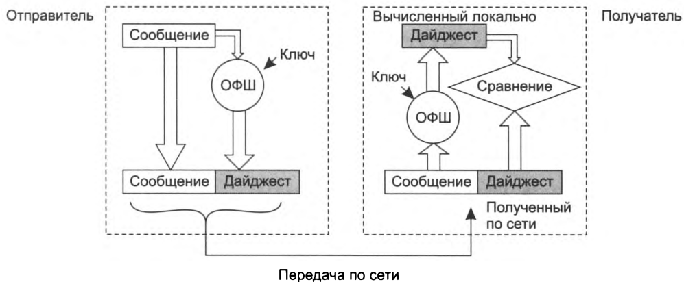
Рис. 26.11. Использование параметрической односторонней функции шифрования для контроля целостности
