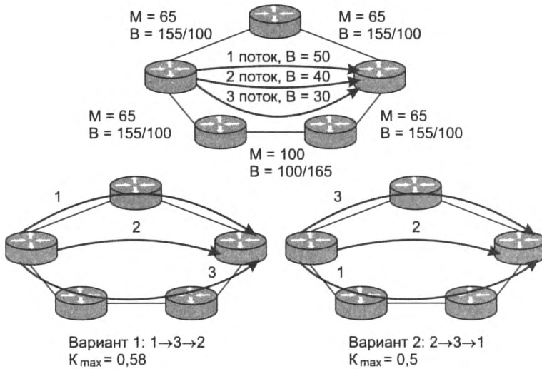
Рис. 20.12. Зависимость качества решения задачи ТЕ от очередности выбора туннелей
