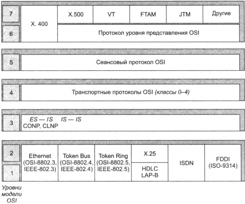
Рис. 4.10. Стек протоколов OSI
