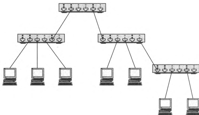
Рис. 3.16. Древовидная топология коммутируемой сети Ethernet
