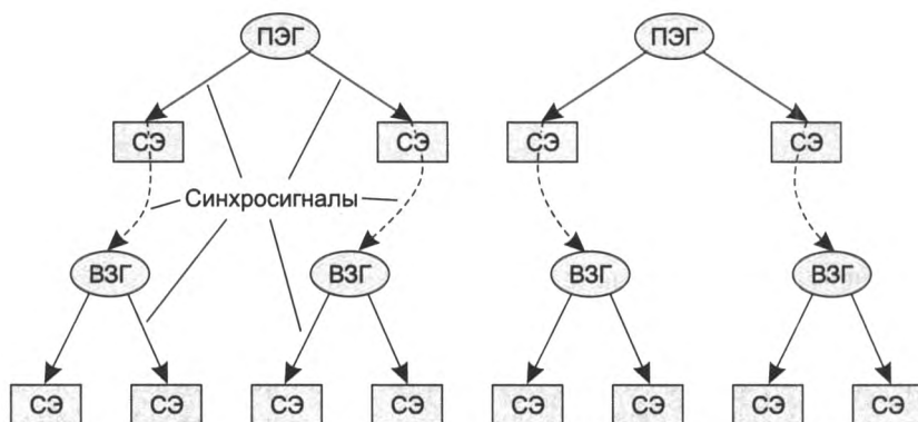
Рис. 8.8. Организация распределения синхросигналов по узлам сети
