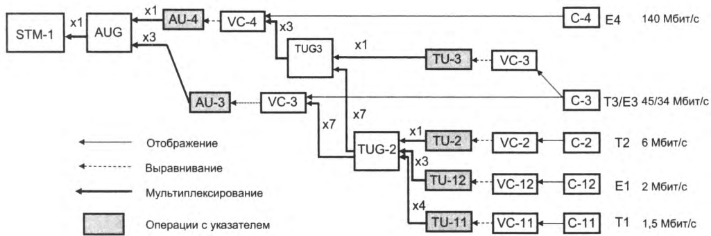
Рис. 8.14. Схема компоновки кадра STM-1 из потоков PDH разной скорости
