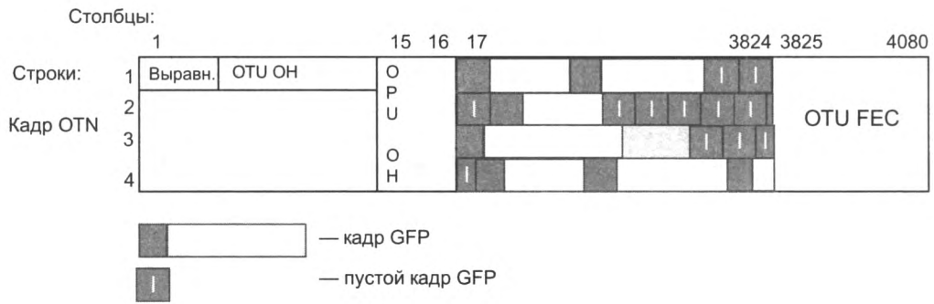
Рис. 9.13. Размещение кадров STM в полях данных кадров OTN
