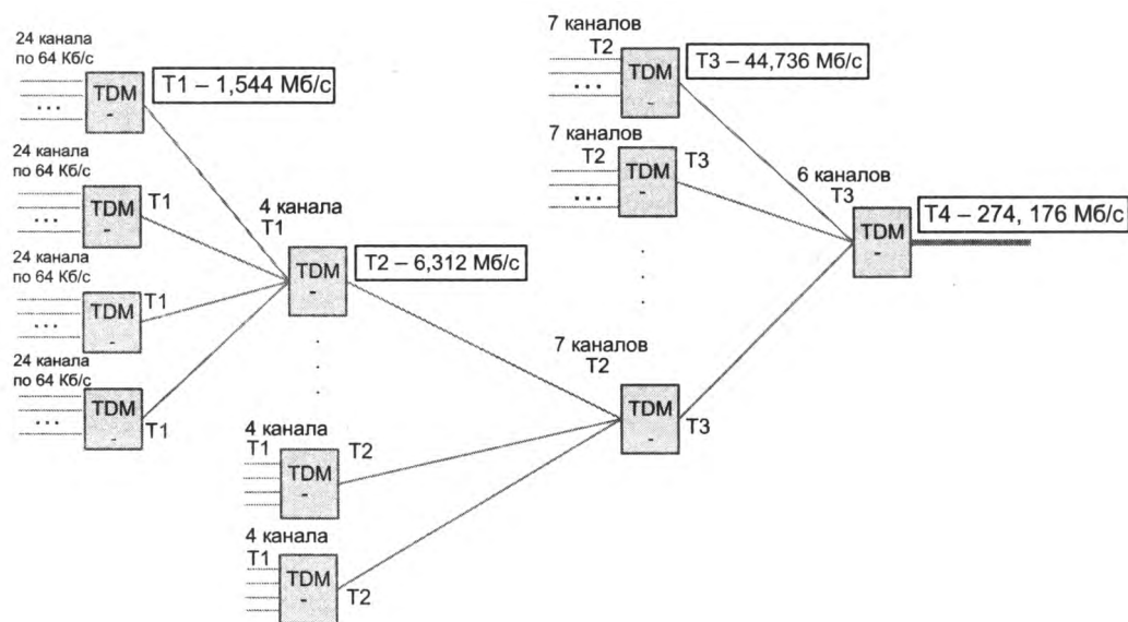
Рис. 8.7. Система Т-каналов
