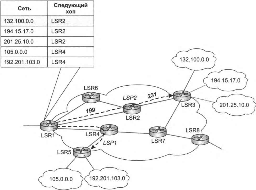
Рис. 20.10. Новый путь LSP2
