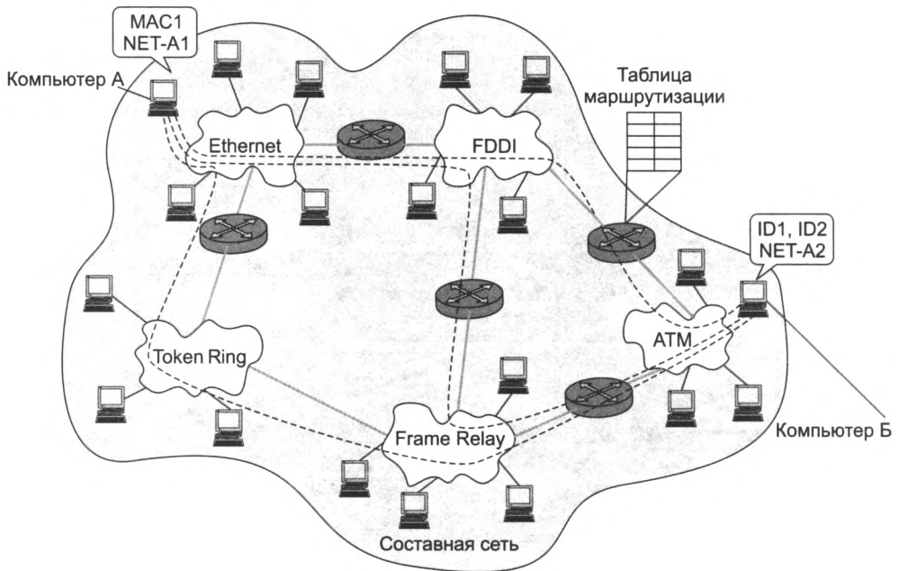
Рис. 4.8. Пример составной сети
