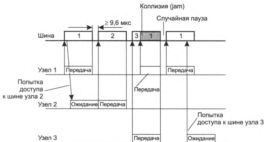
Рис. 10.5. Метод случайного доступа CSMA/CD
