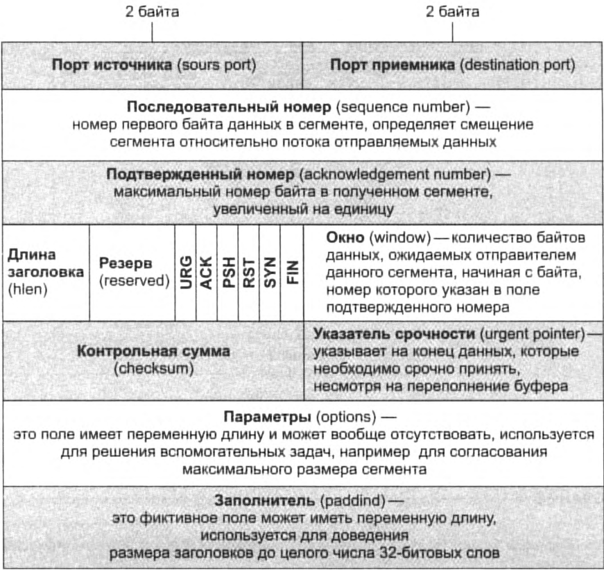
Рис. 15.5. Формат заголовка TCP-сегмента
