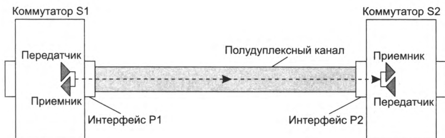
Рис. 2.19. Полудуплексный канал — разделяемая среда
