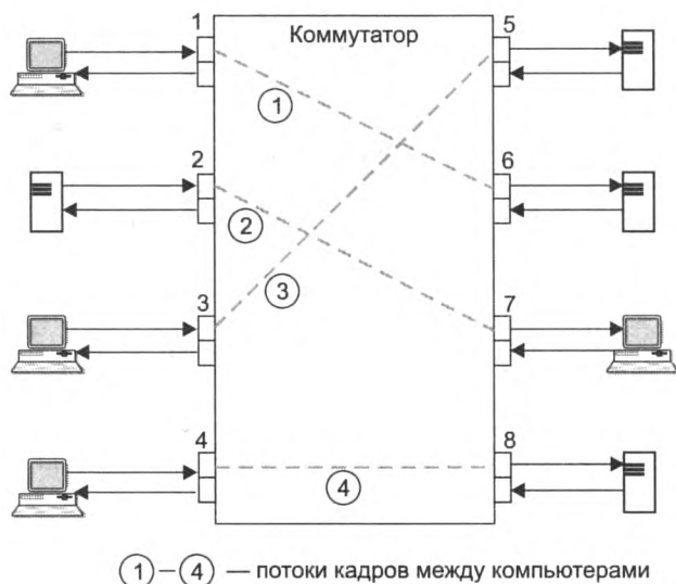
Рис. 10.14. Параллельная передача кадров коммутатором
