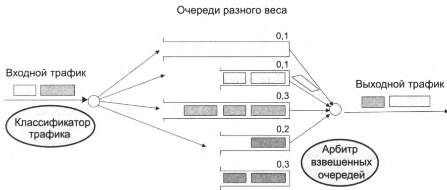
Рис. 5.15. Взвешенные очереди
