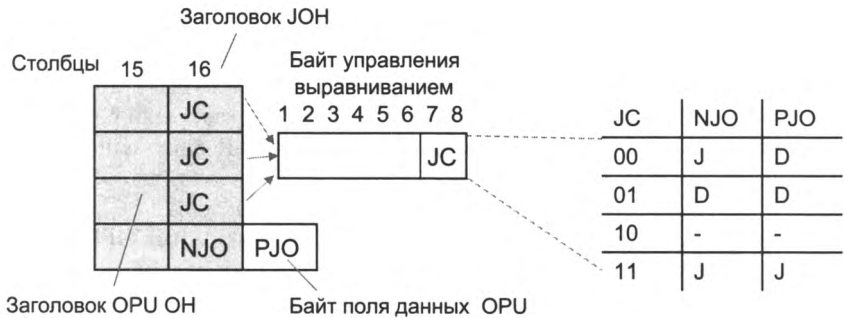
Рис. 9.12. Заголовок выравнивания JON и байты выравнивания NJO и PJO
