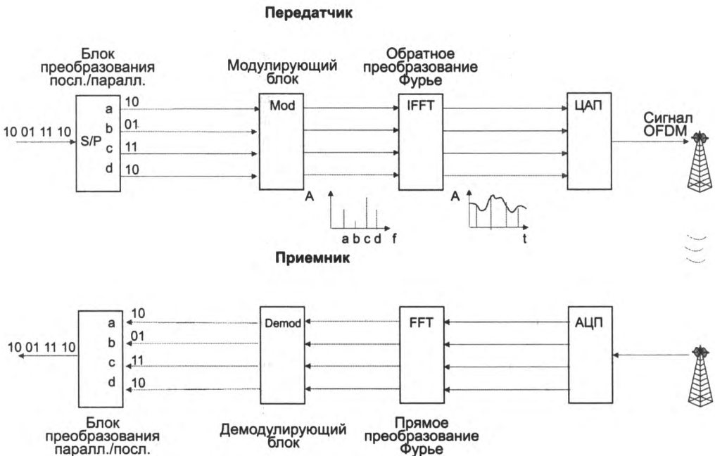
Рис. 21.17. Преобразование сигналов в системе передатчик-приемник OFDM
