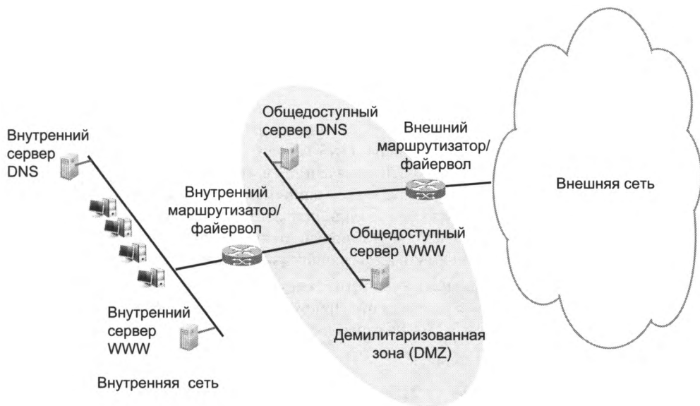
Рис. 28.12. Файервол на базе двух маршрутизаторов
