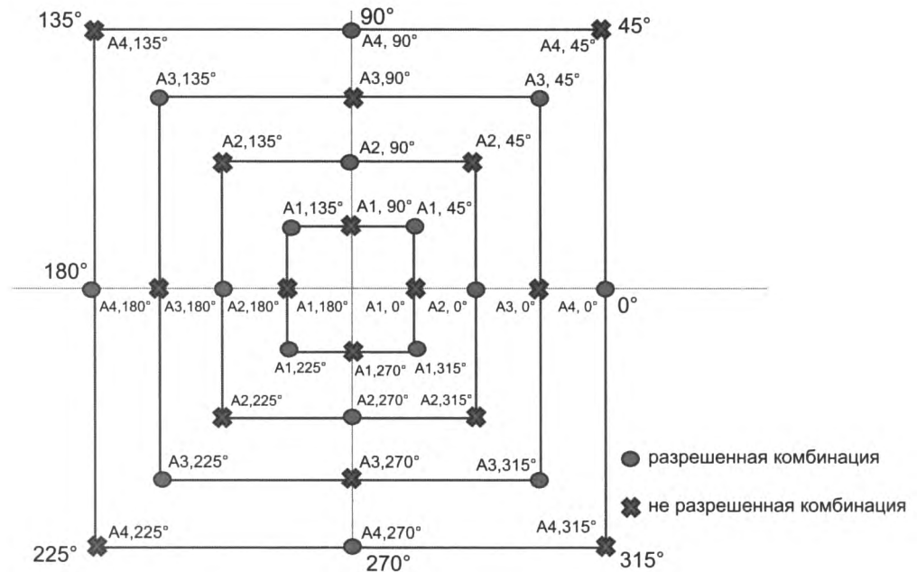
Рис. 7.9. Квадратурная амплитудная модуляция с 16 состояниями сигнала
