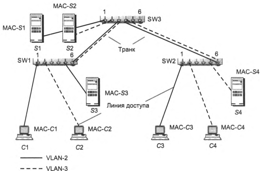
Рис. 11.14. Разбиение сети на две виртуальные локальные сети
