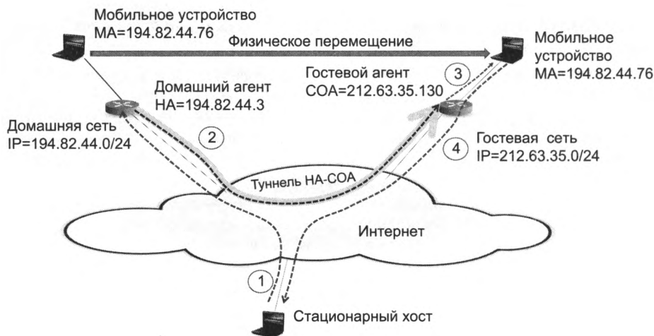
Рис. 23.9. Обмен трафиком через туннель между домашним и внешним агентами
