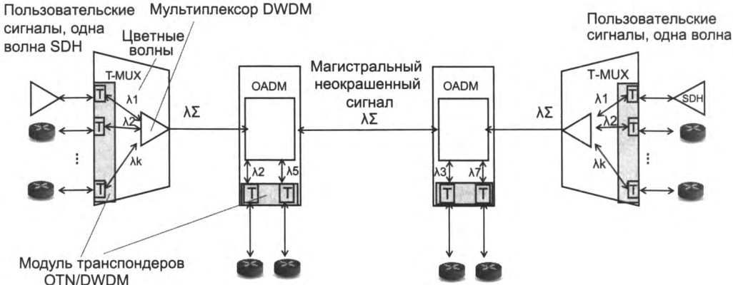
Рис. 9.17. Сеть OTN/DWDM с транспондерами
