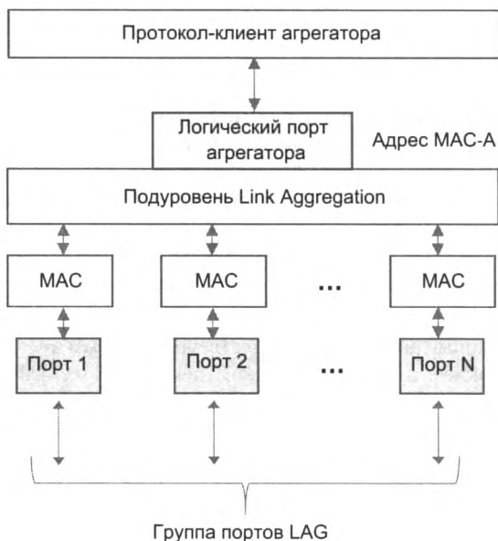
Рис. 11.6. Позиция подуровня агрегирования линий связи в стеке протоколов Ethernet
