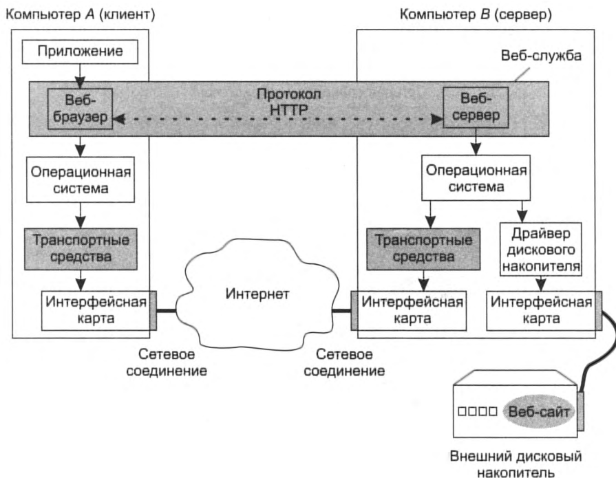
Рис. 2.4. Веб-служба
