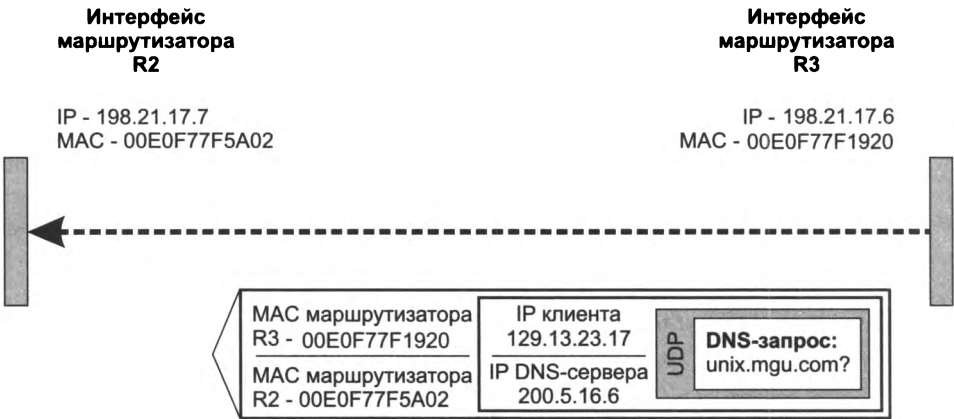
Рис. 14.6. Кадр Ethernet с DNS-запросом, отправленный с маршрутизатора R3 маршрутизатору R2
