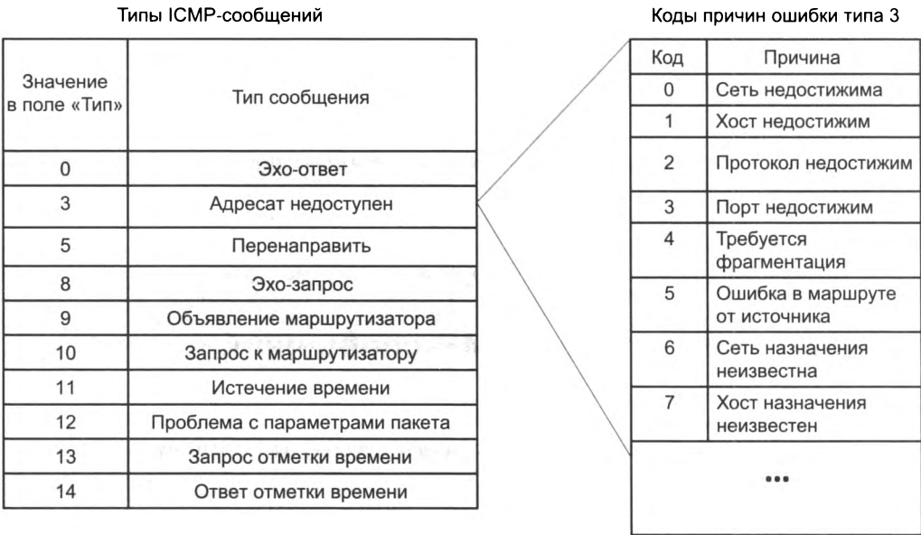
Рис. 14.15. Типы ICMP-сообщений и коды причин ошибки типа 3
