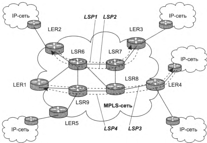
Рис. 20.2. MPLS-сеть
