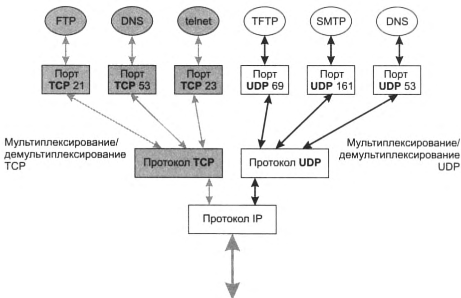
Рис. 15.1. Мультиплеккирование и демультиплеккирование на транспортном уровне
