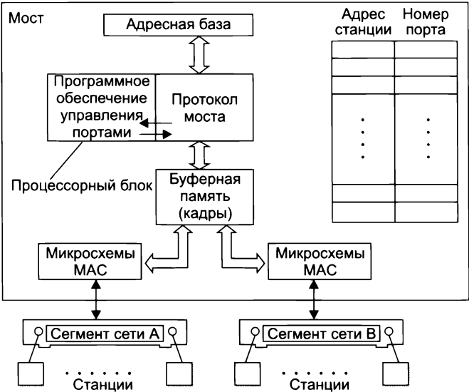
Рис. 10.11. Структура моста/коммутатора
