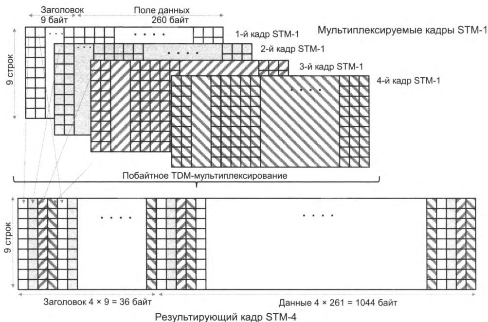
Рис. 8.13. Мультиплексирование четырех кадров STM-1 в кадр STM-4
