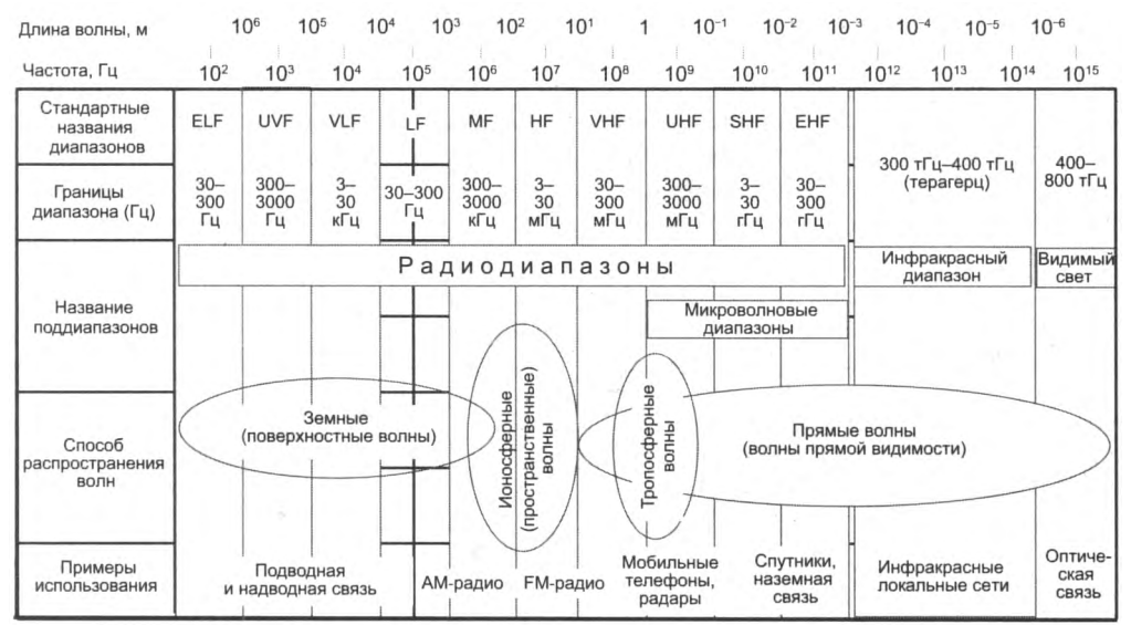
Рис. 21.2. Диапазоны электромагнитного спектра. Стандартные диапазоны частот:
