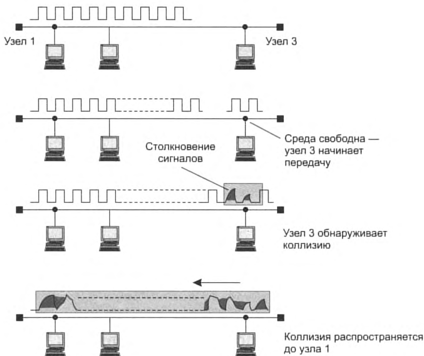
Рис. 10.6. Схема возникновения и распространения коллизии
