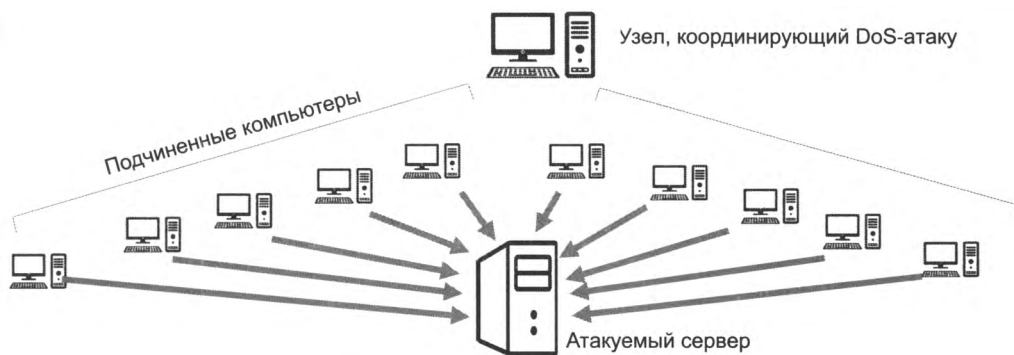
Рис. 26.6. Схема DDoS-атаки
