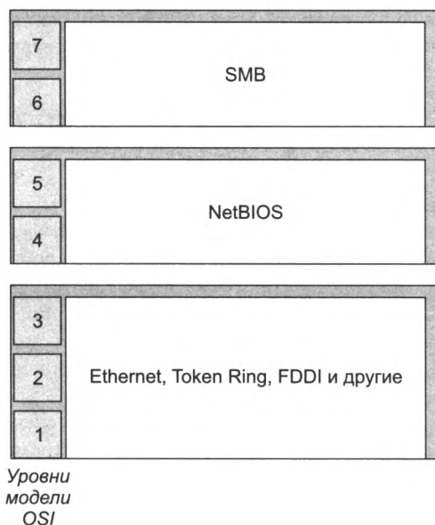
Рис. 4.11. Стек NetBIOS/SMB
