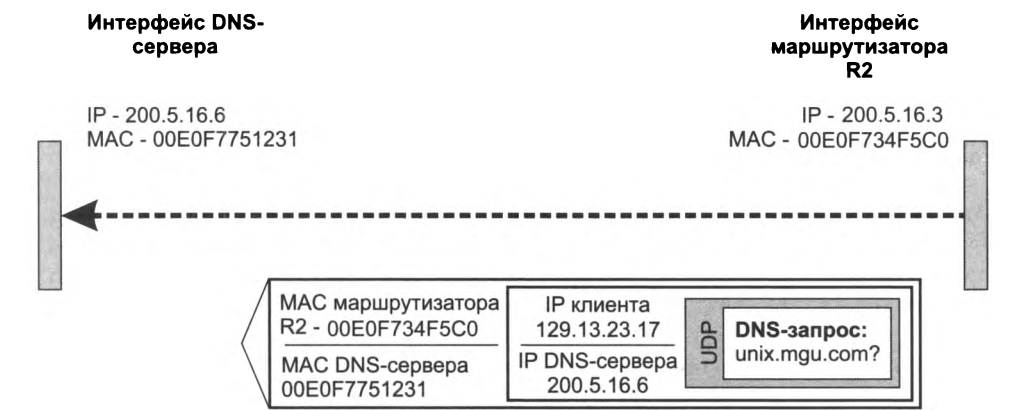
Рис. 14.7. Кадр Ethernet с DNS-запросом, отправленный с маршрутизатора R2
