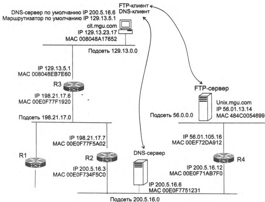
Рис. 14.4. Пример IP-маршрутизации
