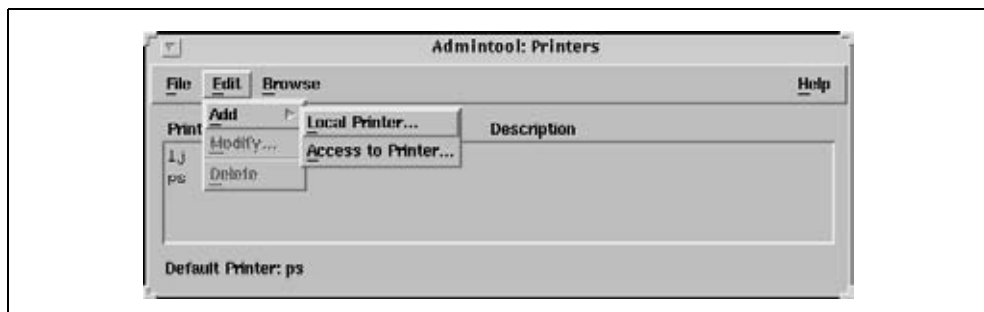
Рис. 9.1. Менеджер печати
