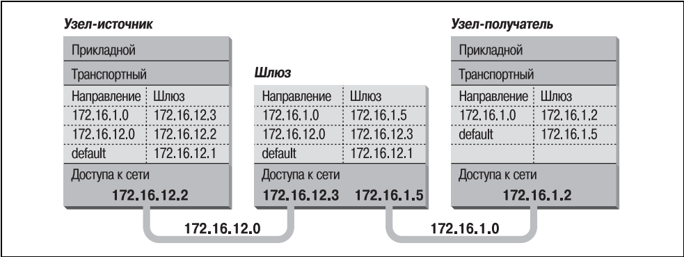
Рис. 2.4. Табличная маршрутизация
