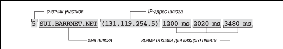
Рис. 13.2. Вывод traceroute
