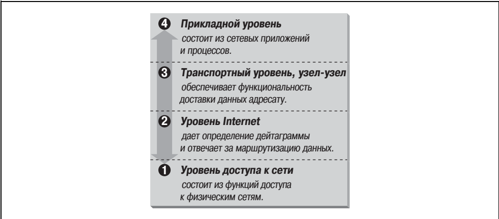
Рис. 1.2. Архитектура TCP/IP
