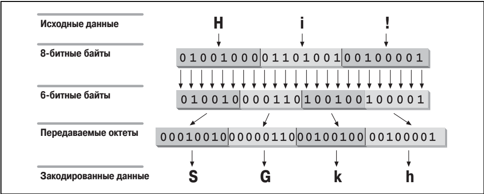
Рис. 3.4. Кодирование base64
