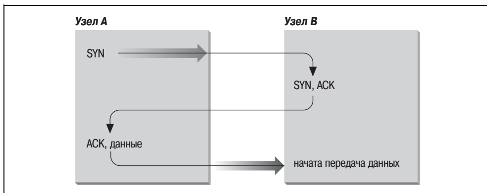
Рис. 1.10. Тройное рукопожатие
