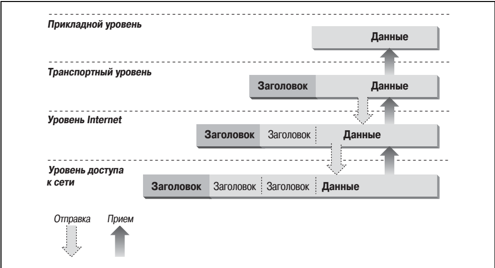
Рис. 1.3. Инкапсуляция данных
