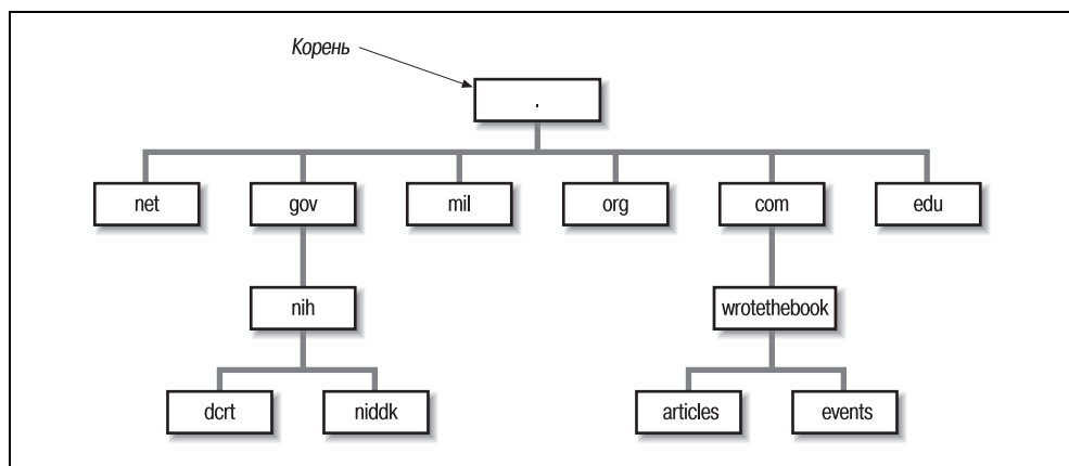
Рис. 3.1. Иерархия доменов
