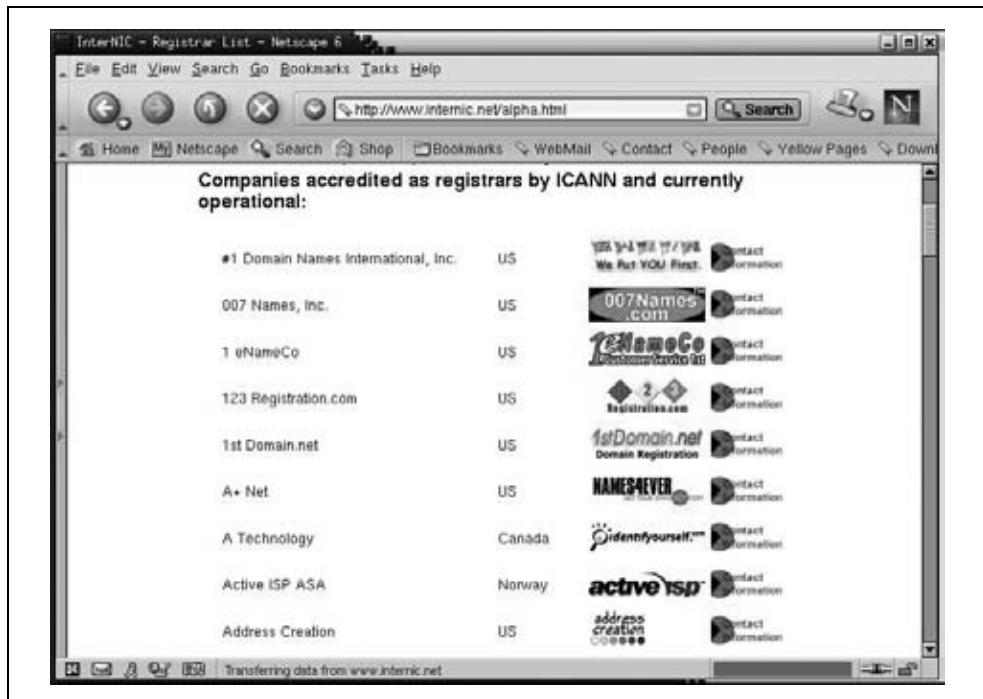
Рис. 4.2. Перечень регистраторов
