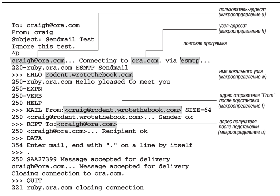
Рис. 10.5. Подробная диагностика
