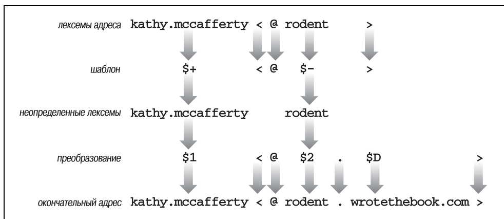
Рис. 10.3. Переписывание адреса
