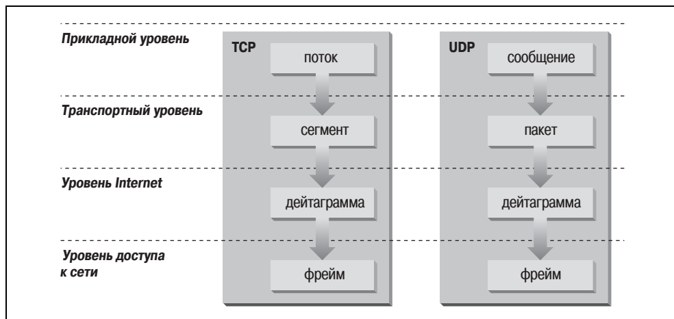
Рис. 1.4. Структуры данных
