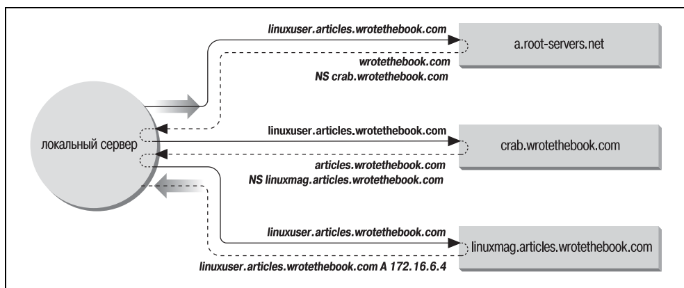
Рис. 3.2. DNS-запрос
