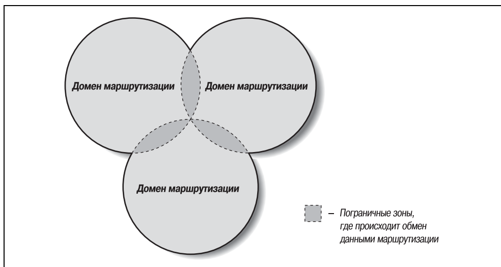
Рис. 2.3. Домены маршрутизации
