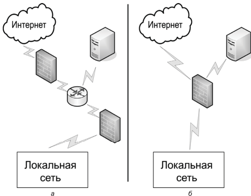
Рис. 5.7. Варианты создания демилитаризованной зоны: а — с использованием двух межсетевых экранов; б — с использованием одного межсетевого экрана
