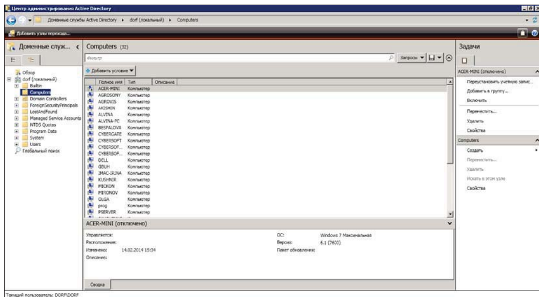
Рис. 6.2. Центр администрирования Active Directory Windows Server 2008: список компьютеров домена
