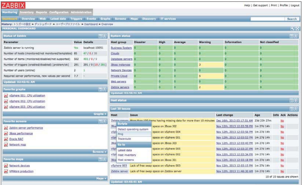
Рис. 7.1. Панель управления Zabbix
