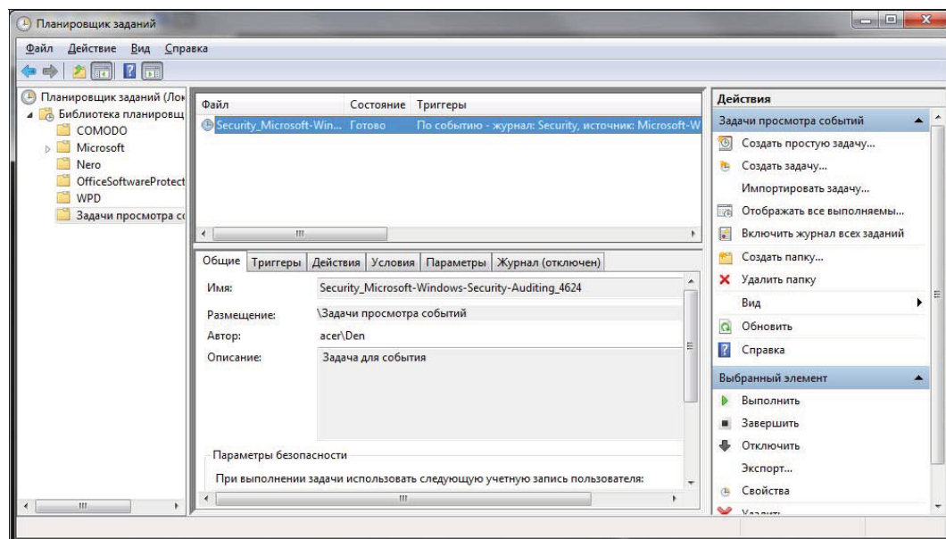
Рис. 7.4. Планировщик заданий Windows 7. Это задание отсылает сообщение по электронной почте на указанный адрес в случае появления нового сообщения в созданном администратором настраиваемом представлении журнала событий
