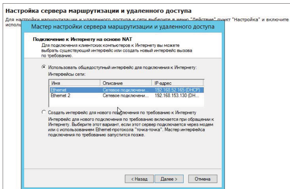
Рис. 5.5. Выбор интерфейса для соединения с Интернетом
