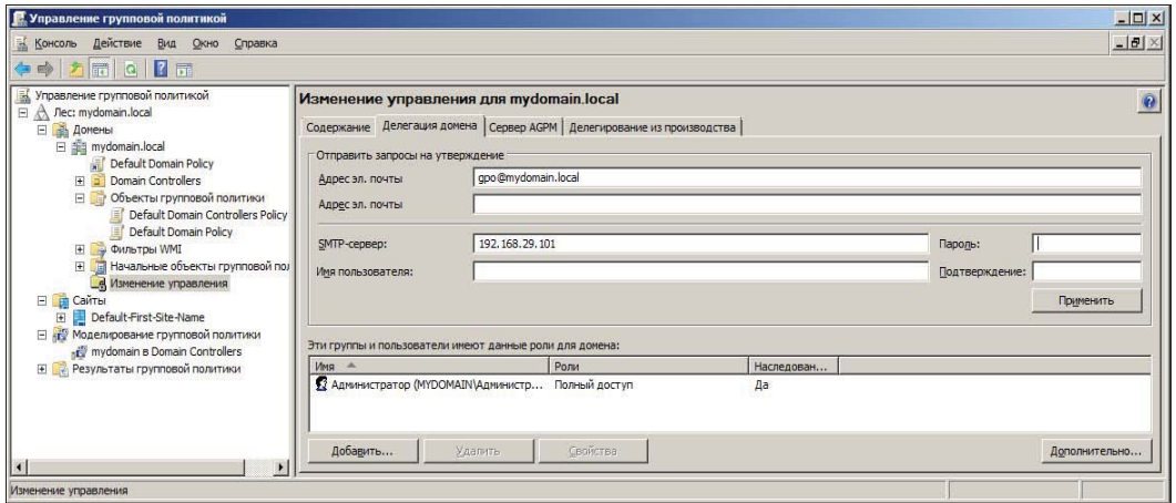
Рис. 6.8. Назначения прав администраторам по управлению групповыми политиками
