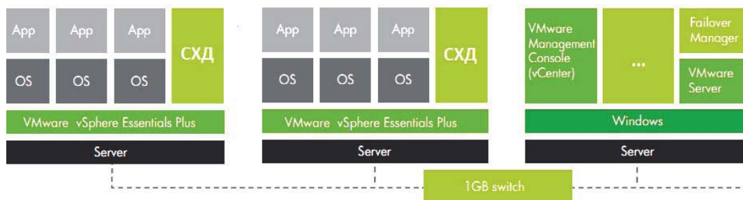
Рис. 8.2. Вариант логической структуры решения на продуктах компании VMware
