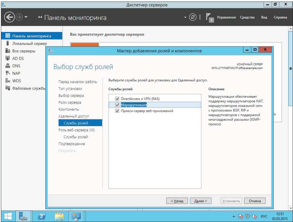
Рис. 5.2. Установка службы ролей
