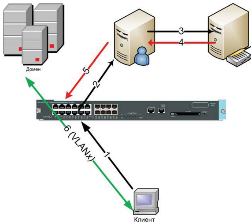
Рис. 9.3. Последовательность подключения клиента по протоколу 802.1x
