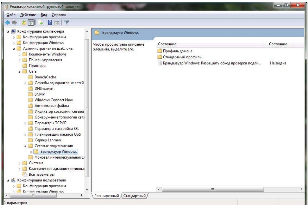
Рис. 5.11. Настройка параметров брандмауэра Windows при помощи групповых политик
