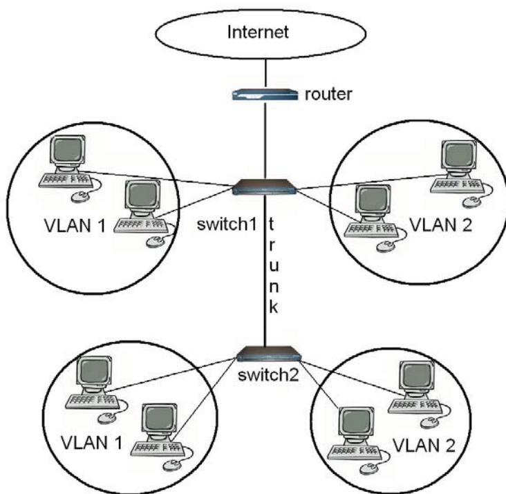
Рис. 8.8. Конфигурация виртуальной локальной сети с доступом к Интернету
