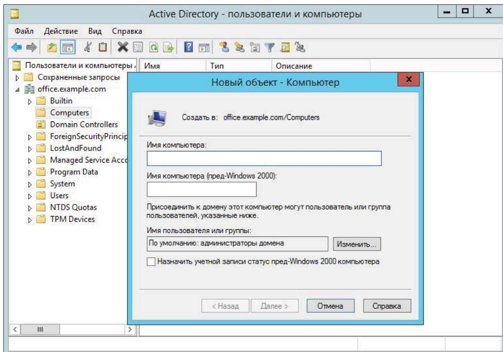
Рис. 4.2. Создание объекта компьютер с делегированием его подключения к домену
