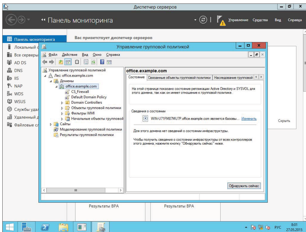
Рис. 6.4. Оснастка Управление групповой политикой (Windows Server 2012)
