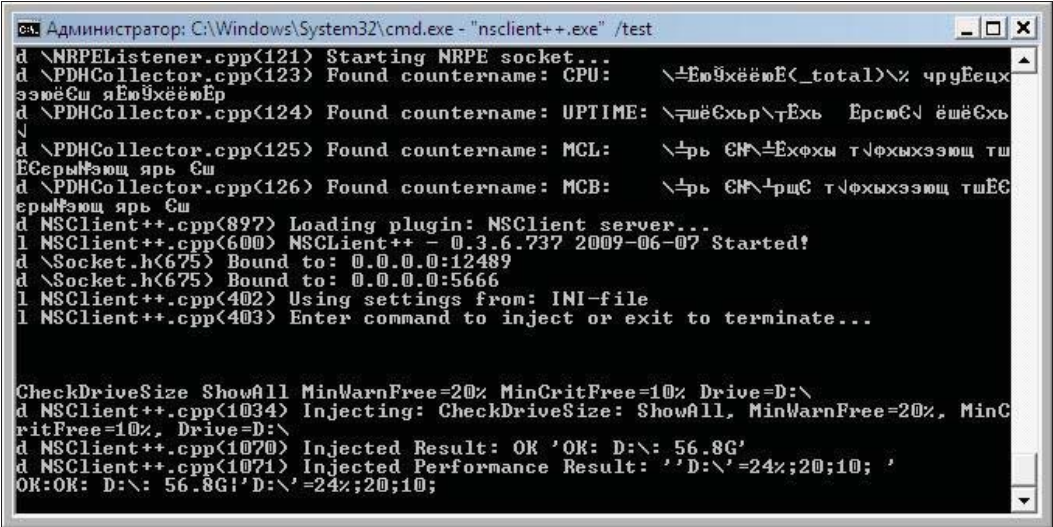
Рис. 7.8. Окно программы NSClient++ в диагностическом режиме
