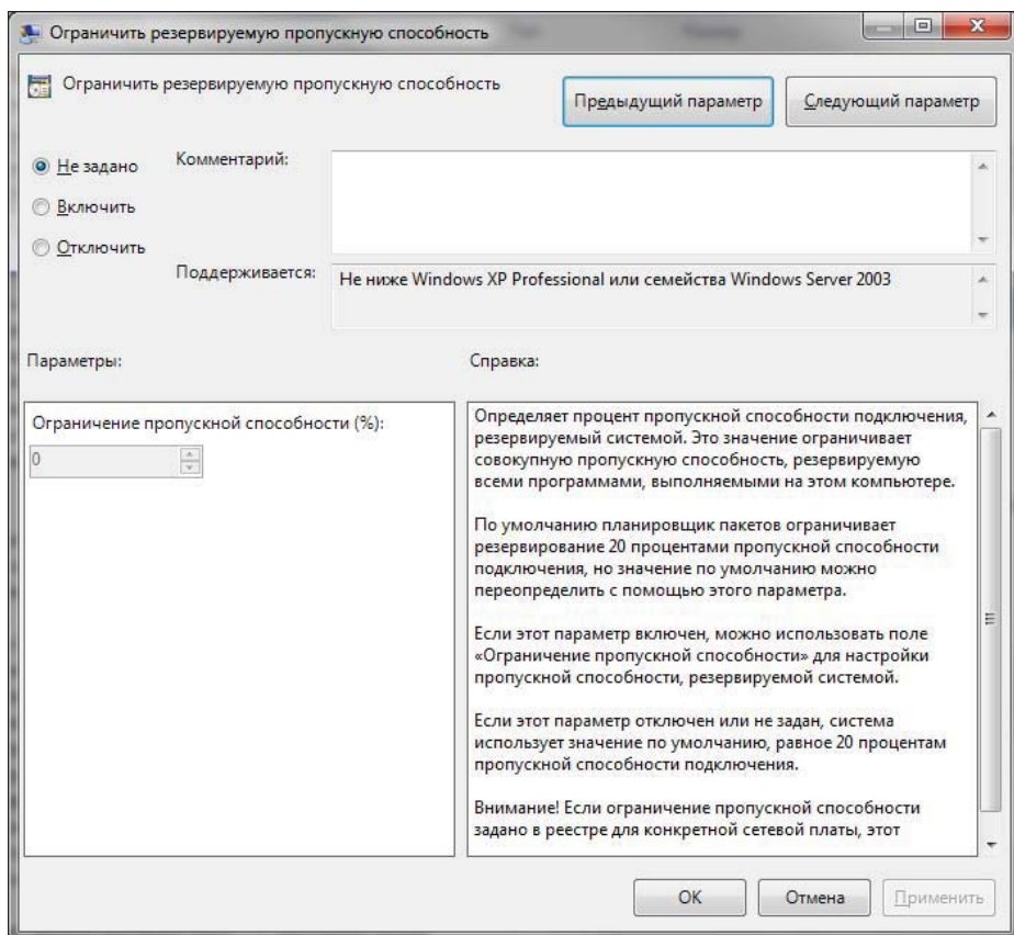
Рис. 3.7. Настройка резервируемой пропускной способности
