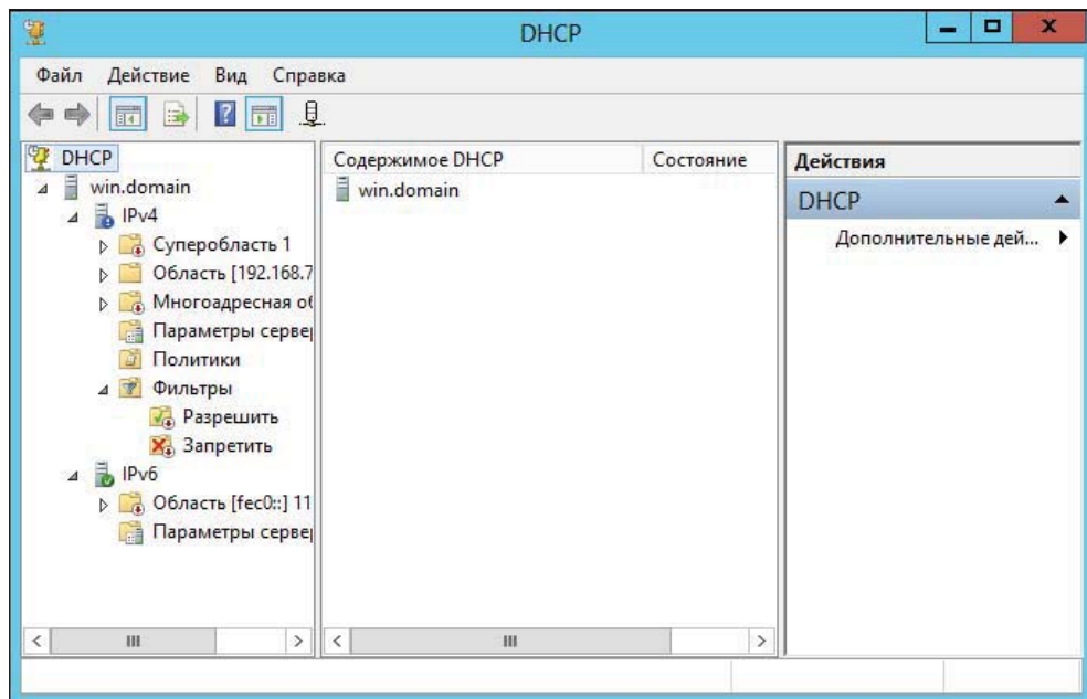
Рис. 3.17. Консоль управления DHCP в Windows Server 2012 R2
