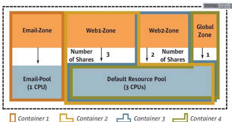
Рис. 8.1. Пример разбиения Solaris-сервера на зоны
