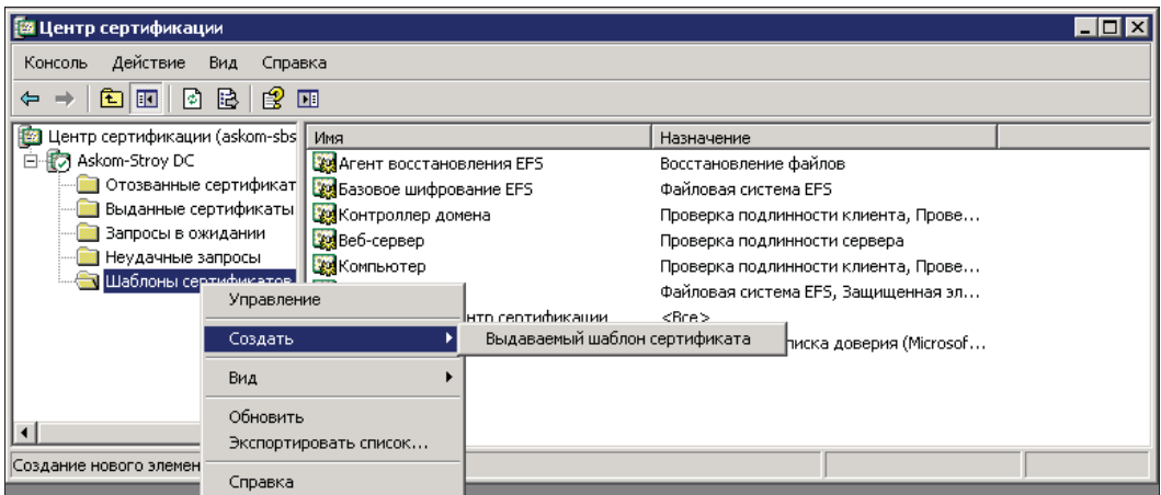
Рис. 9.4. Публикация шаблона сертификата RADIUS-сервера. Для использования в протоколе 802.1x аутентификации на основе сертификатов сервер IAS должен получить специальный сертификат, который по умолчанию не опубликован в Центре сертификации
