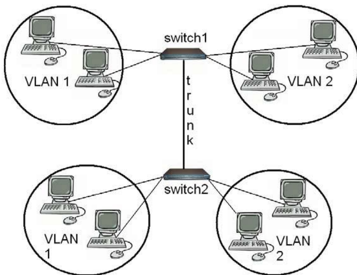
Рис. 8.7. Усовершенствованная топология сети Cisco
