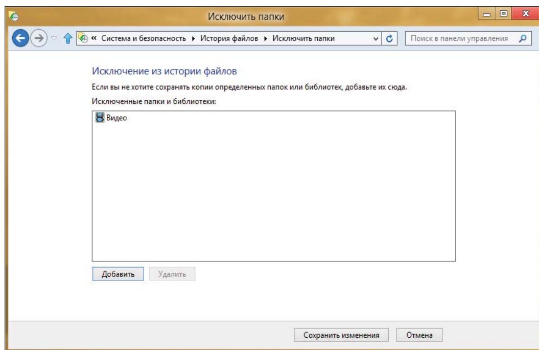
Рис. 11.32. Список исключений
