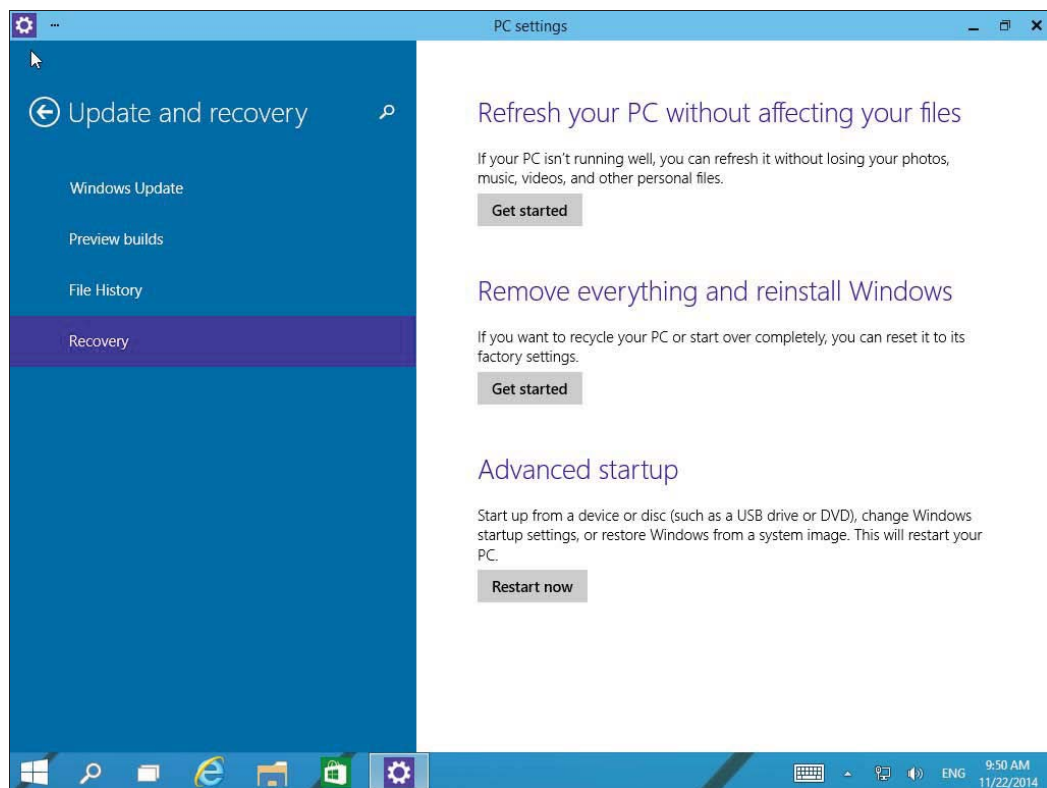
Рис. 11.20. Раздел Recovery
