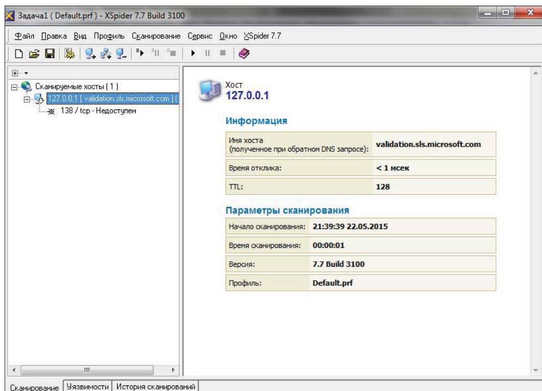
Рис. 9.6. Программа XSpider
