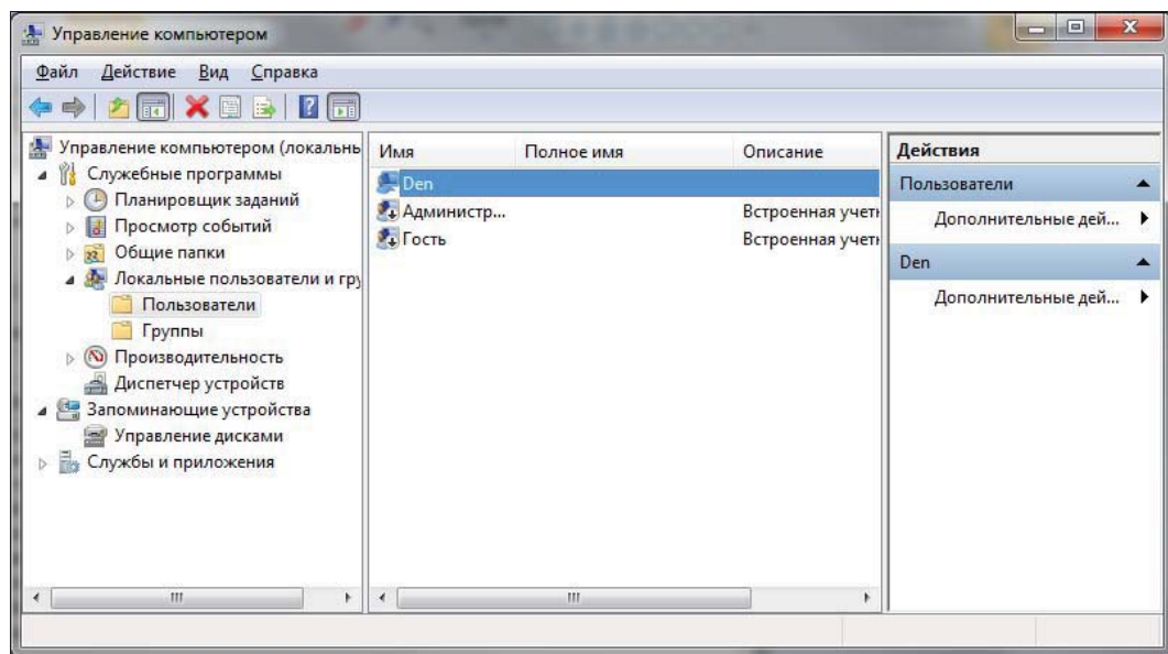
Рис. 4.11. Локальные пользователи
