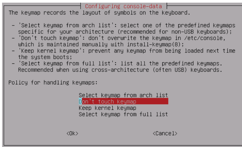
Рис. 6.18. Выбор раскладки
