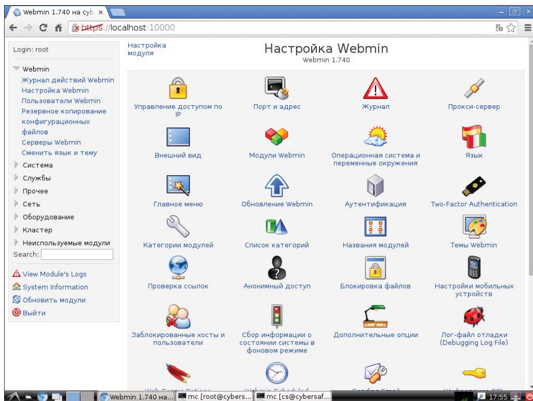
Рис. 2.9. Веб-интерфейс Webmin
