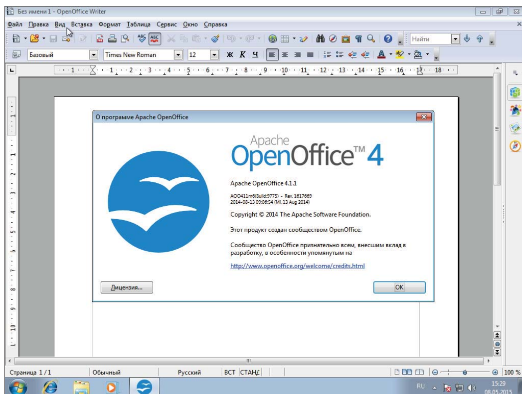
Рис. 2.6. Интерфейс OpenOffice
