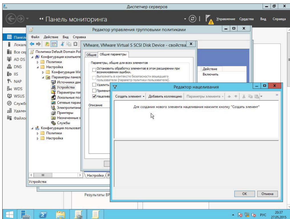
Рис. 6.9. Редактор нацеливания
