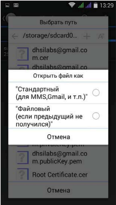
Рис. 9.31. Выберите Стандартный
