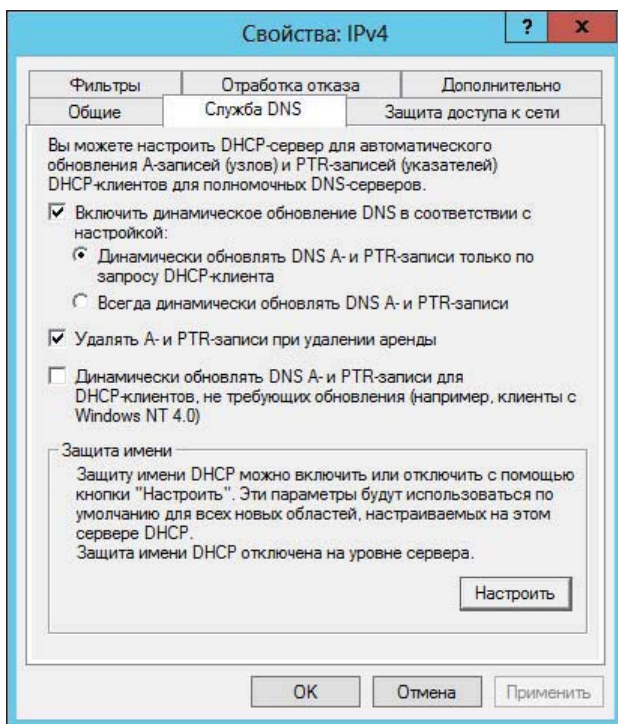
Рис. 3.19. Свойства IPv4 в оснастке DHCP
