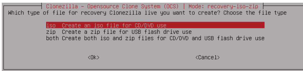
Рис. 6.25. Выбор режима команды recovery-iso-zip
