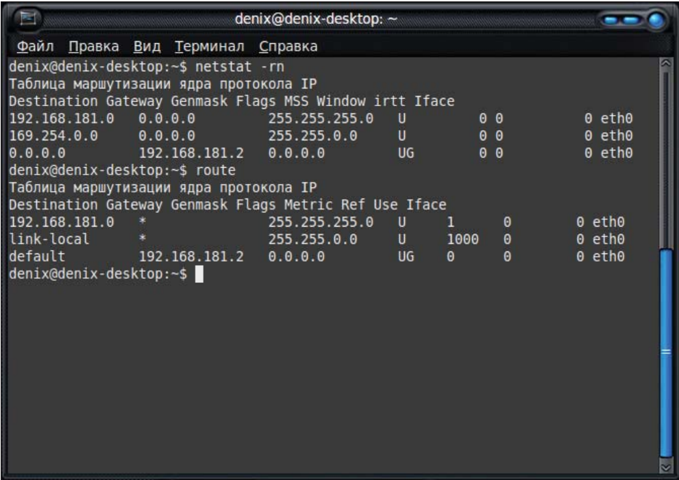
Рис. 3.14. Команды netstat -rn и route
