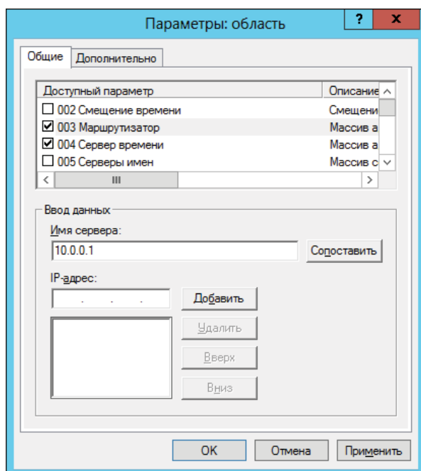
Рис. 3.18. Изменение опций области (Windows Server 2012 R2)
