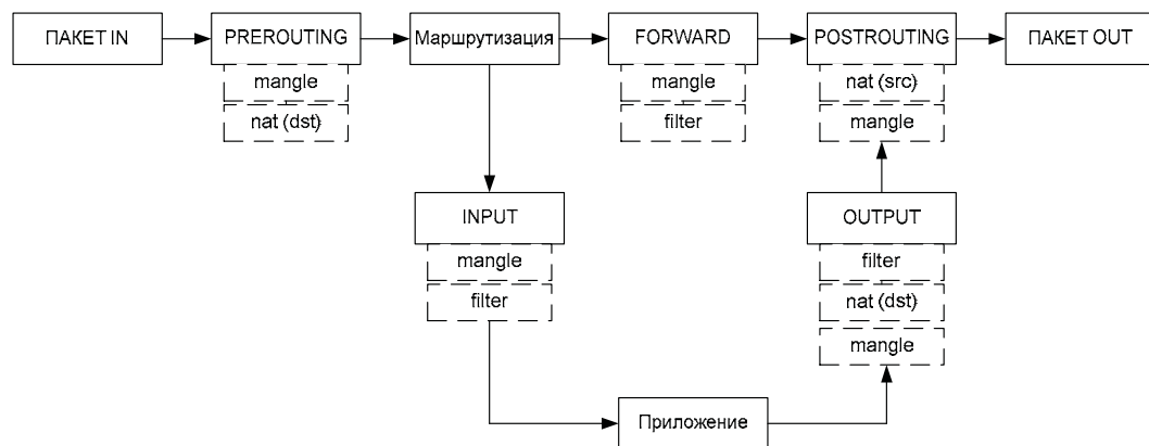
Рис. 5.12. Схема обработки пакета
