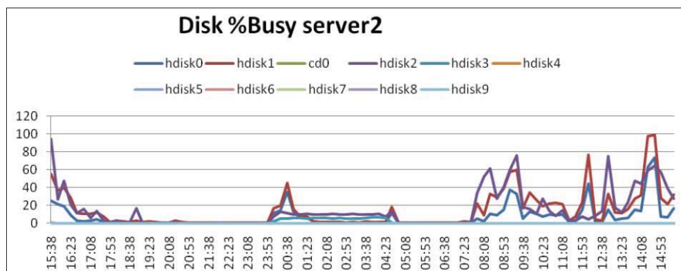
Рис. 11.38. Один из графиков отчета по данным мониторинга AIX-системы программой pmon
