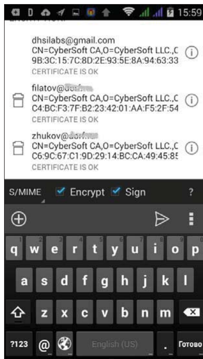
Рис. 9.35. Сертификаты
