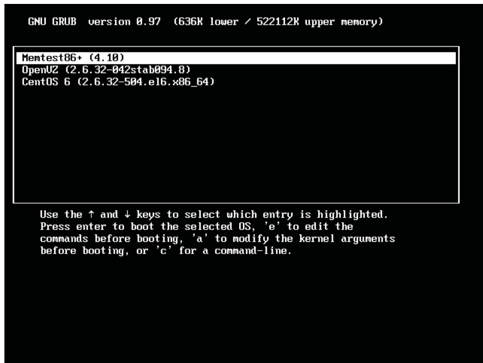
Рис. 11.10. Загрузчик Linux
