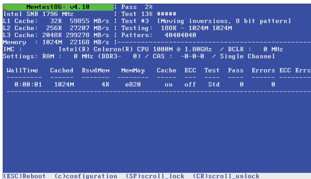
Рис. 11.11. Программа memtest86+
