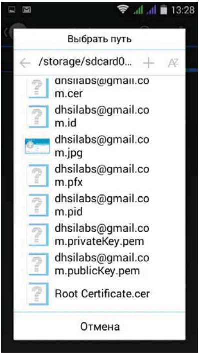
Рис. 9.30. Выбор сертификата
