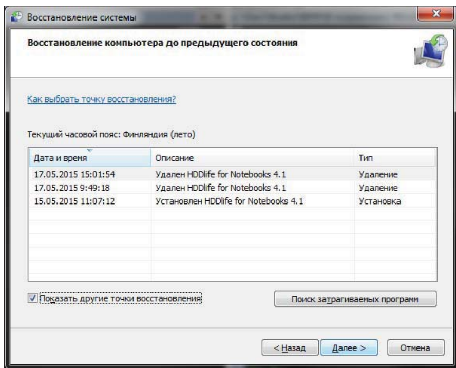
Рис. 11.24. Восстановление системы
