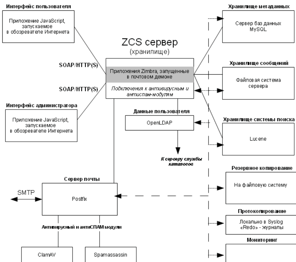
Рис. 2.7. Архитектура ZCS
