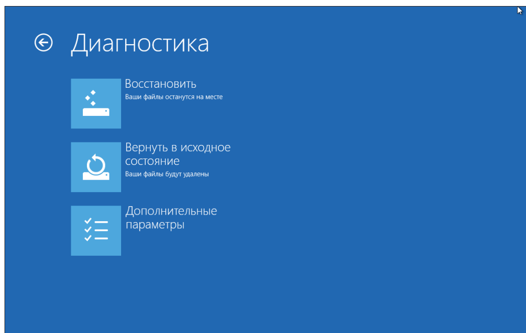
Рис. 11.15. Меню Диагностики
