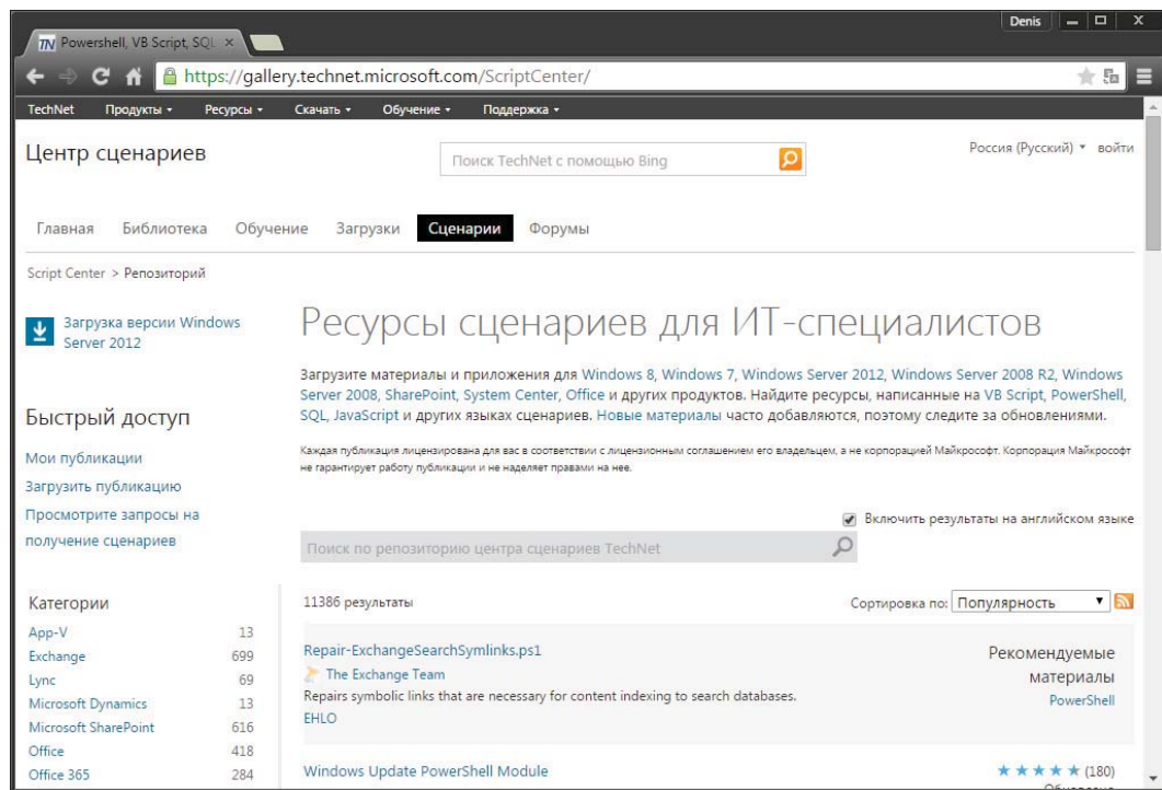
Рис. 6.11. Центр сценариев
