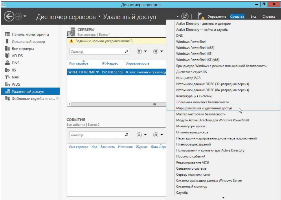
Рис. 5.3. Диспетчер серверов
