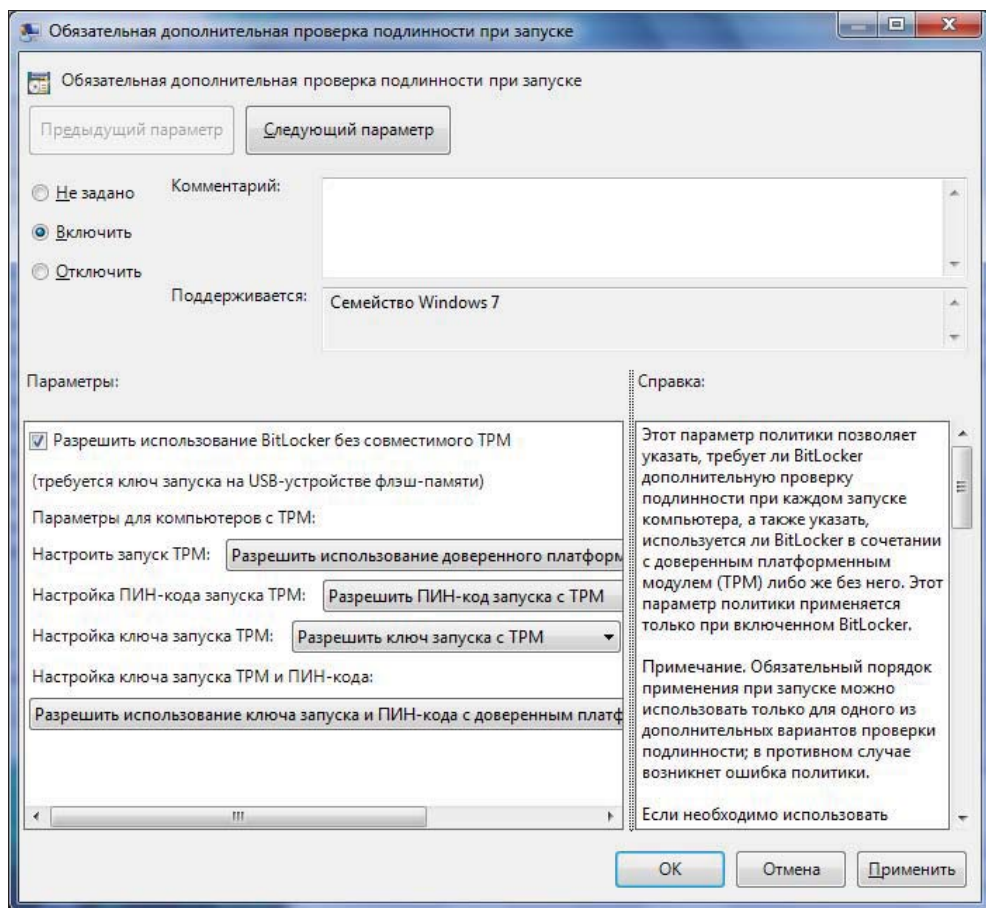
Рис. 9.20. Настройка параметров для включения BitLocker на компьютерах без TPM
