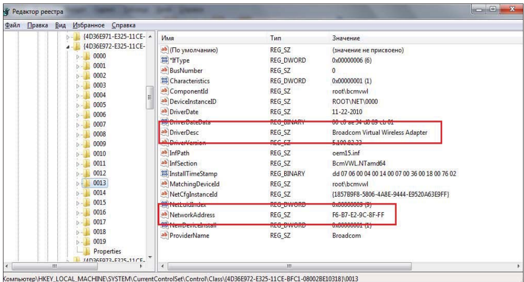
Рис. 3.15. Изменение MAC-адреса сетевого адаптера с помощью реестра
