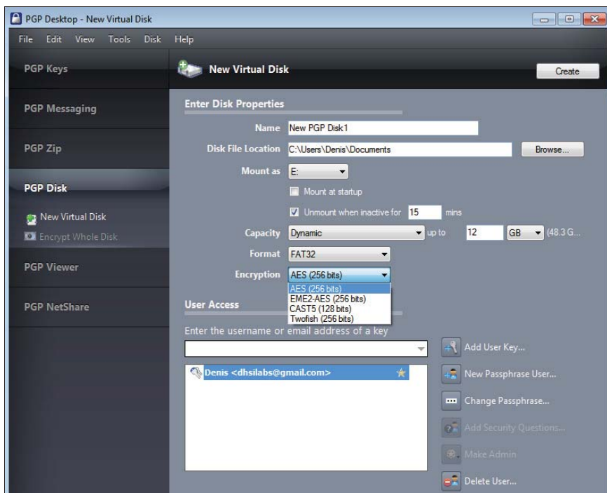
Рис. 9.16. Для создания зашифрованного диска в программе PGP достаточно определить только несколько параметров
