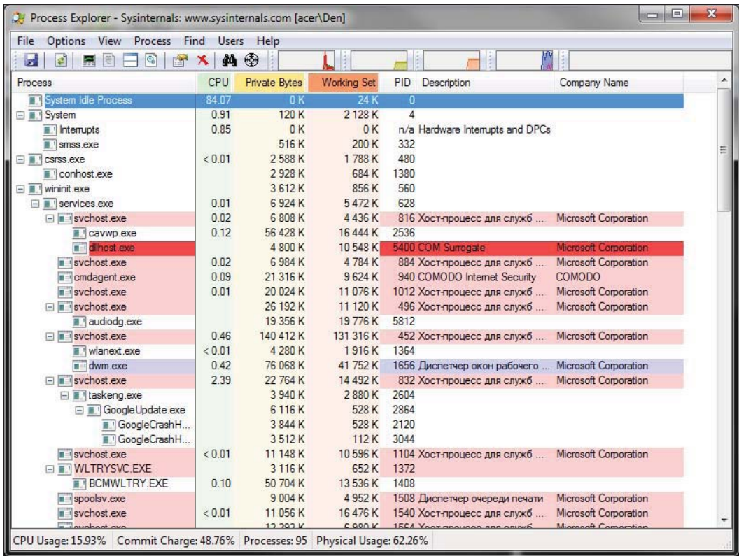
Рис. 9.12. Программа Process Explorer позволяет увидеть иерархию запущенных в системе процессов
