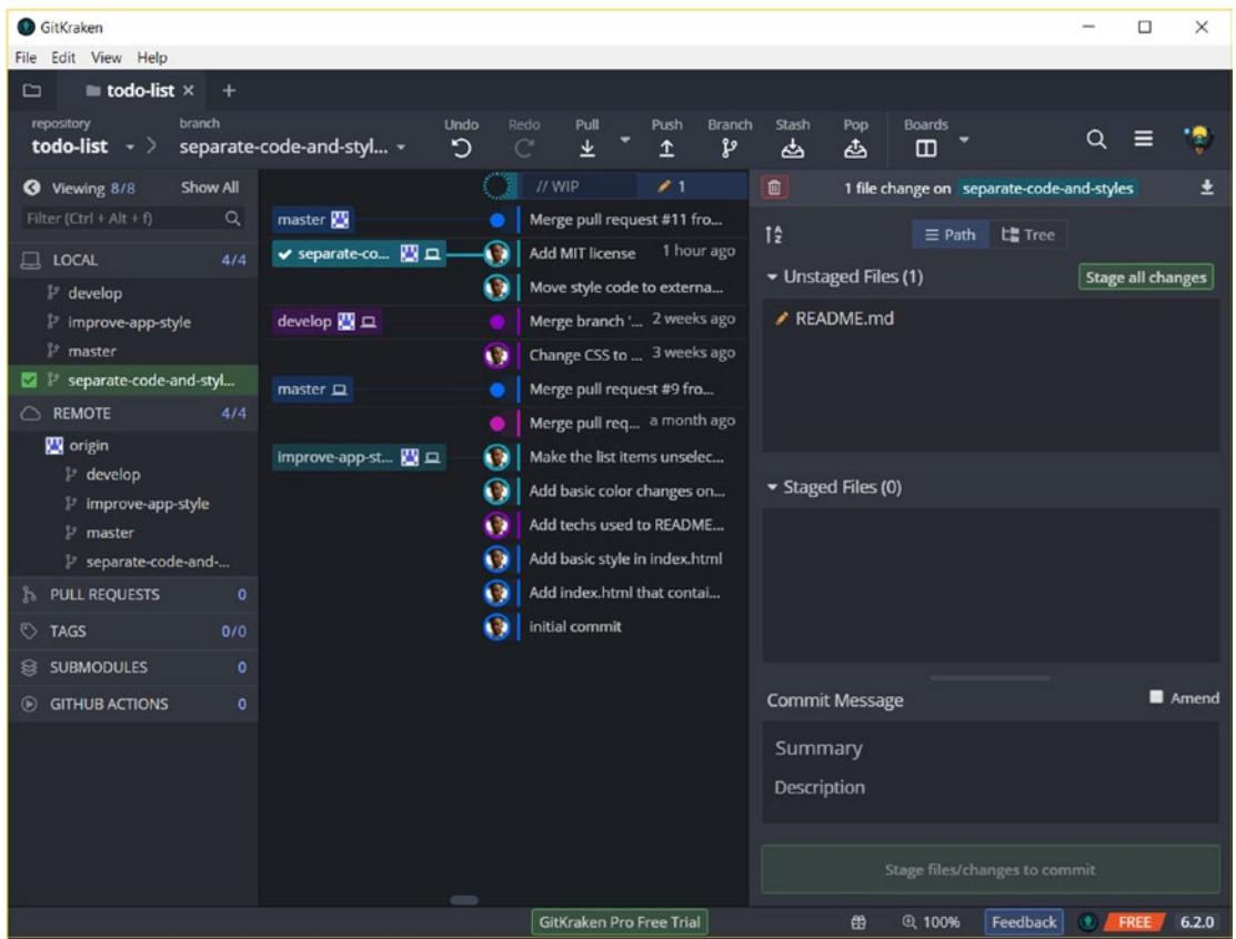
Figure 15-15. GitKraken overview
