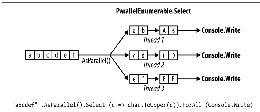
Figure 23-3. PLINQ ForAll
