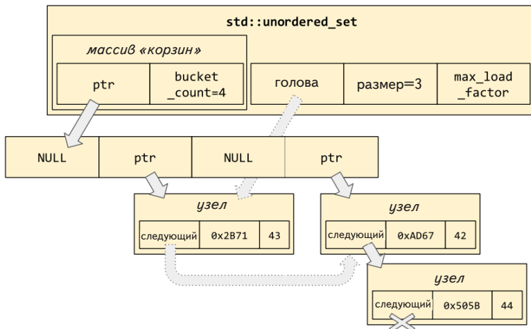
Рис. 4.10. Организация контейнера std::unordered_set в памяти
