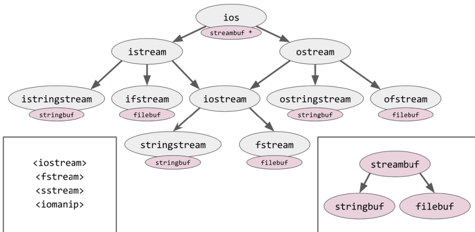
Рис. 9.1. Иерархия классов потоков и stringstream в C++17
