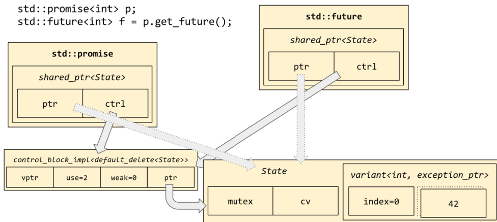
Рис. 7.1. Схематическое представление типов promise и future
