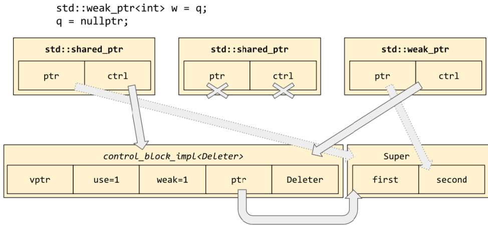
Рис. 6.5. Создание невладеющей ссылки и обнуление второго владеющего указателя shared_ptr
