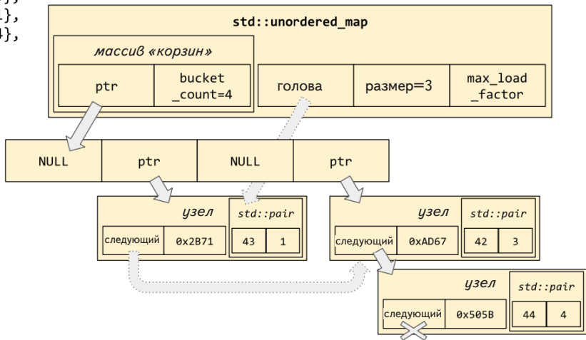
Рис. 4.11. Организация контейнера std::unordered_map в памяти
