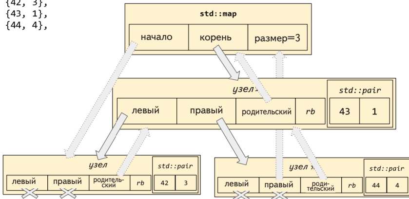
Рис. 4.8. Организация контейнера std::map в памяти
