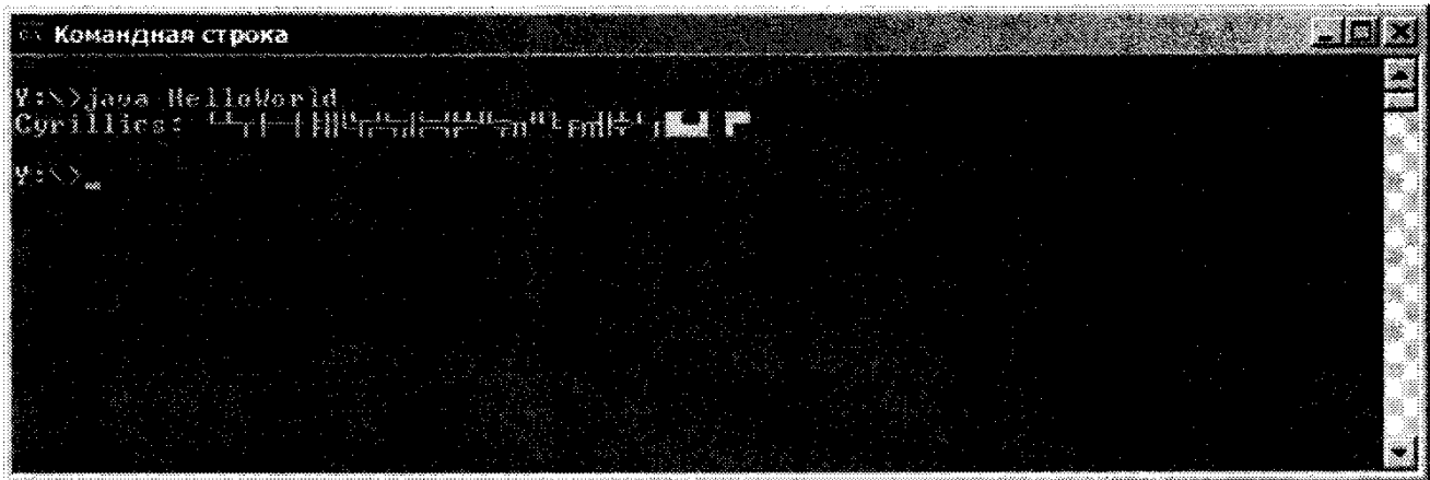
Рис. 6.3. Некорректный вывод русских символов
