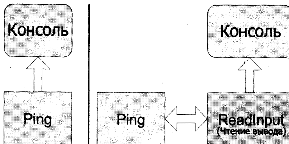
Рис. 6.1. Структура программы для чтения данных внешнего приложения
