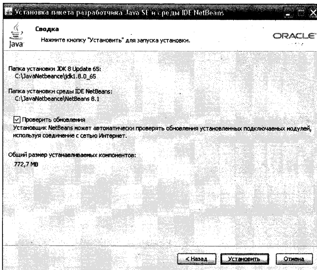
Рис. 2.4. Установка JDK и NetBeans (шаг 3)
