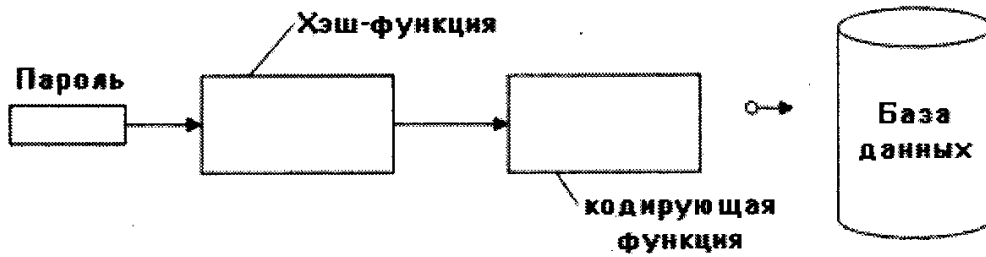
Рис. 6.7. Обычная схема для сохранения хэш-ключа в базу данных
