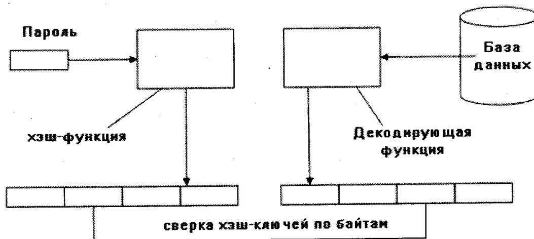
Рис. 6.8. Схема сверки хэш-ключей паролей
