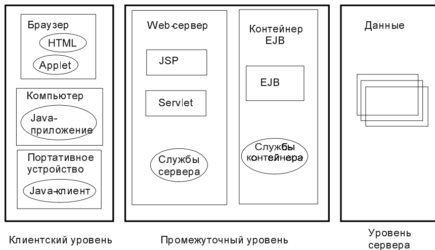
Рис. 5.3. Детализированная модель многоуровневой архитектуры
