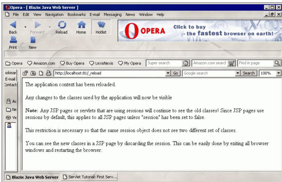
Рис. 4.1. Перезагрузка всех сконфигурированных сервлетов, загрузка классов
