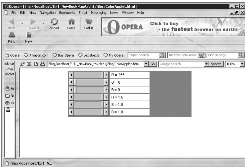
Рис. 1.13. Изменение цвета
