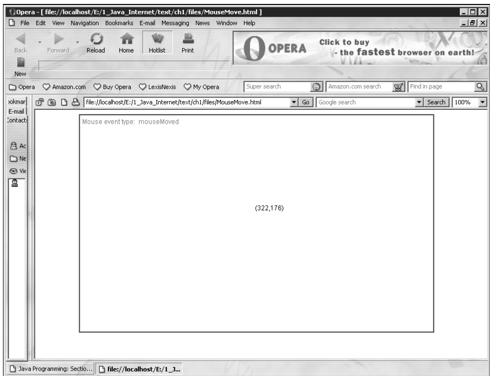
Рис. 1.19. Движение мыши
