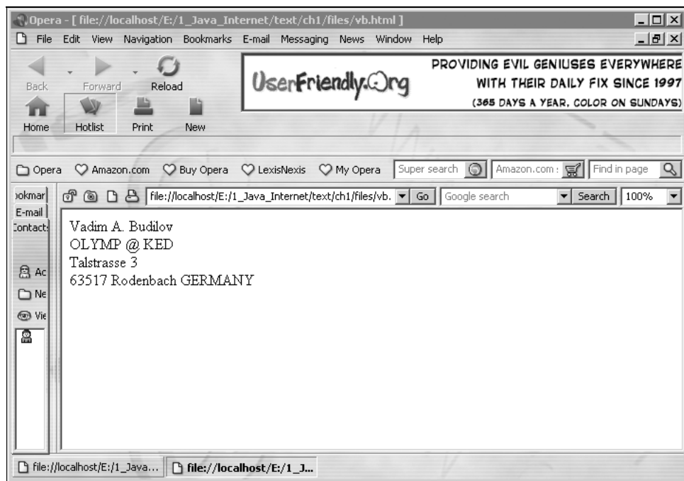
Рис. 1.8. Перенос строки
