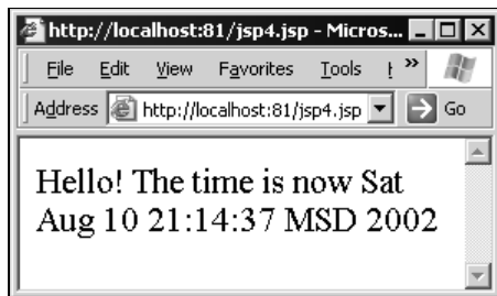
Рис. 3.6. Выведенное HTML-сообщение
