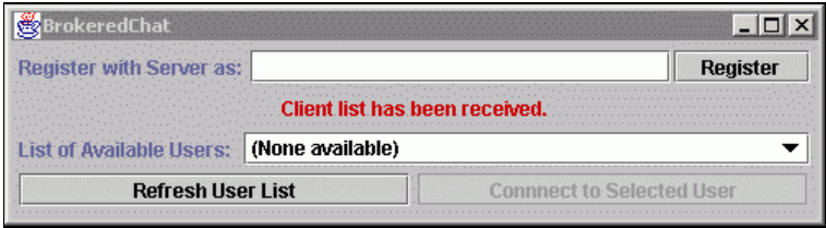
Рис. 2.11. Сервер найден
