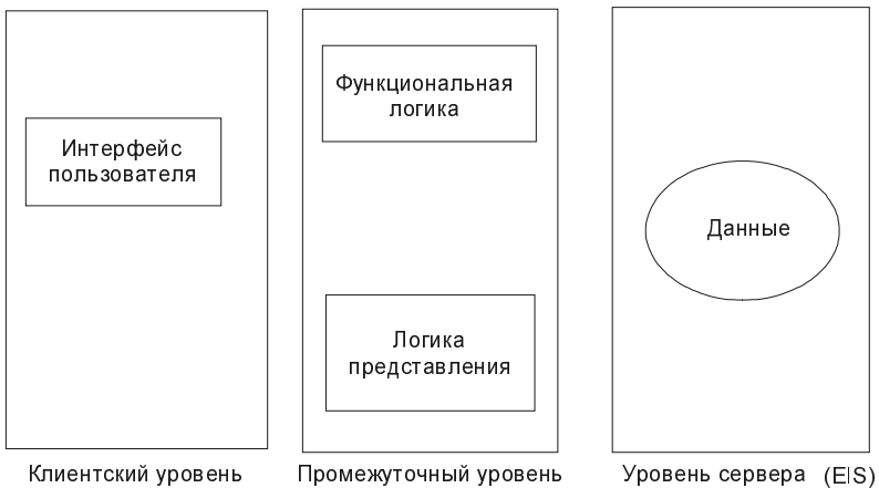
Рис. 5.2. Многоуровневая архитектура
