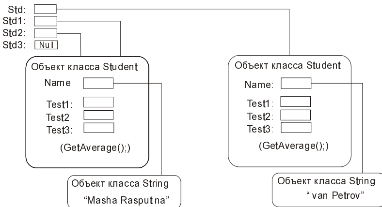
Рис. П4.6. Схема памяти компьютера
