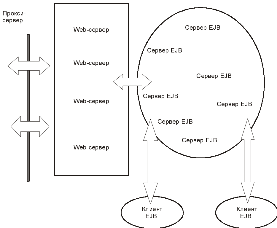
Рис. 3.15. Архитектура сервера Blazix
