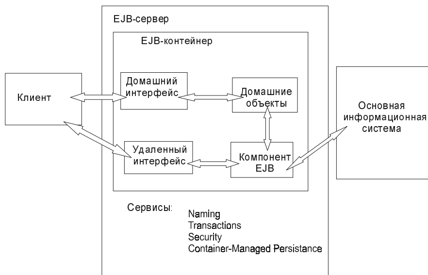
Рис. 5.4. Архитектура приложения, использующего серверные компоненты EJB
