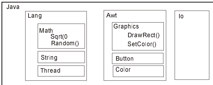
Рис. П4.5. Структура пакета Java
