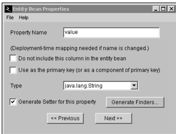
Рис. 5.13. Задание значений параметров для столбца value
