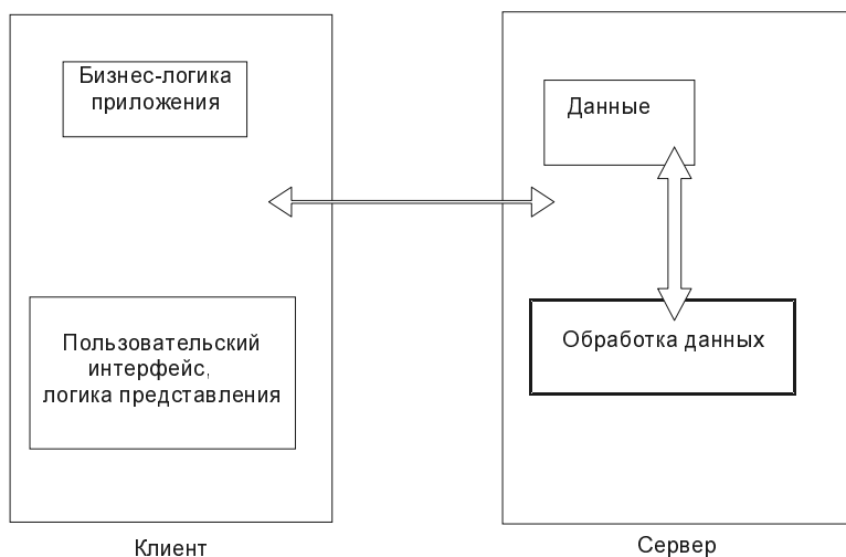
Рис. 5.1. Архитектура клиент-сервер
