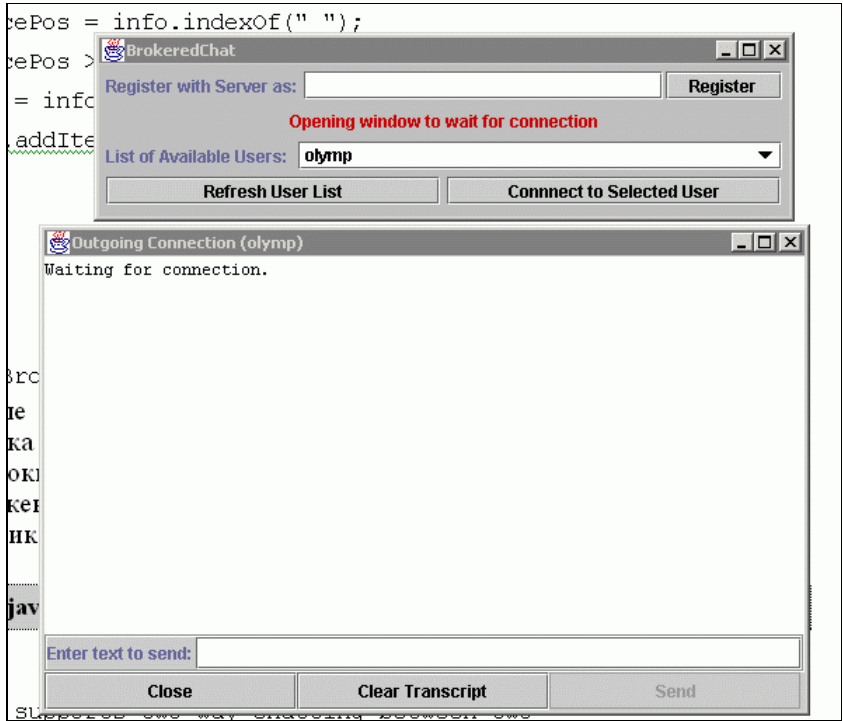
Рис. 2.12. Регистрация пользователя
