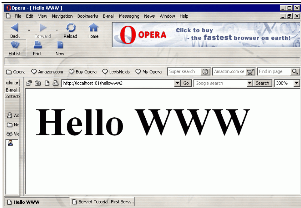
Рис. 4.5. Сервлет HelloWWW2
