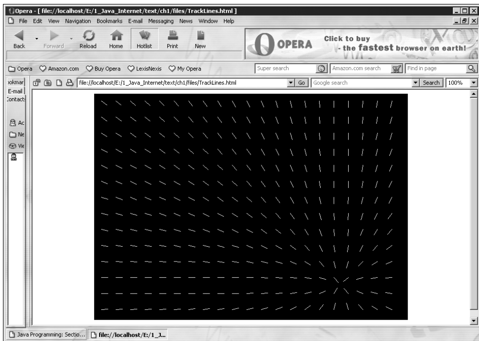
Рис. 1.22. Вращающиеся отрезки
