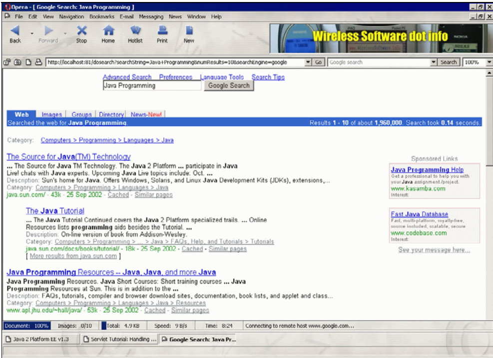
Рис. 4.18. Запрос выполнен
