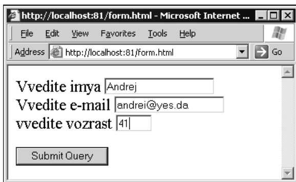
Рис. 3.13. Заполнение формы
