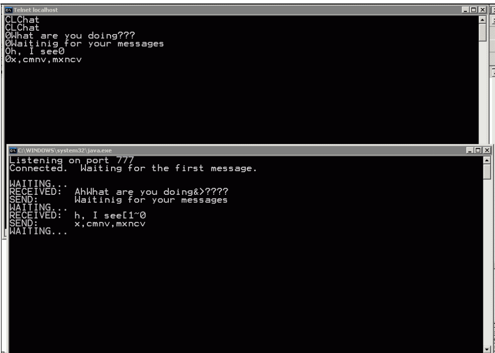
Рис. 2.9. Сервер (листинг 2.11) и клиент telnet на порте 777
