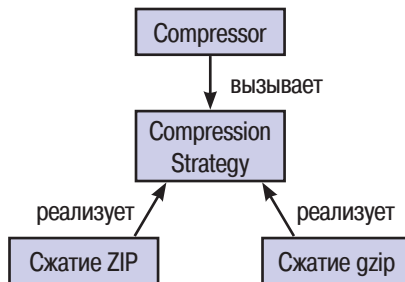
Рис. 8.2 ❖ Паттерн Стратегия
