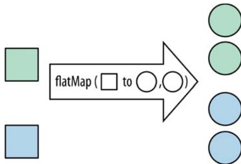
Рис. 3.7 ❖ Операция flatMap
