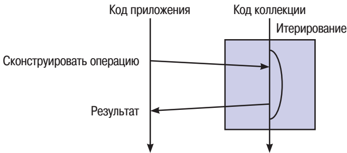
Рис. 3.2 ❖ Внутреннее итерирование
