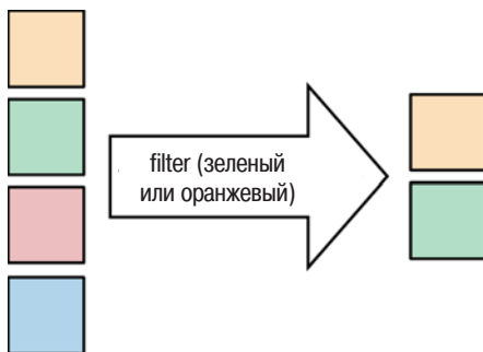
Рис. 3.5 ❖ Операция filter
