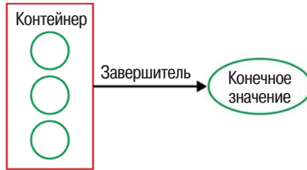
Рис. 5.6 ❖ Завершитель
