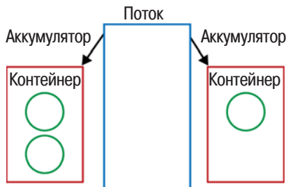
Рис. 5.4 ❖ Аккумулятор
