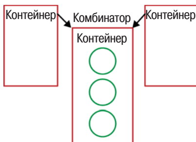
Рис. 5.5 ❖ Комбинатор
