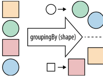
Рис. 5.2 ❖ Коллектор groupingBy
