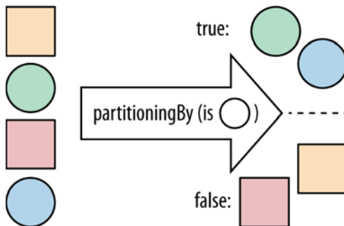
Рис. 5.1 ❖ Коллектор partitioningBy
