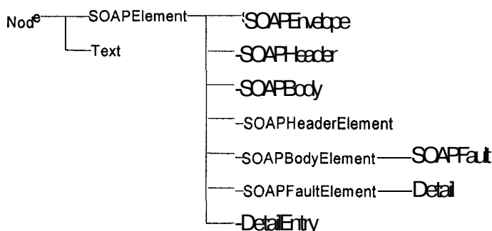
Рис. 6.1. Иерархия интерфейсов SAAJ
