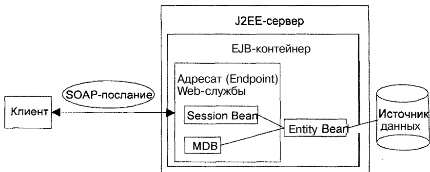
Рис 7.2. Реализация Web-службы компонентами EJB
