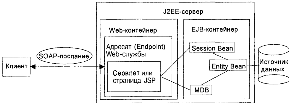
Рис 7.1. Компоненты EJB в составе Web-службы
