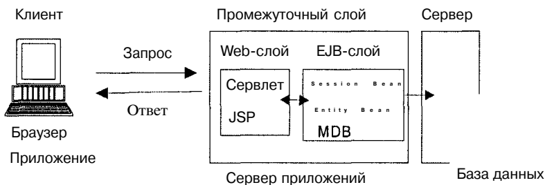
Рис. 2.2. Многослойная архитектура
