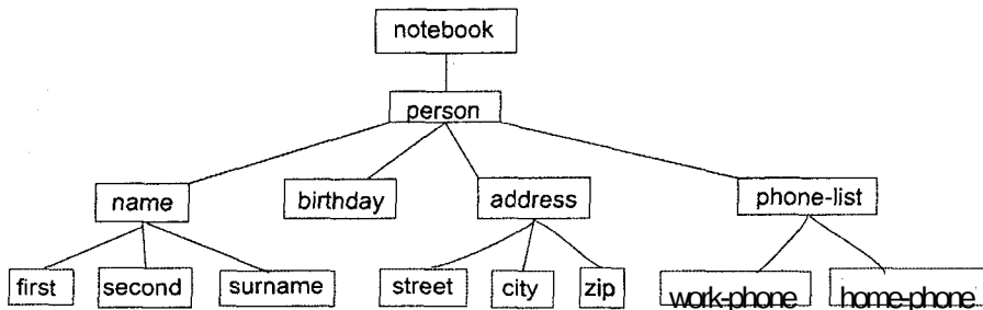
Рис. 1.1. Дерево элементов документа XML
