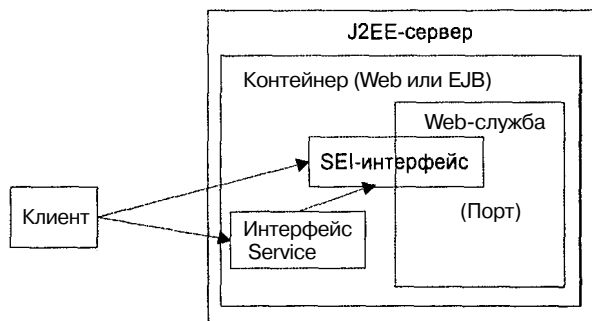
Рис. 7.3. Схема, предлагаемая спецификацией "WS for J2EE"
