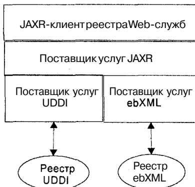
Рис. 2.4. Обращение к реестру Web-служб
