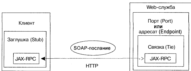
Рис. 6.2. Механизм JAX-RPC
