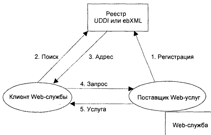
Рис. 2.3. Взаимодействие клиента Web-службы с ее поставщиком
