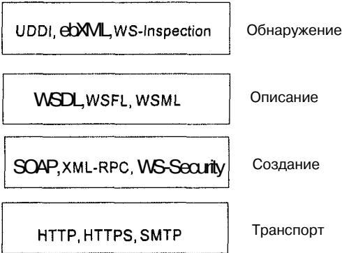
Рис. 2.5. Стек протоколов Web Services
