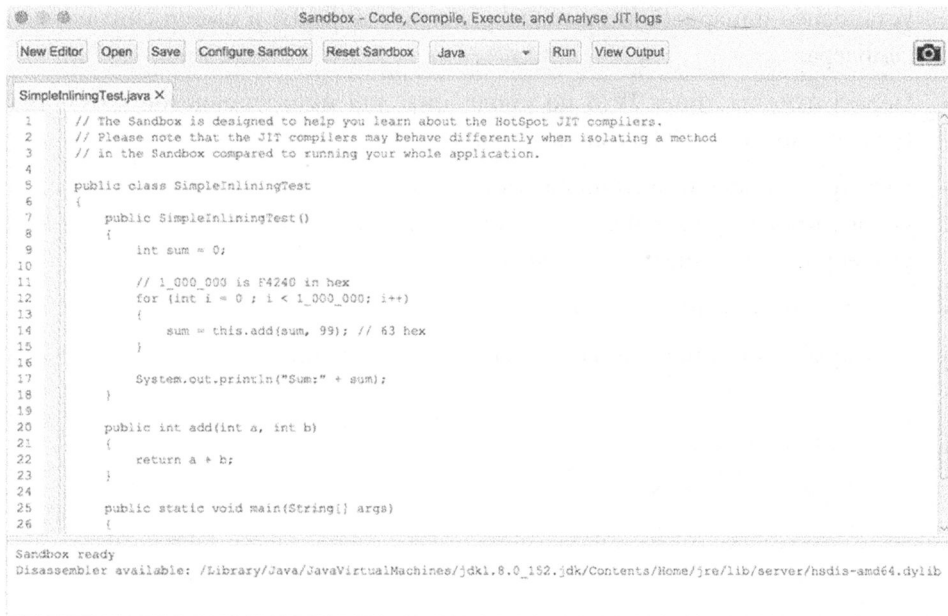
Рис. 10.2. Песочница JITWatch
