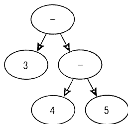
Рис. 19.1. Неправильный порядок группировки выражений
