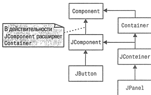
Рис. 10.4. Более удачная иерархия контейнеров Swing
