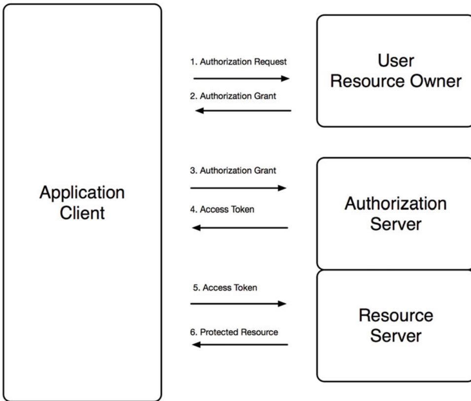
Figure 9-7. OAuth flow
