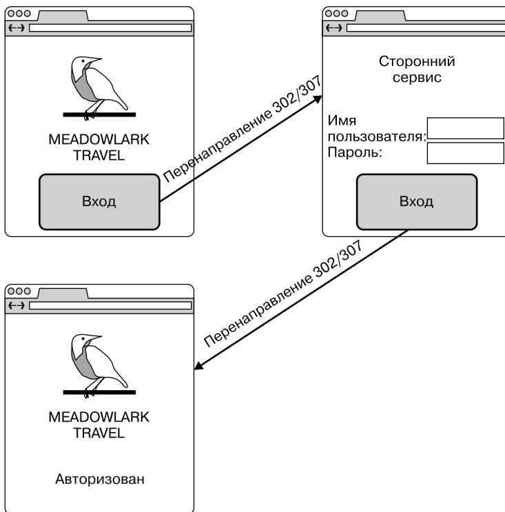
Рис. 18.1. Процесс сторонней аутентификации
