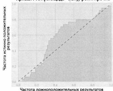
Кривая РХП (площадь=0.57)/рок и прочие
