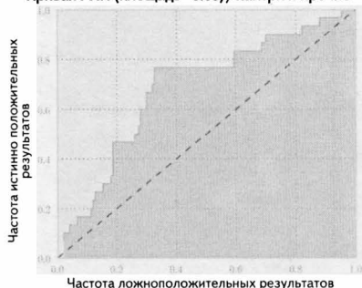
Кривая РХП (площадь=0.57)/рок и прочие
