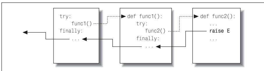
Рис. 35.2. Вложенные инструкции try/finally : когда возбуждается исключение, управление возвращается самой последней инструкции try и выполняется ее блок finally , после этого исключение продолжит свое движение по блокам finally во всех активных инструкциях try , пока в конечном счете не будет достигнут обработчик по умолчанию, где производится вывод сообщения об ошибке. Предложения finally перехватывают (но не останавливают) исключения – они определяют действия, которые должны выполняться «на выходе»
