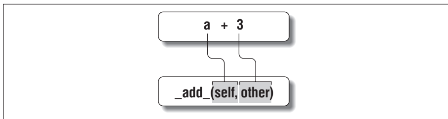
Рис. 26.3. Механизм перегрузки отображает операторы выражений и другие встроенные операции, выполняемые над экземплярами классов, на специальные имена методов в классе. Эти специальные методы являются необязательными и могут наследоваться, как обычные методы. Здесь использование оператора «+» приводит к вызову метода __add__
