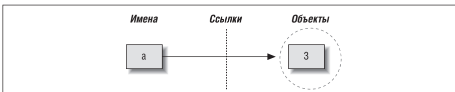
Рис. 6.1. Имена и объекты после выполнения операции присваивания a = 3 . Переменная превращается в ссылку на объект 3. Во внутреннем представлении переменная в действительности является указателем на пространство памяти с объектом, созданным в результате интерпретации литерального выражения 3
