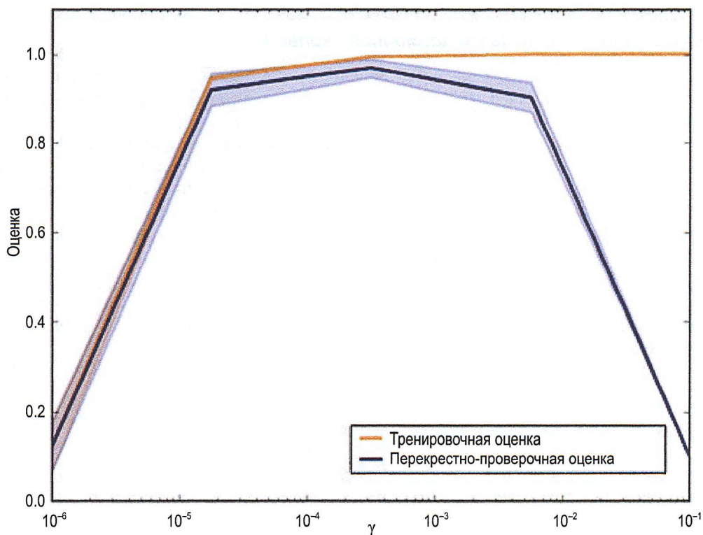
Проверочная кривая модели SVM
