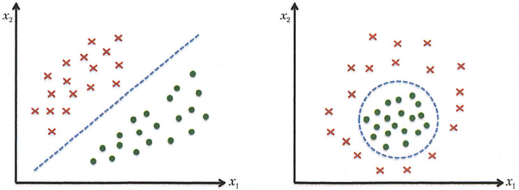
Линейные задачи в сопоставлении с нелинейными
