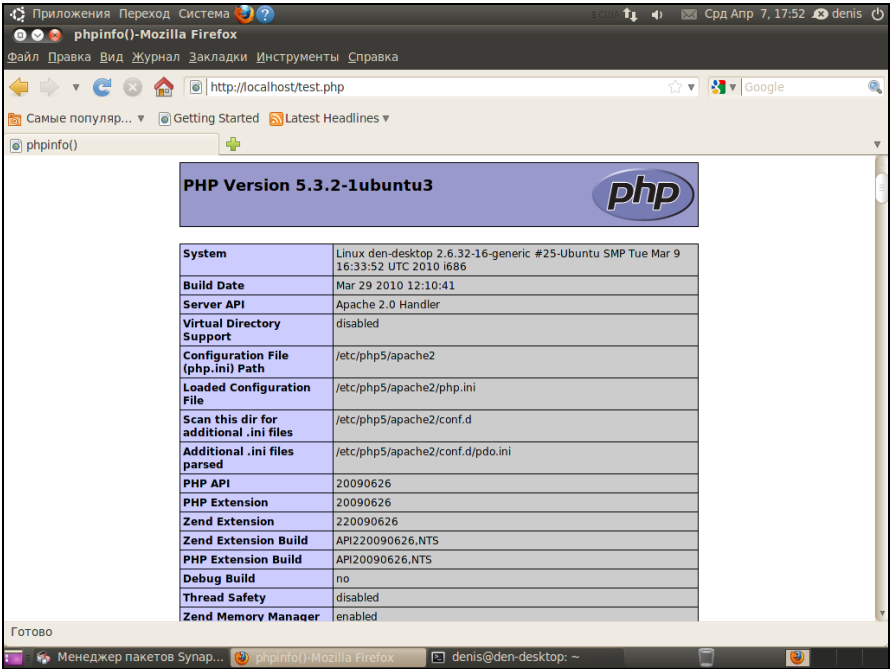
Рис. 18.3. Тестовый сценарий
