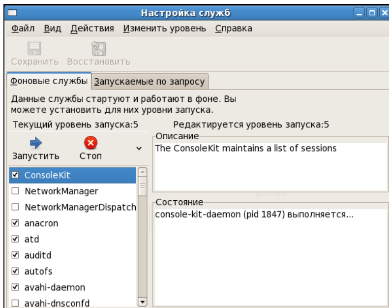
Рис. 11.1. Конфигуратор system-config-services
