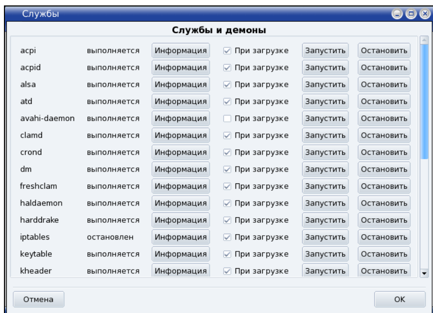
Рис. 11.4. Конфигуратор drakxservices
