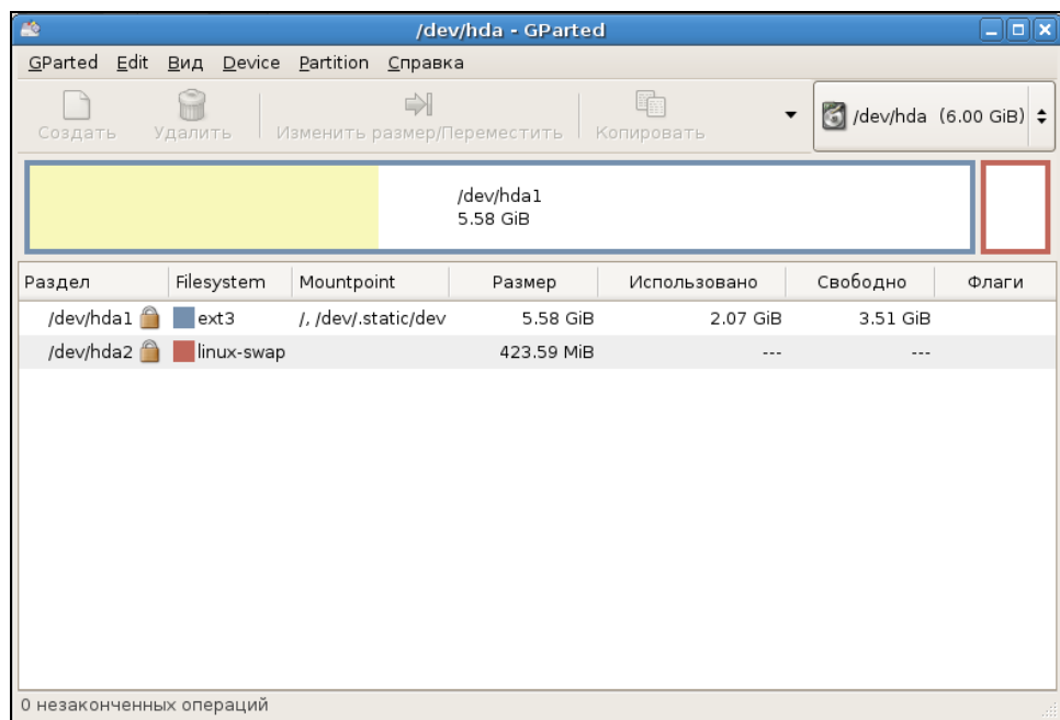
Рис. 9.9. Программа GParted
