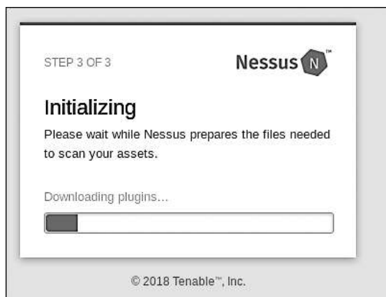
Рис. 6.6. Инициализация Nessus
