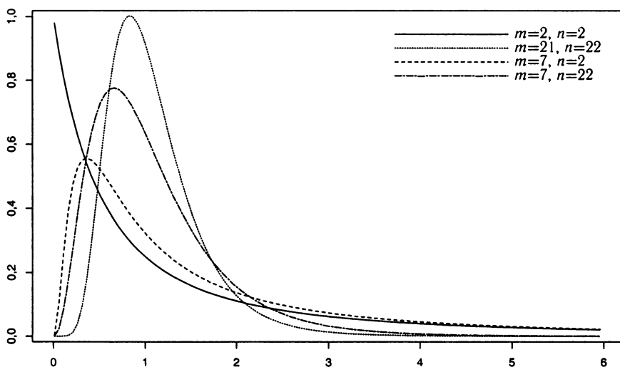
Рис. 1.3. Плотности распределения Фишера при m = 2, n = 2 ; m = 7, n = 2 ; m = 21, n = 22 ; m = 7, n = 22
