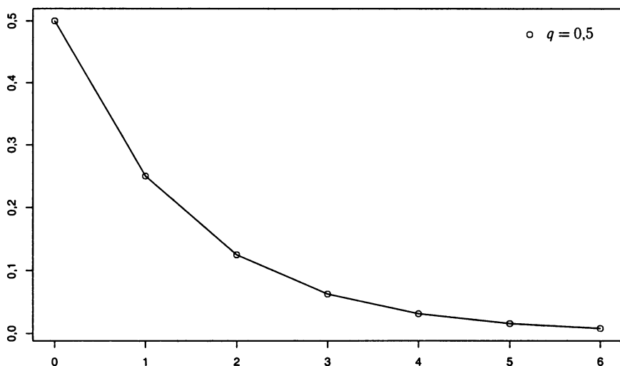
Рис. 1.4. Геометрическое распределение
