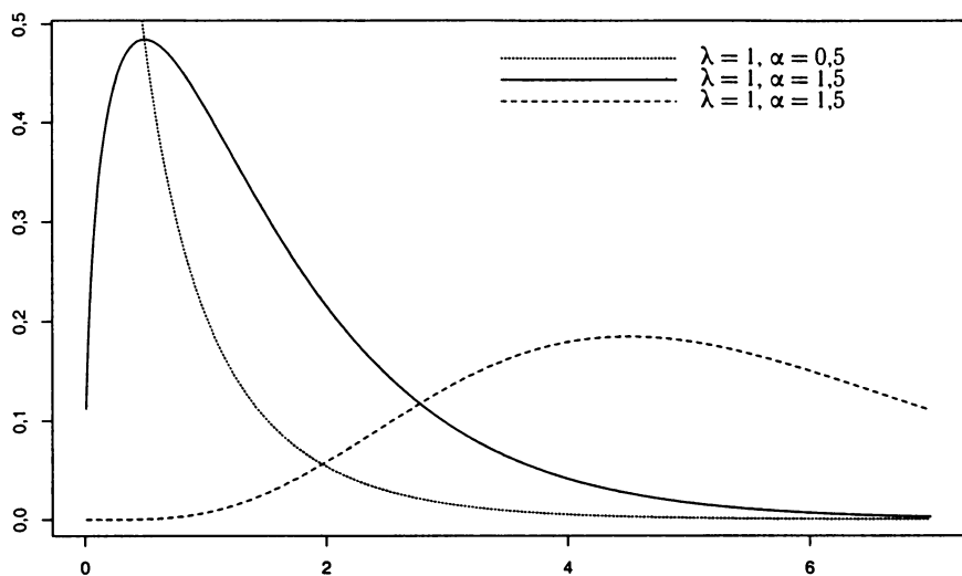
Рис. 2.7. Плотности гамма-распределения
