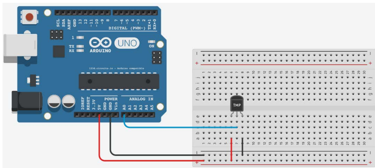
Рис. 6.4: Пример подключения аналогового датчика температуры
