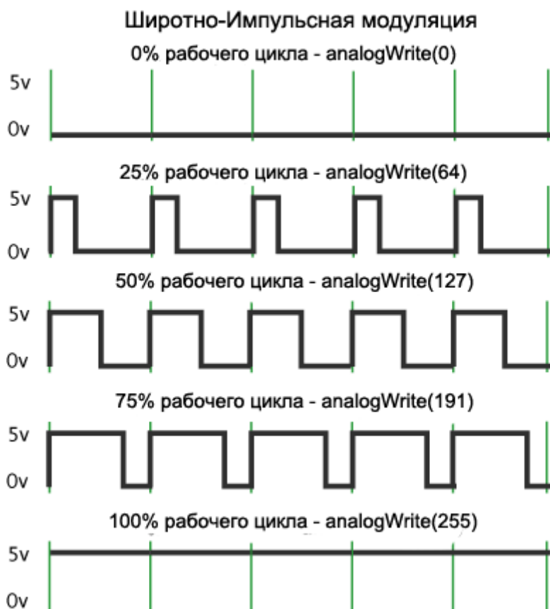
Рис. 7.1: Сигналы широтно-импульсной модуляции
