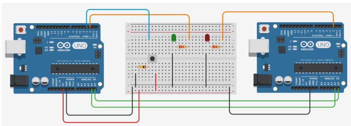
Рис. 8.2: Пример подключения шины i 2 C
