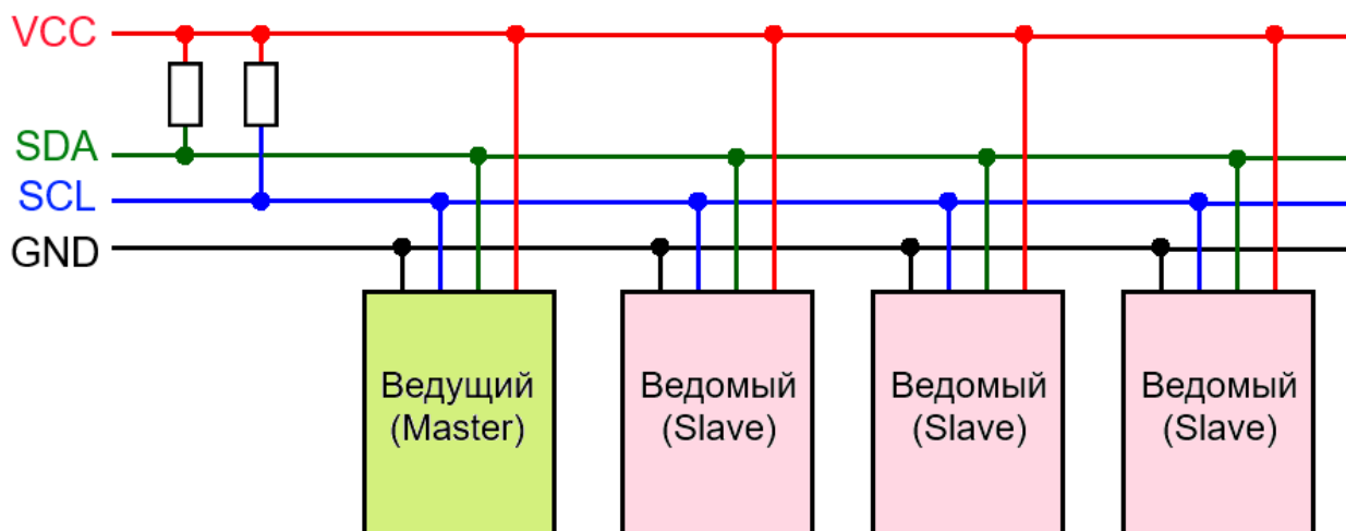
Рис. 8.1: Шина I 2 C
