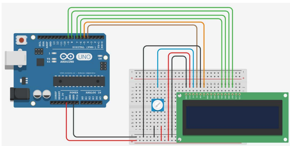
Рис. 5.4: Пример подключения дисплея к общей схеме
