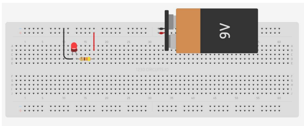
Рис. 3.8: Работа светодиода
