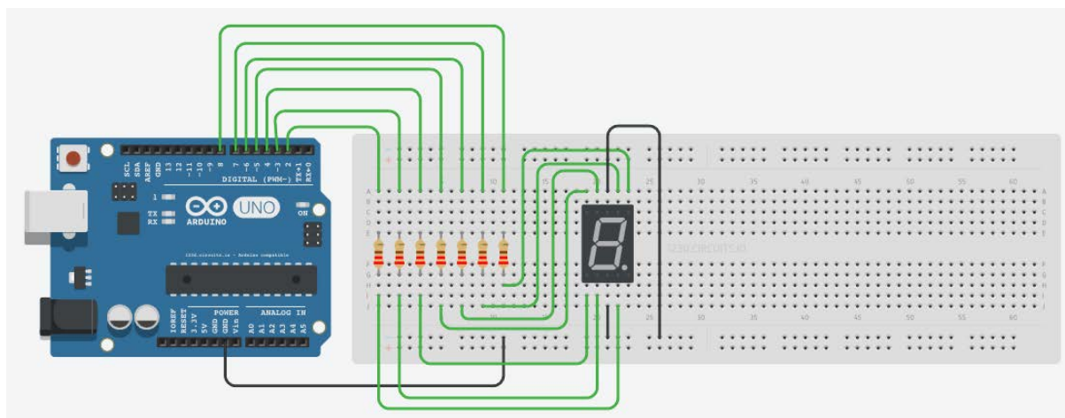
Рис. 5.2: Пример подключения семисегментного индикатора
