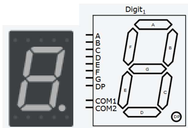
Рис. 5.1: Сегментный индикатор
