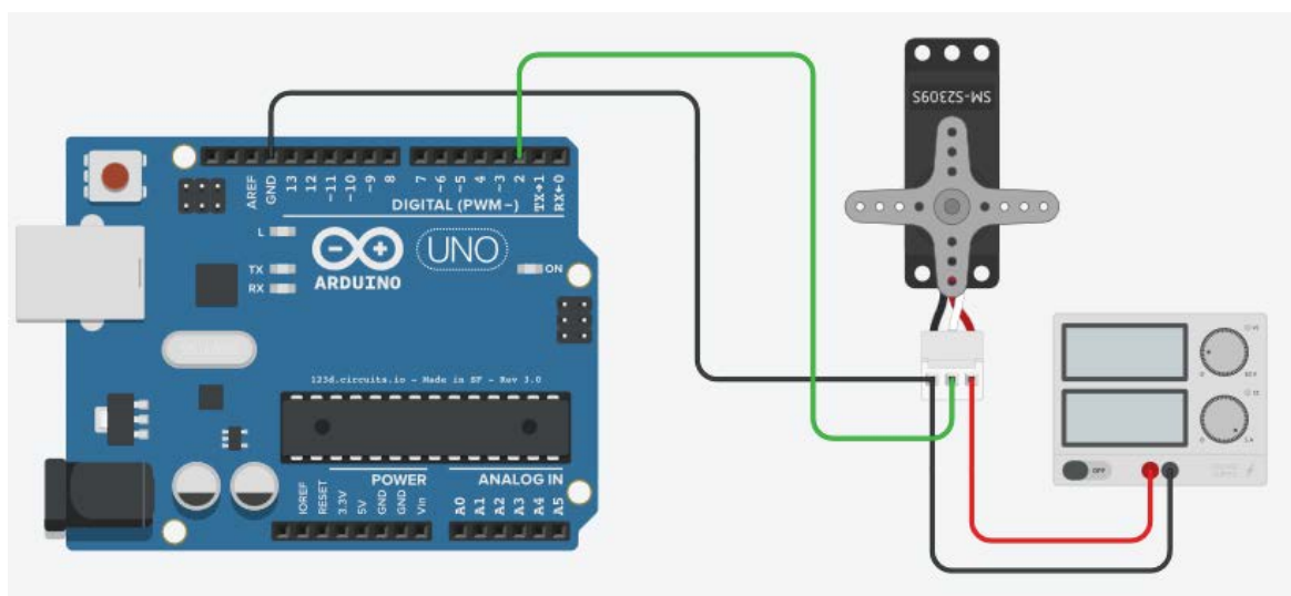
Рис. 7.5: Пример подключения серводвигателя
