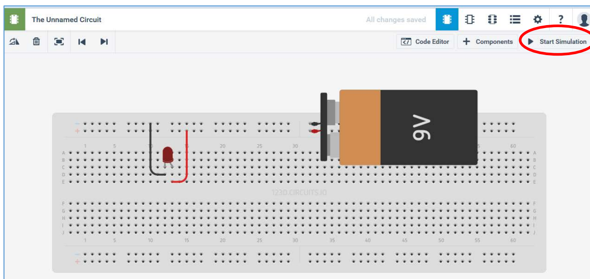
Рис. 3.7: Пример подключения светодиода
