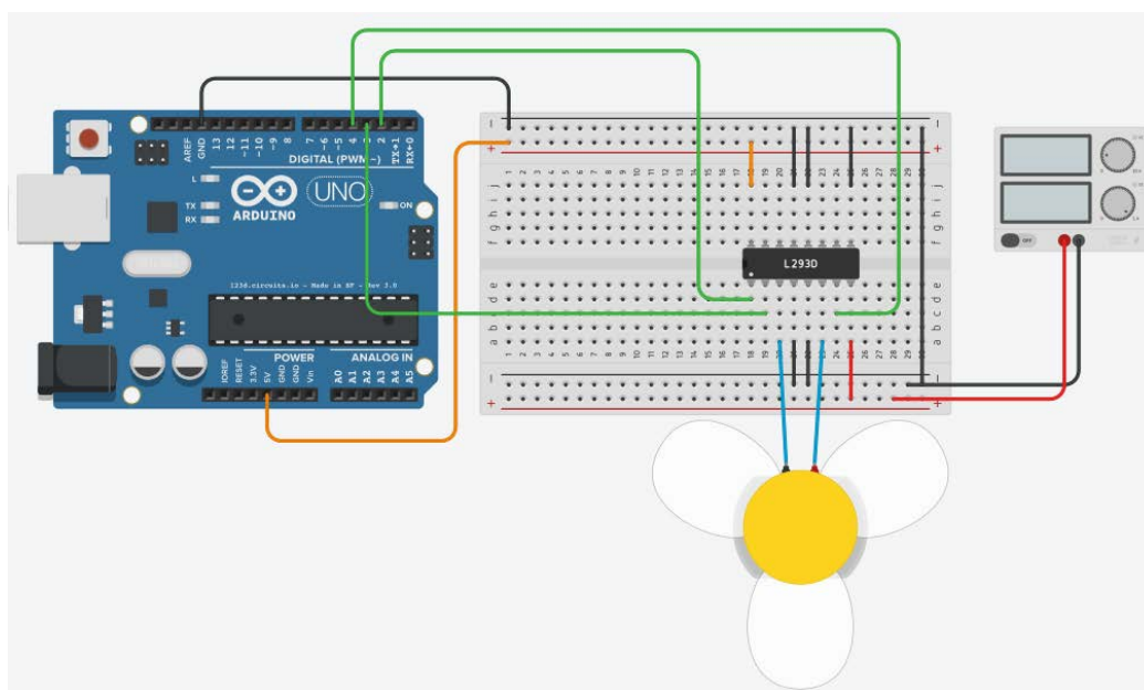
Рис. 7.3: Пример подключения микросхемы L293D
