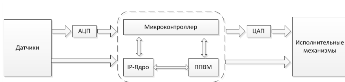
Рис. 1.1: Устройство встроенных систем
