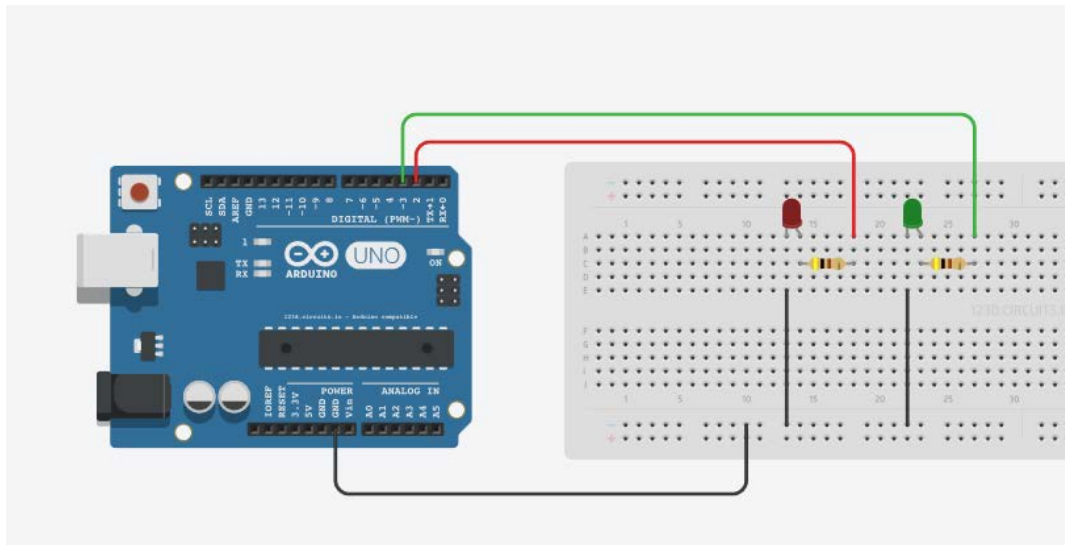
Рис. 4.3: Схема подключения двух светодиодов
