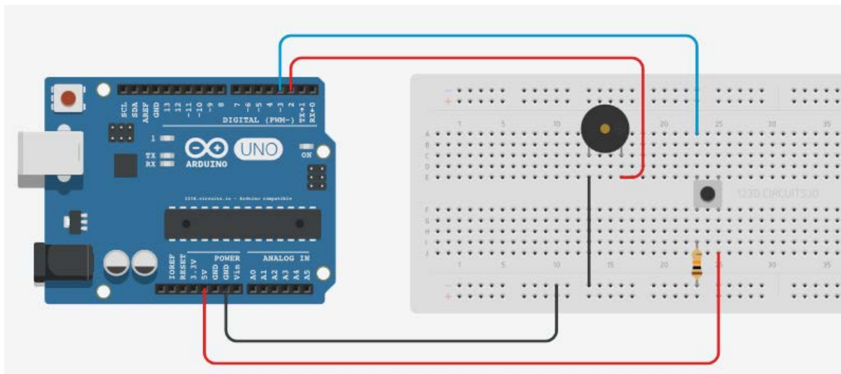
Рис. 4.5: Пример подключения резистора
