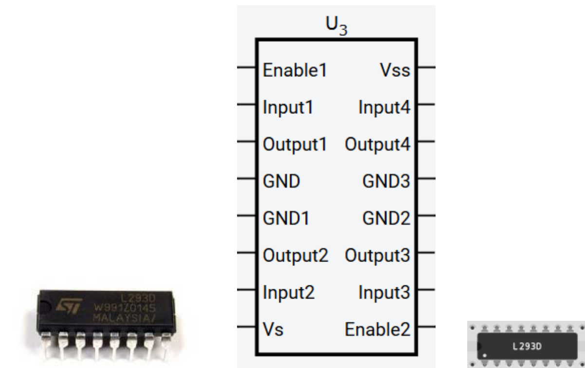
Рис. 7.2: Микросхема L293D
