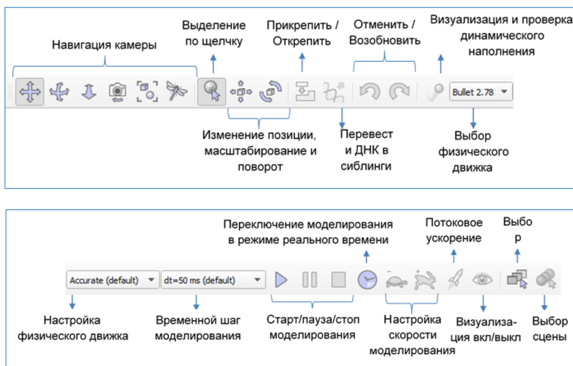
Рис. 9.2: Меню программы V-REP
