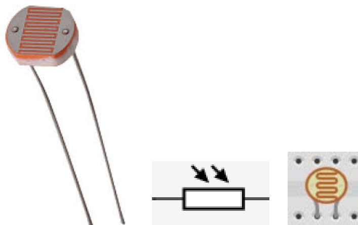
Рис. 6.5: Фоторезистор
