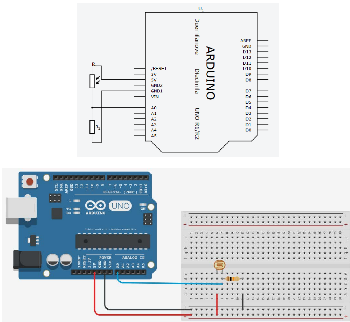
Рис. 6.6: Пример подключения фоторезистора
