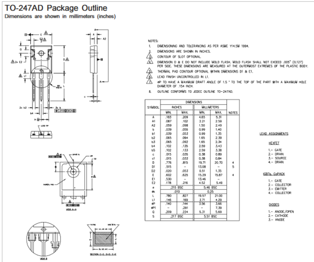
Рис. 2.4: Чертеж транзистора
