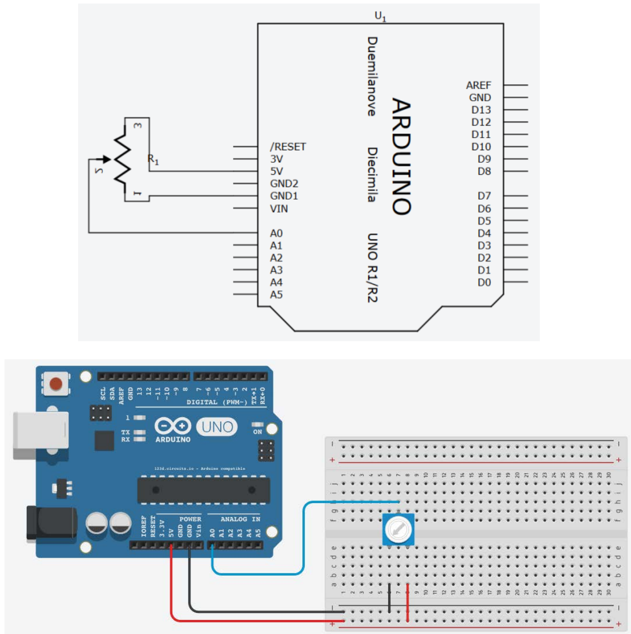
Рис. 6.2: Пример подключения реостата
